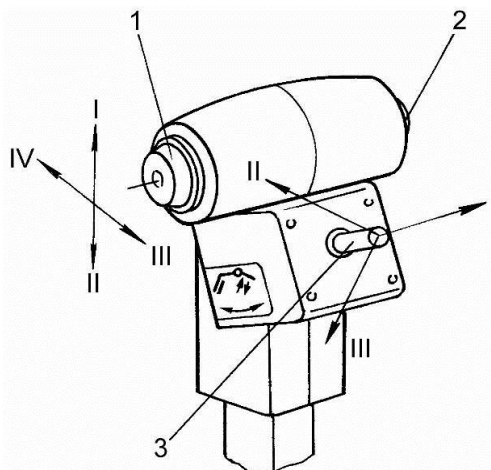
Рисунок 1.30 – Рукоятка управления скоростью движения
