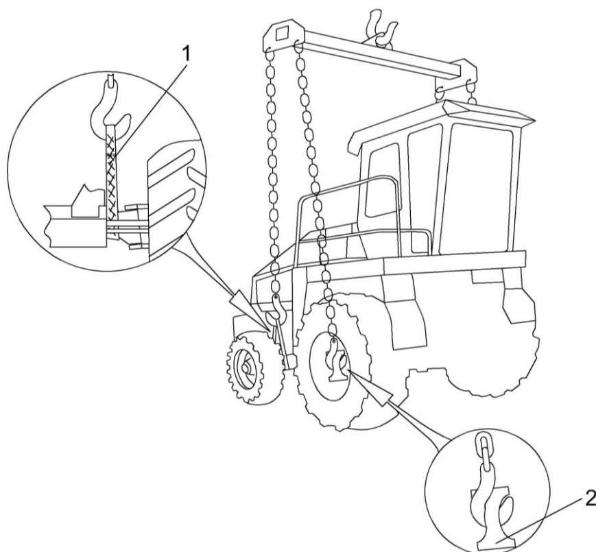
Рисунок 5.1 – Схема строповки
