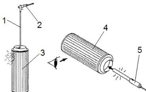
Рисунок 3.2 – Обслуживание основного фильтрующего элемента
