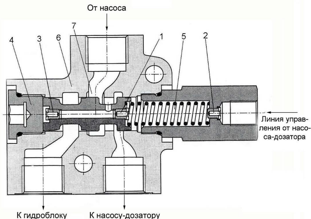
Рисунок 1.21 – Приоритетный клапан
