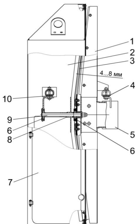
1 – пылесъемник; 2 – диффузор; 3 – сетка; 4, 10 – опоры; 5 – патрубок; 6 – втулка; 7 – дверь; 8 – прокладка; 9 – ось
