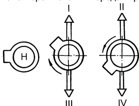
Рисунок 1.25 – Схема переключения передач при движении машины лесохозяйственной кабиной вперед
