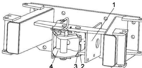
Рисунок 1.8 – Сцепное устройство
