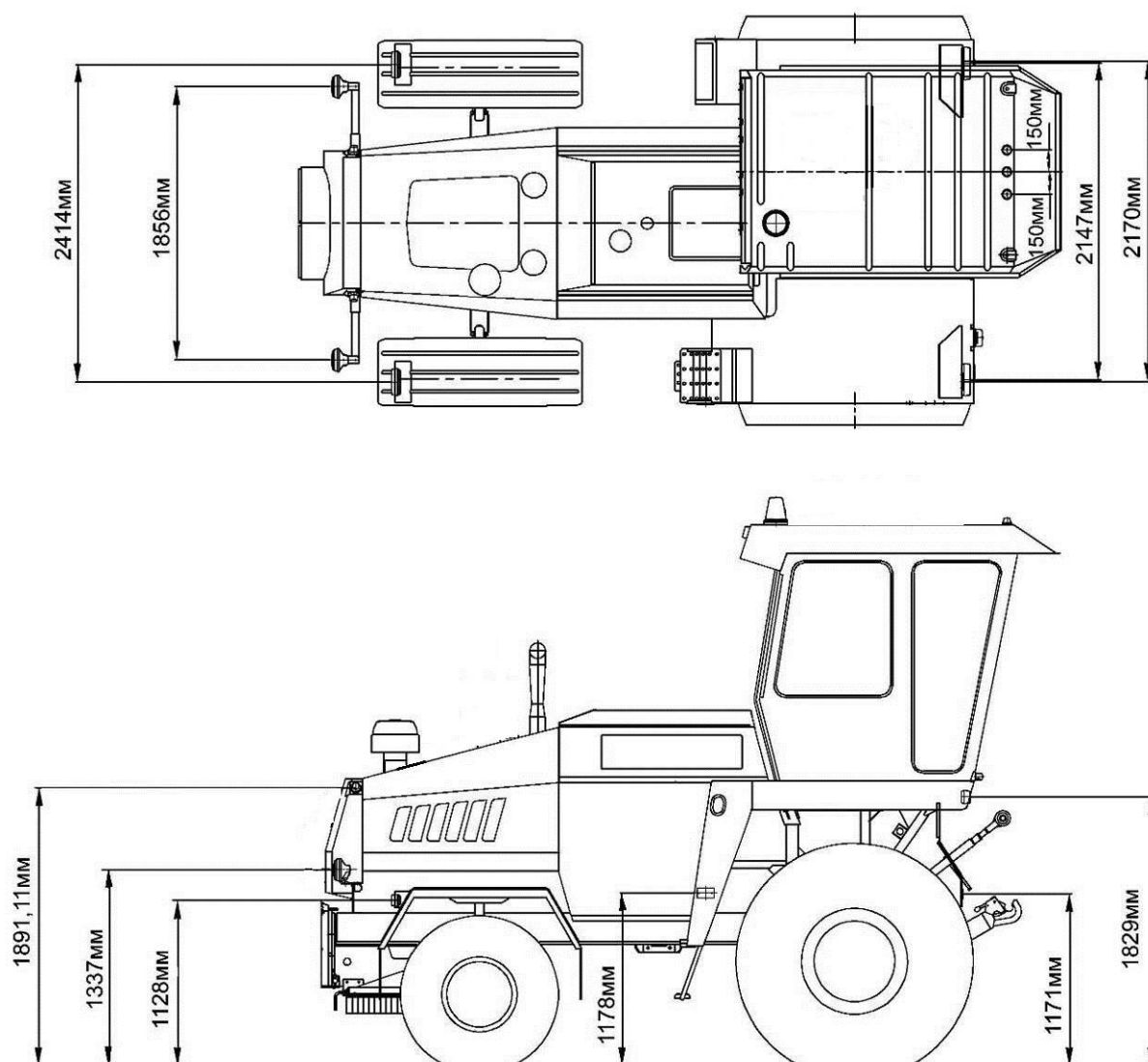
Рисунок 1.23 – Схема расположения элементов наружного освещения и световой сигнализации машины лесохозяйственной
