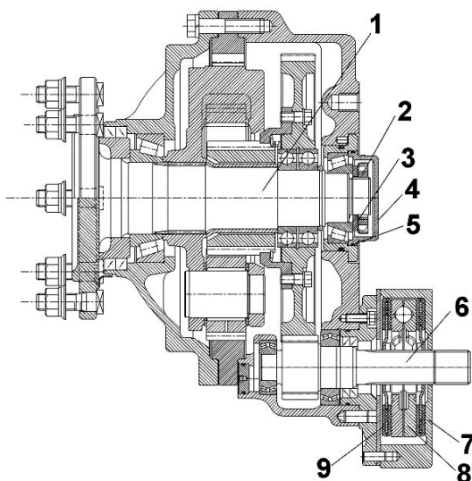
1 – ось колеса; 2 – гайка; 3 – шайба; 4 – крышка; 5 – кольцо резиновое; 6 – ведущий вал; 7 – корпус тормоза; 8 – нажимной диск; 9 – фрикционный диск
