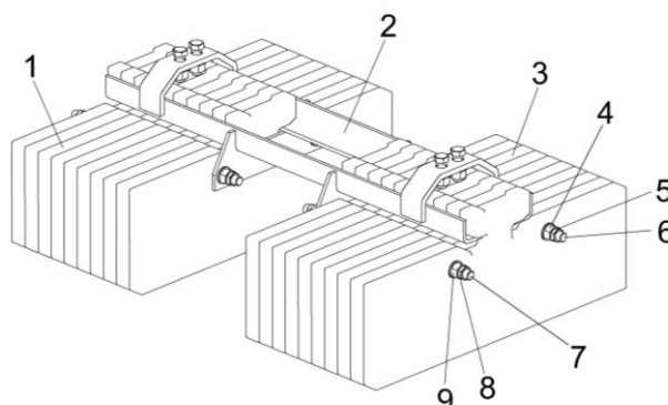
Рисунок 1.9 - Установка противовесов
