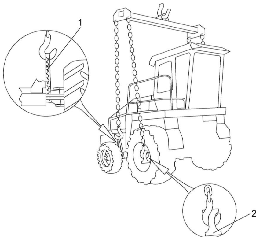
Рисунок 5.1 – Схема строповки
