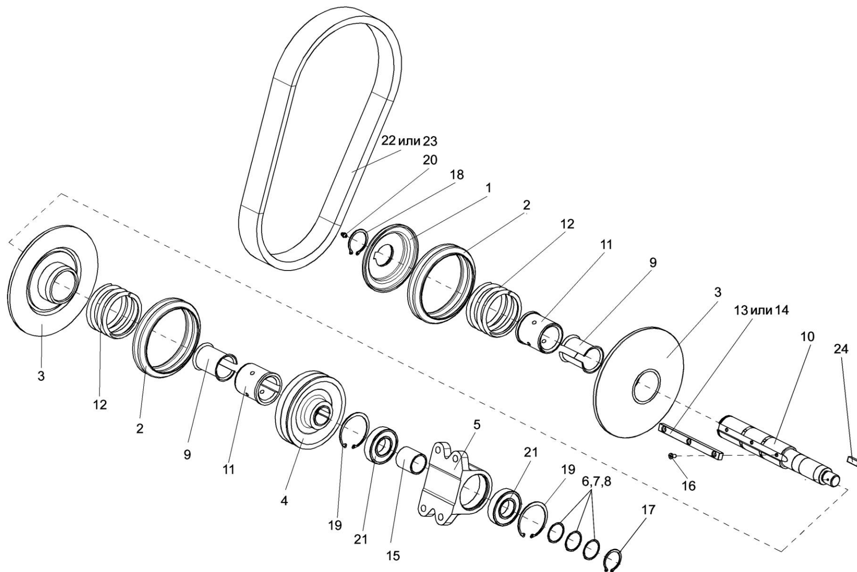
Рисунок 14 – Вариатор КЗР 1514100А
