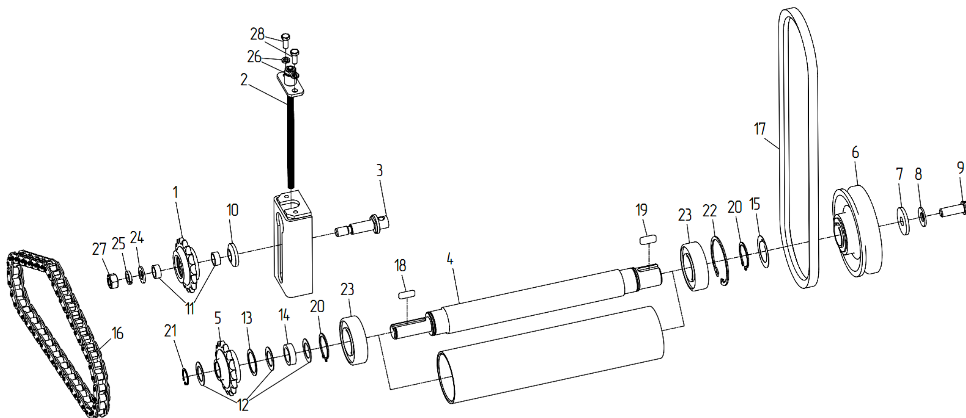
Рисунок 16 – Вал промежуточный привода вариатора
