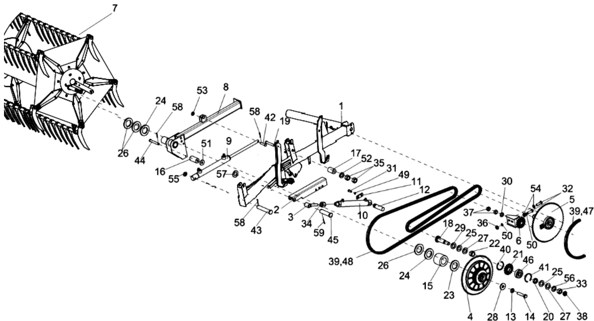
Рисунок 5 – Установка мотовила (вид слева)
