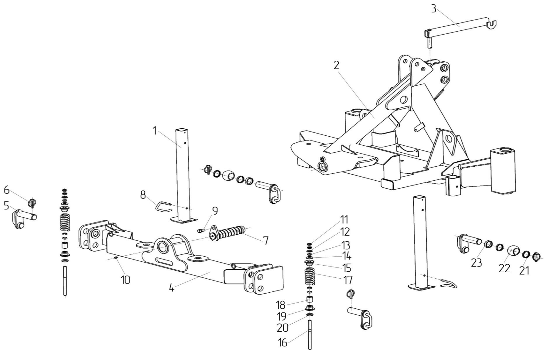
Рисунок 20 – Проставка ЖВЗ 7060000-01
