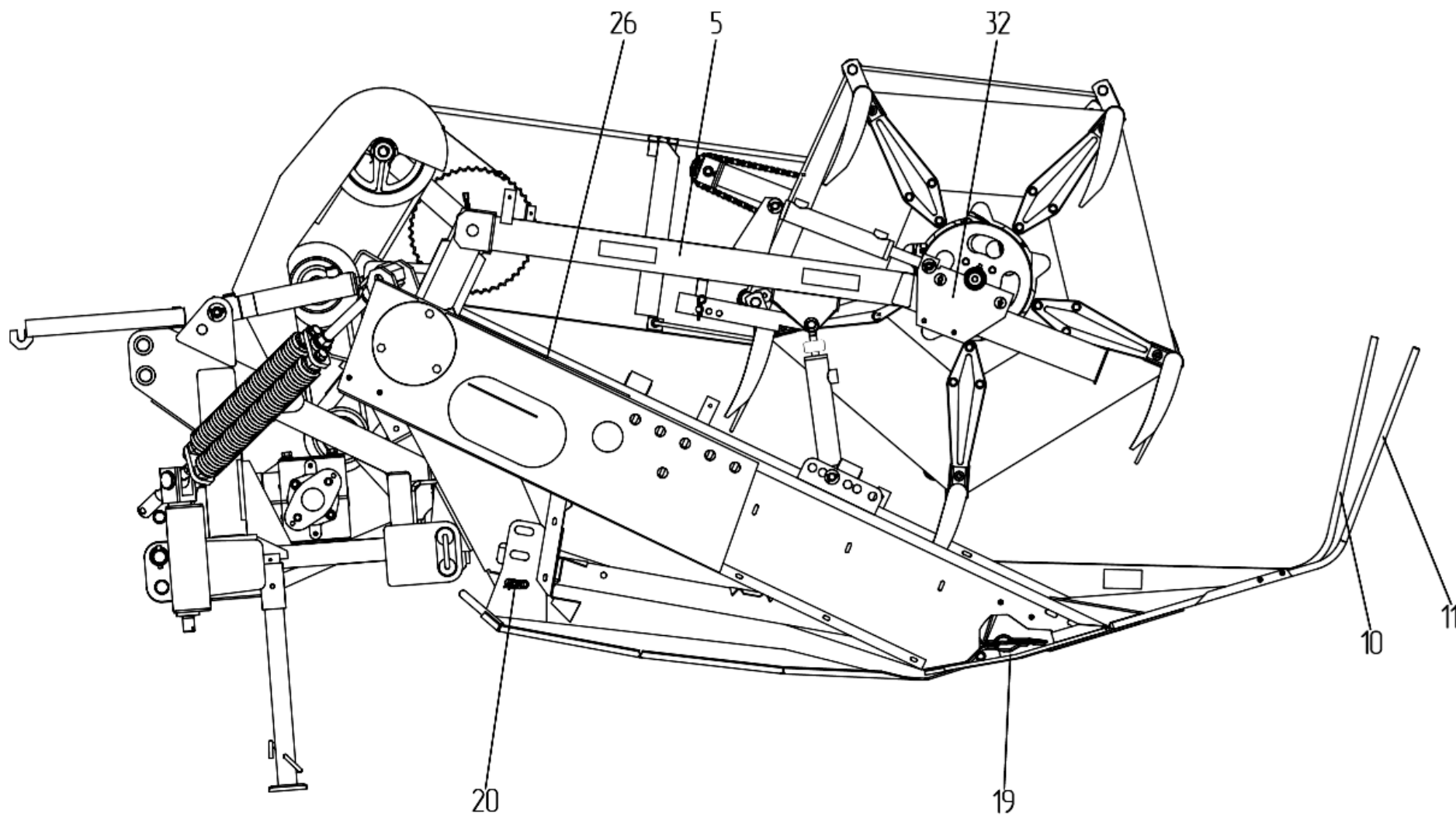
Рисунок 1в – Жатка валковая ЖВЗ-7УМ (ЖВЗ-7-1000000Э)
