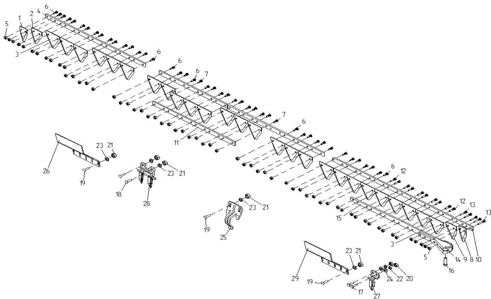
Рисунок 27 – Нож ЖВЗ 2260000 и детали режущего аппарата
