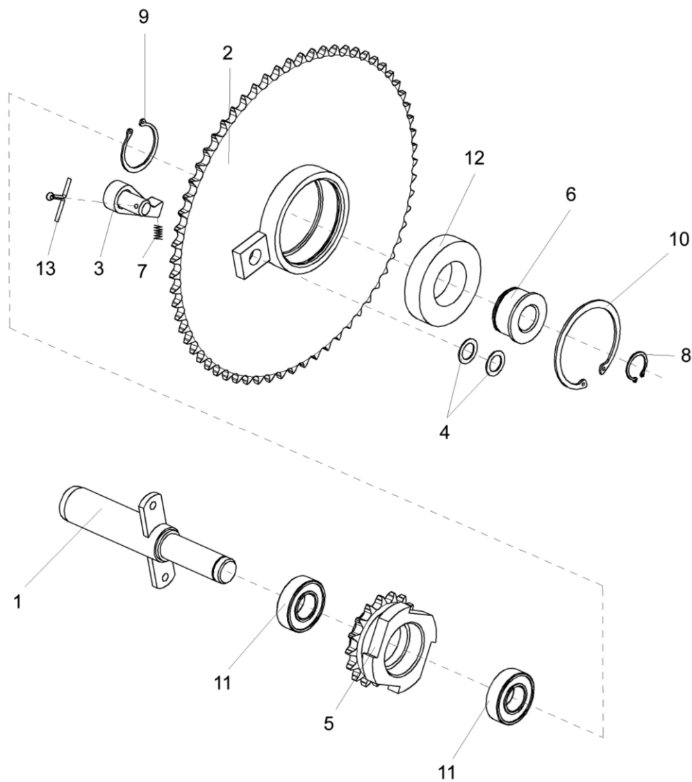
Рисунок 9 – Муфта обгонная КЗР 1504100
