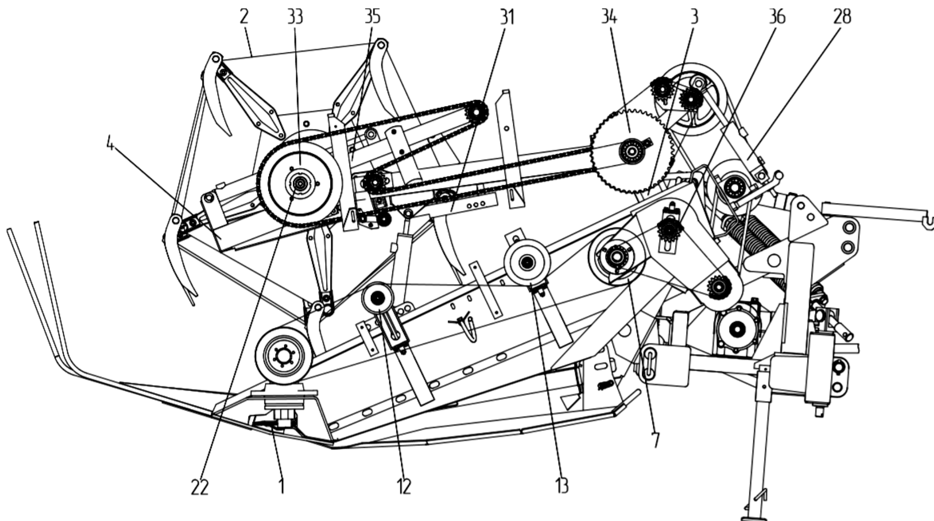
Рисунок 16 – Жатка валковая ЖВЗ-7УМ (ЖВЗ-7-1000000Э)
