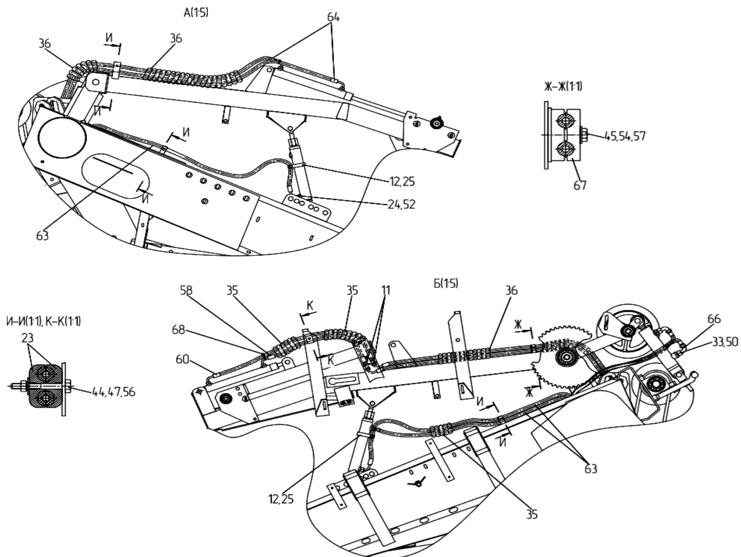
Рисунок 29 – Система гидравлическая ЖВЗ-7-1800000Э
