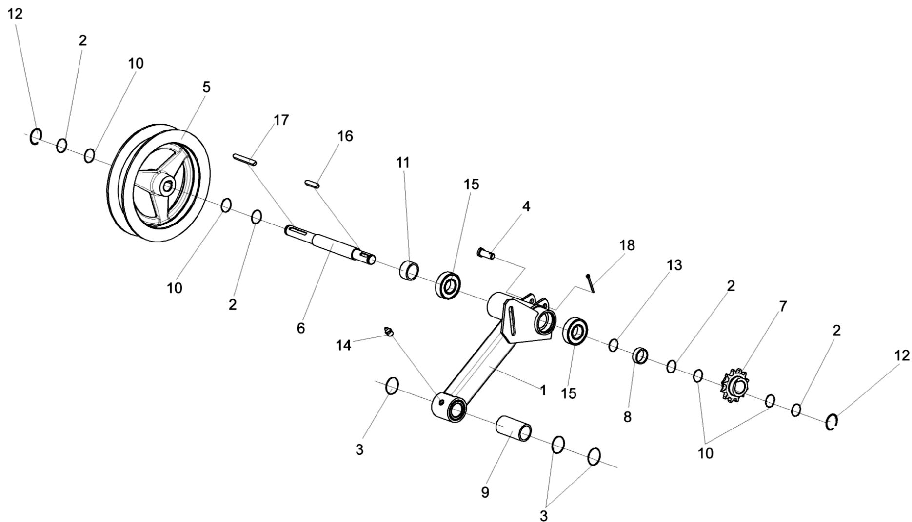
Рисунок 17 – Установка рычага ЖВЗ-7-1504200Э
