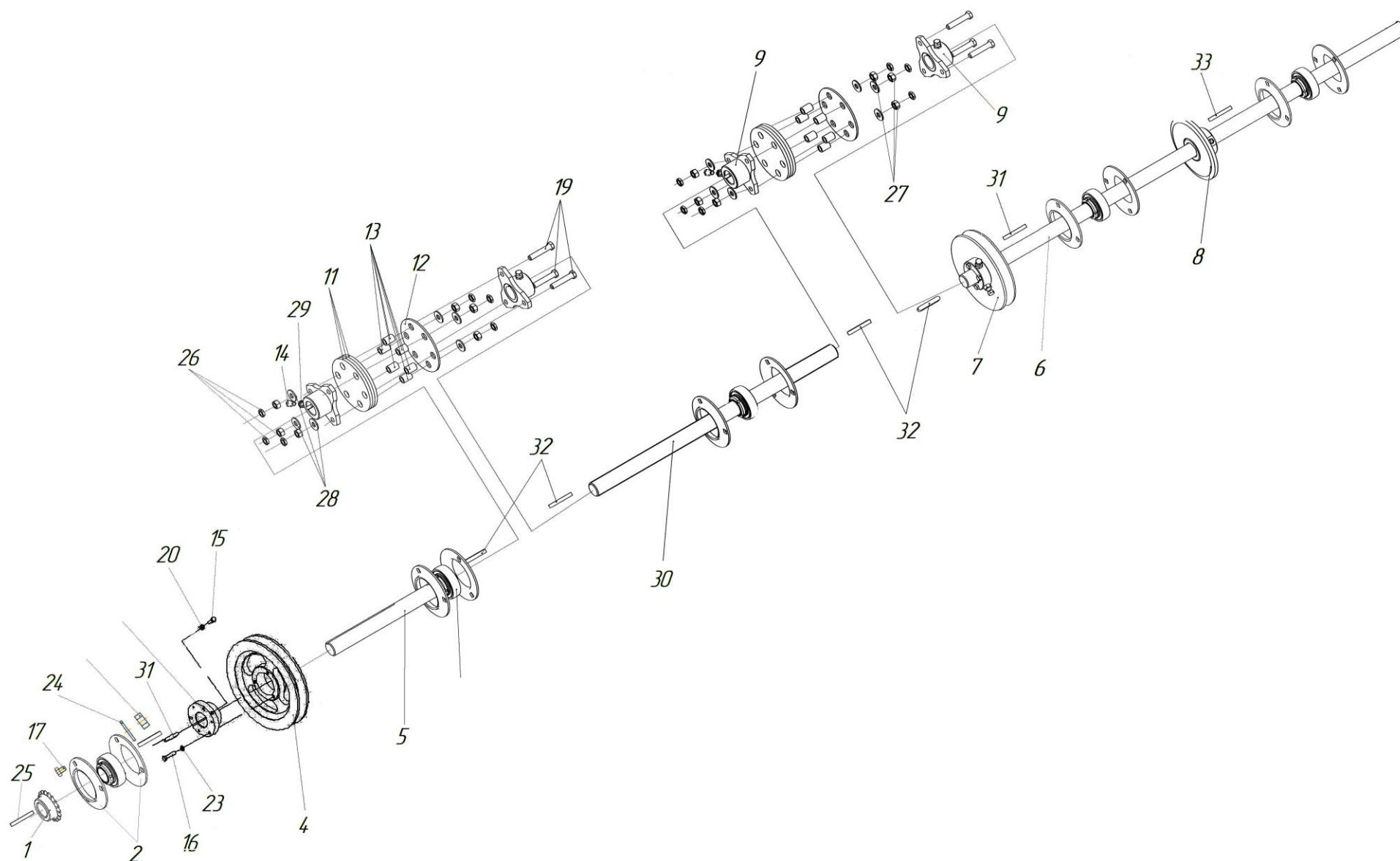
Рисунок 24 – Приводной вал в сборе
