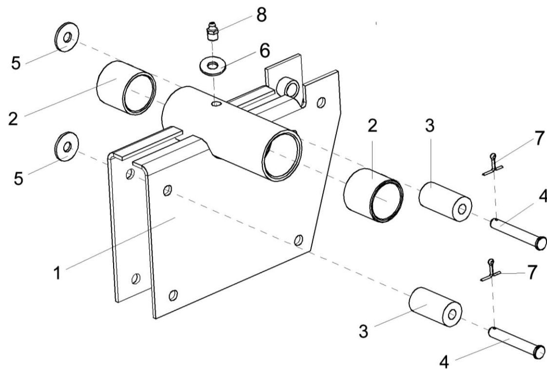
Рисунок 12 – Направляющая КЗК-12-1573100-01
