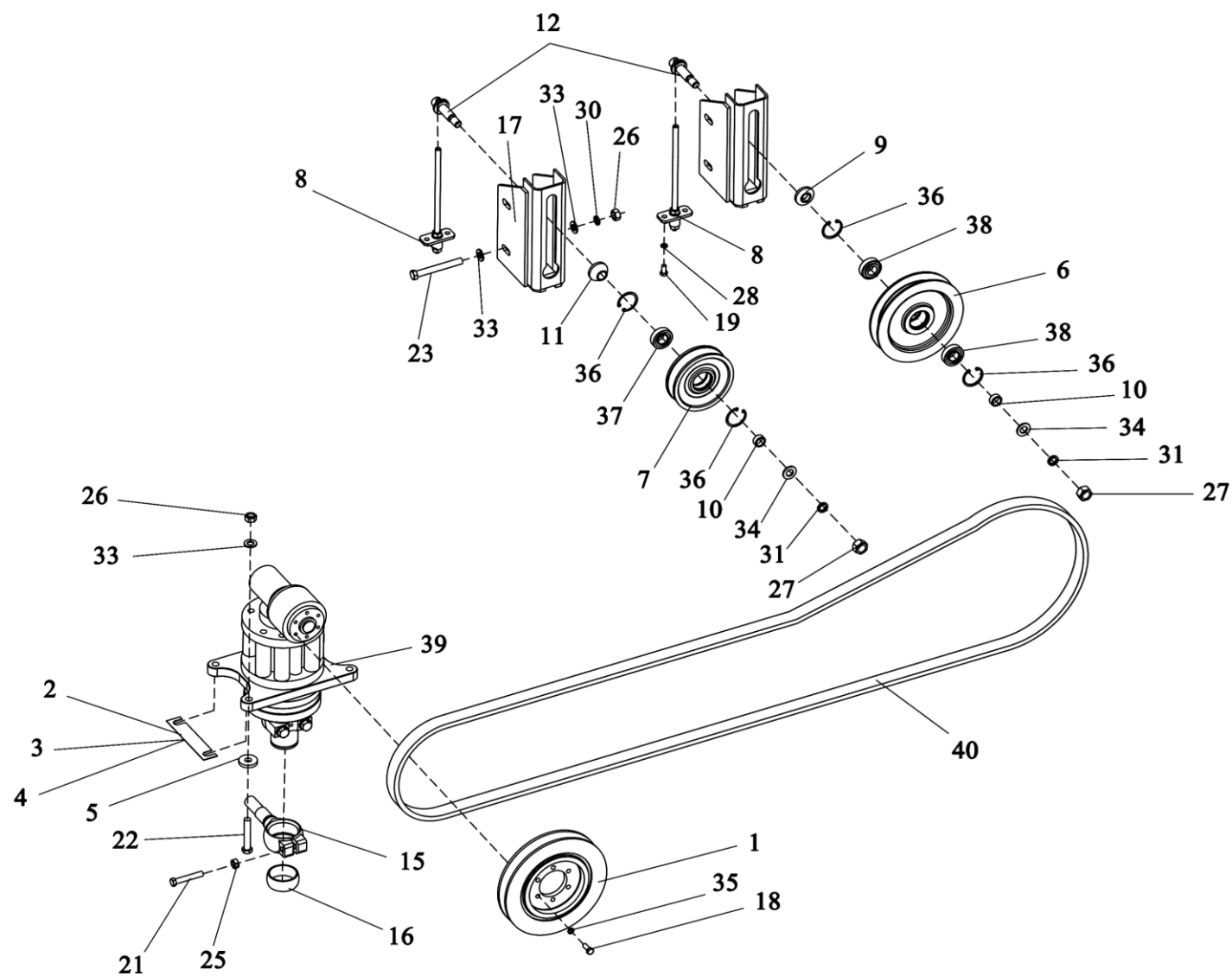
Рисунок 22 – Установка угловой передачи
