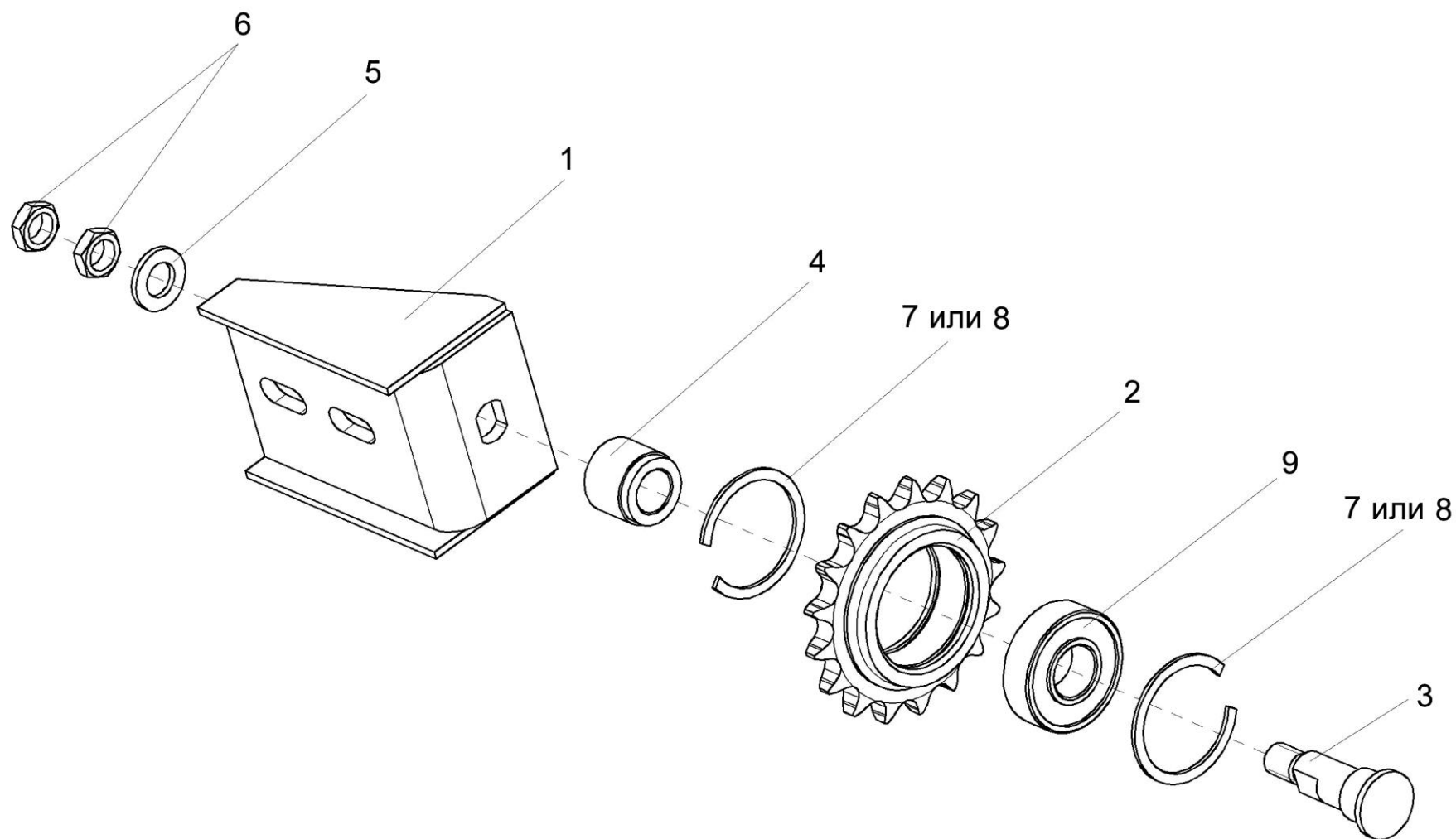
Рисунок 11 – Устройство обводное КЗР 1510000
