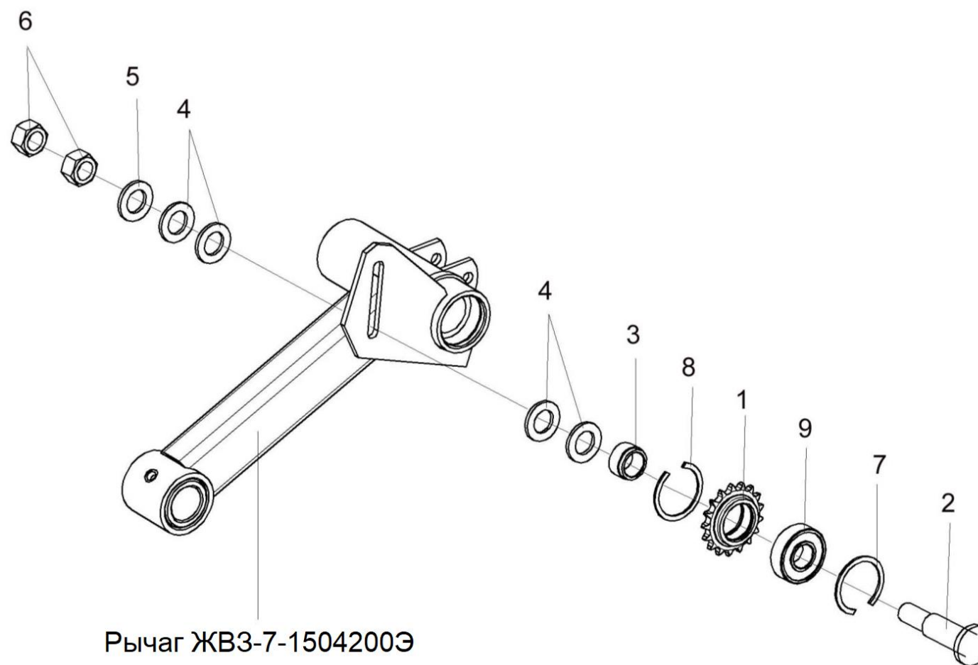
Рисунок 18 – Установка звездочки КЗР 1510020
