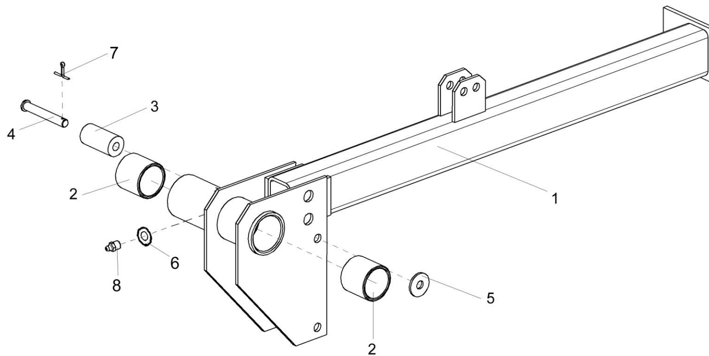
Рисунок 13 – Направляющая КЗР 1573080-01
