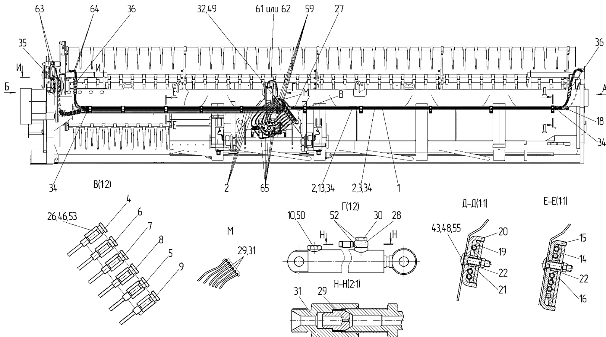
Рисунок 28 – Система гидравлическая ЖВЗ-7-1800000Э
