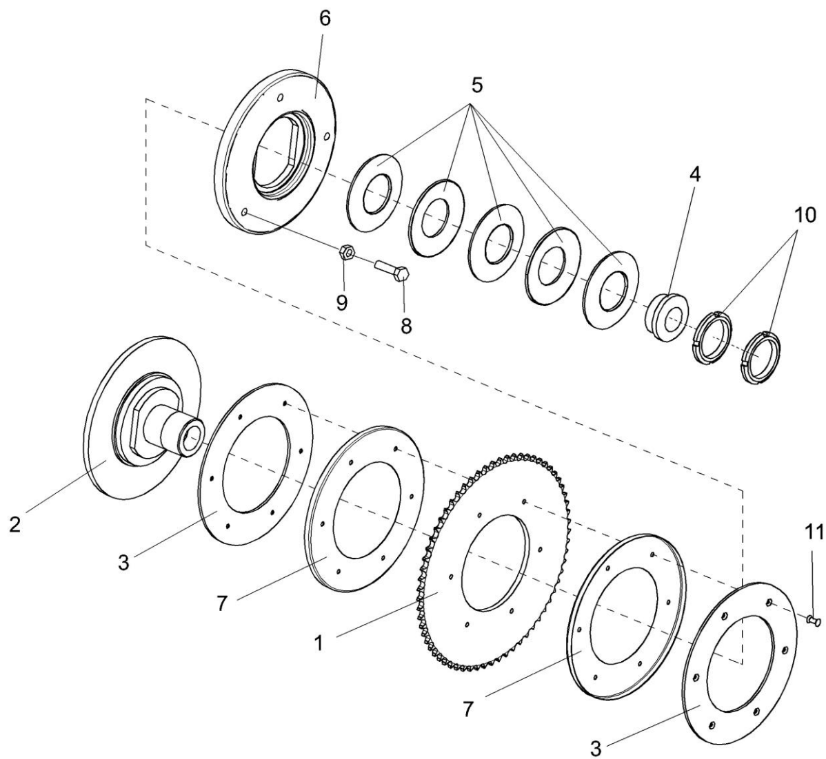
Рисунок 10 – Муфта фрикционная КЗР 1503140А
