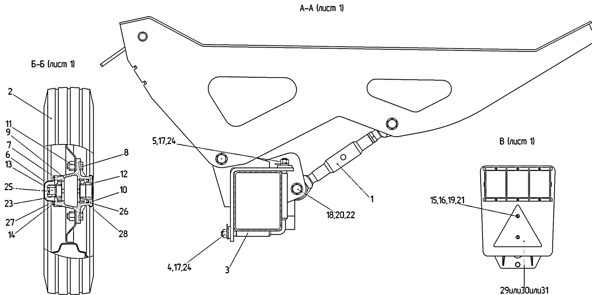
Рисунок 31 – Тележка транспортная ЖВЗ-7-1590010 (Лист 2)
