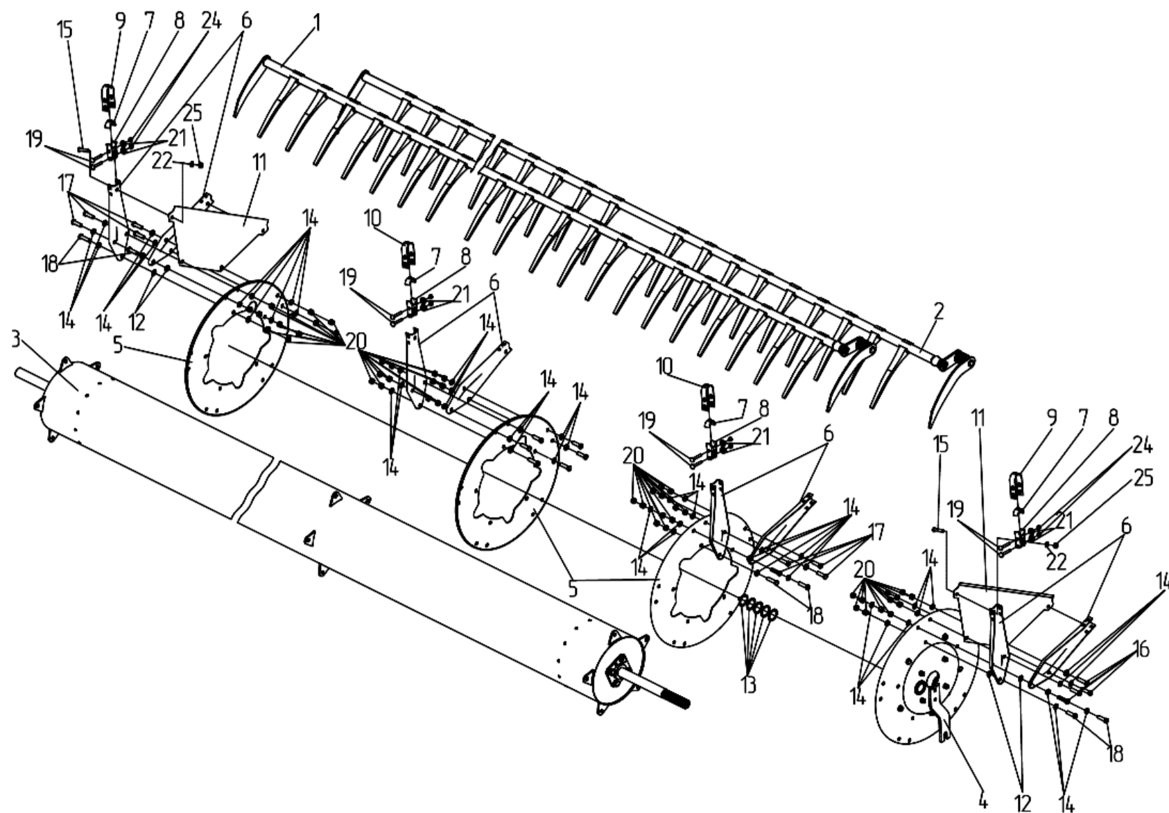
Рисунок 2 – Мотовило ЖВЗ-7-1503010Э
