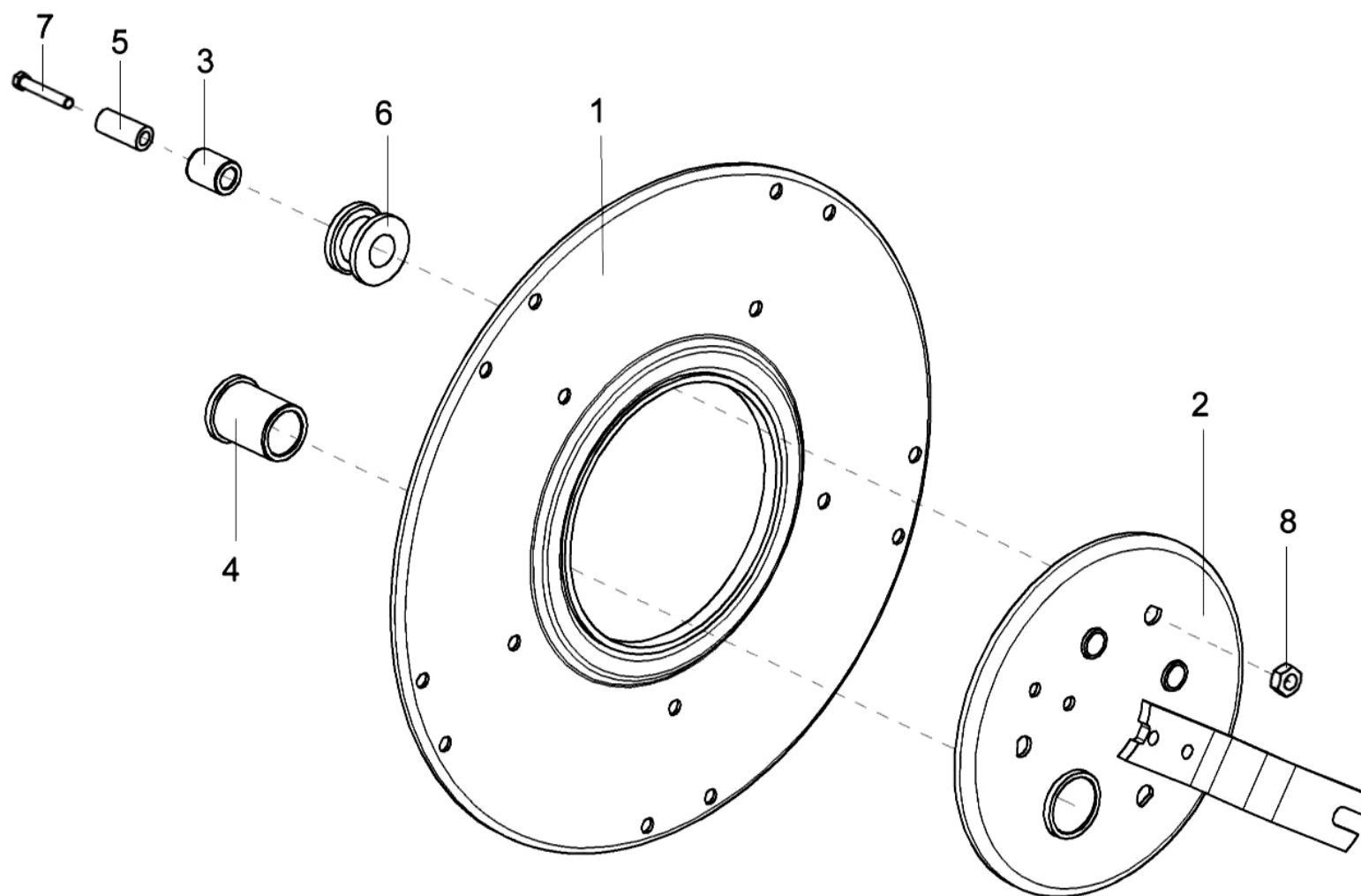
Рисунок 8 – Эксцентрик КЗК-12-1573170
