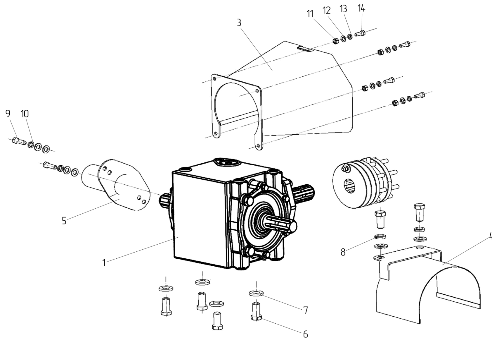
Рисунок 21 – Редуктор КПР 9303100
