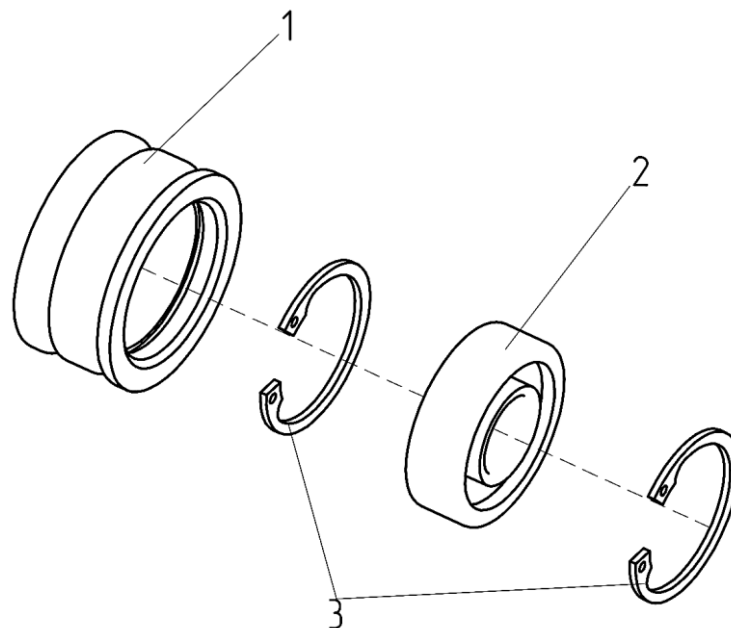
Рисунок 7 – Ролик ЖВЗ-7-1508180
