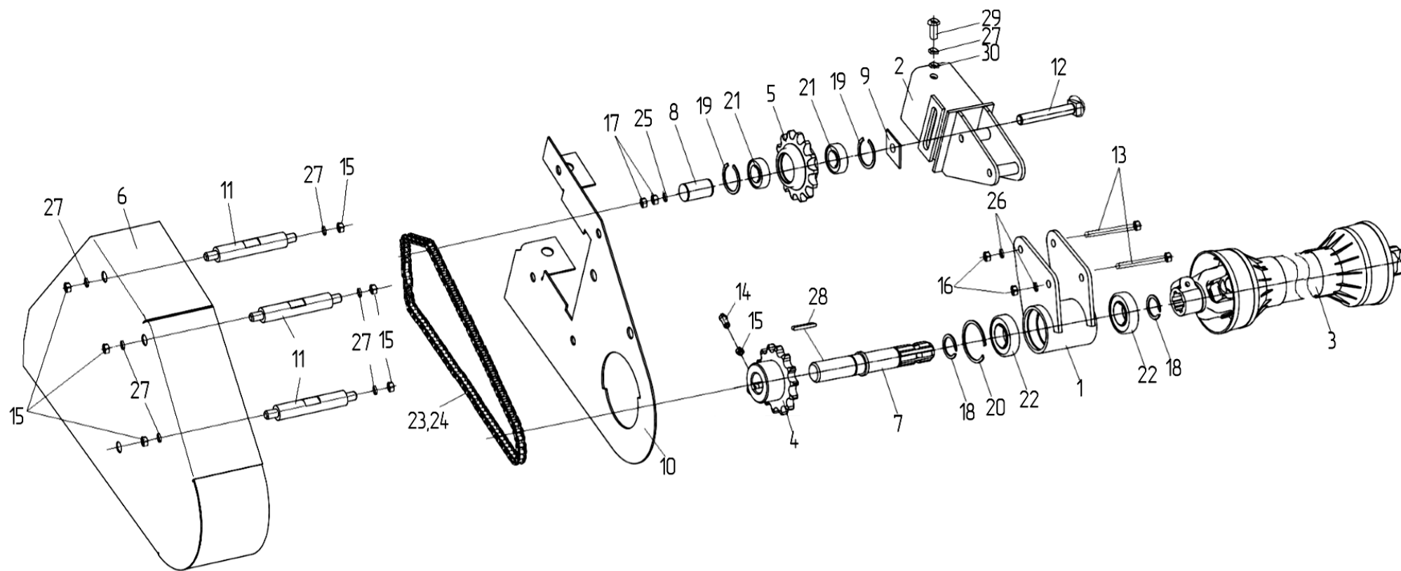
Рисунок 19 – Установка контрпривода ЖВЗ 7910000
