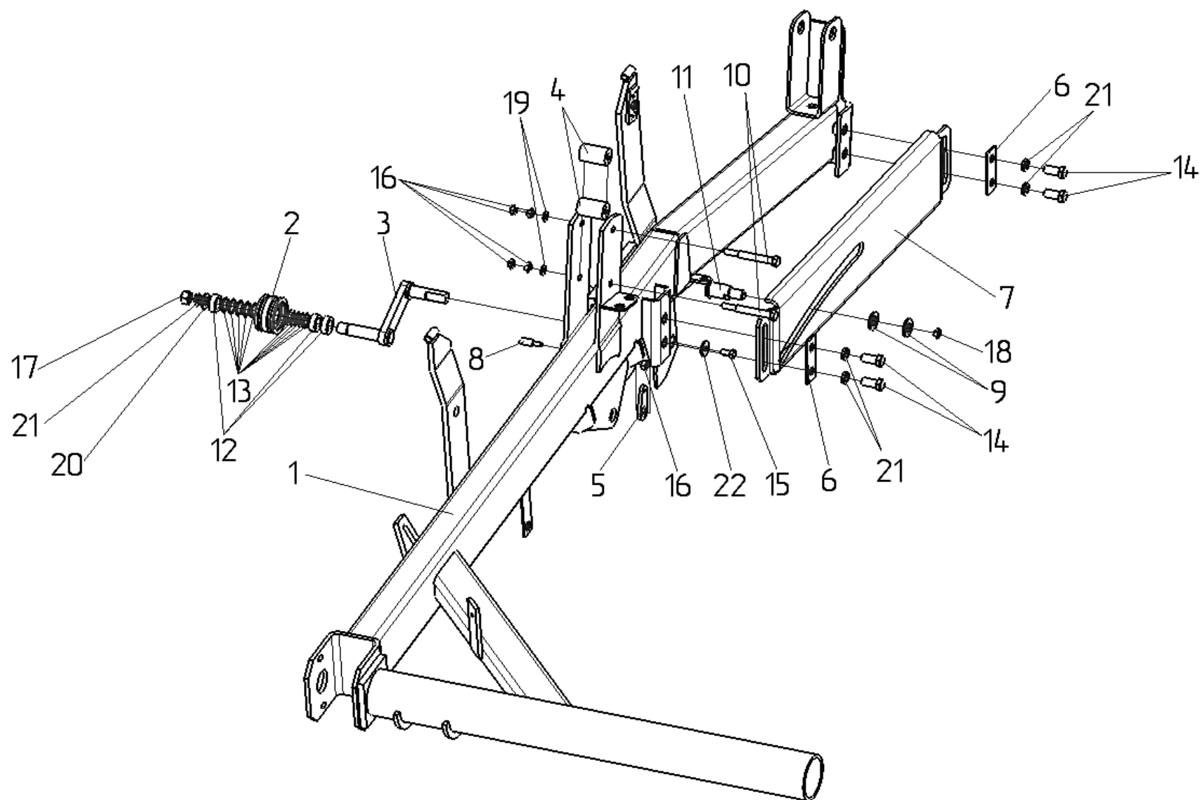
Рисунок 6 – Поддержка левая ЖВЗ-7-1508100Э
