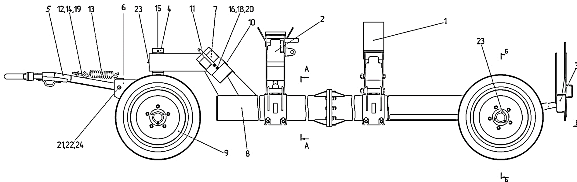
Рисунок 30 – Тележка транспортная ЖВЗ-7-1590010 (Лист 1)
