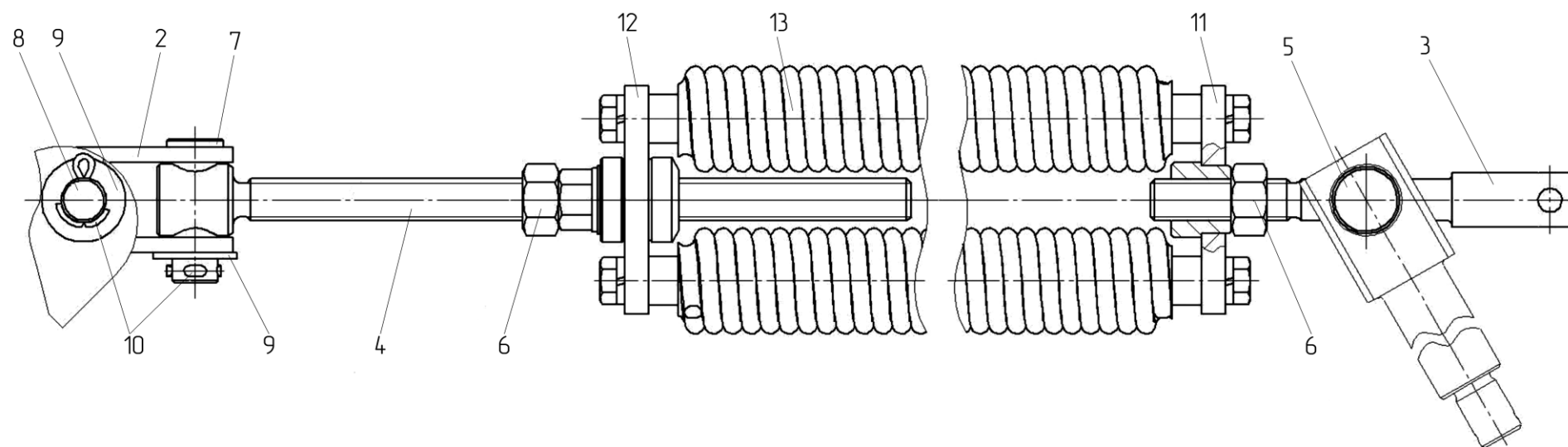
Рисунок 26 – Установка механизма копирования ЖВЗ 7064000
