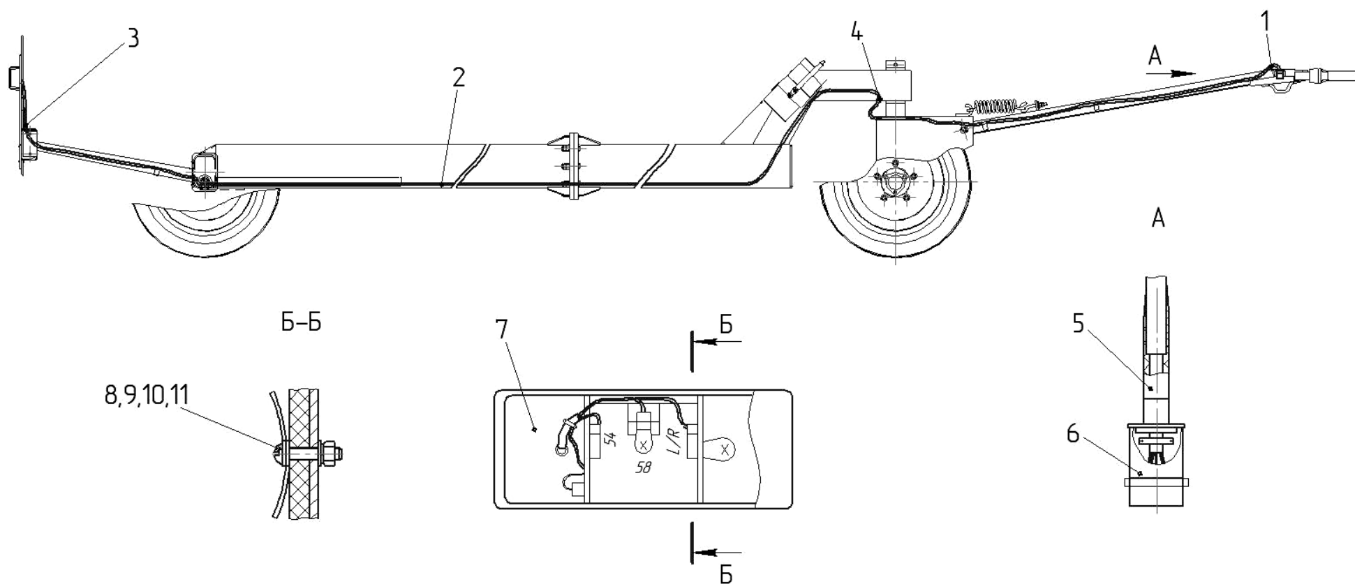
Рисунок 32 – Установка электрооборудования тележки транспортной ЖВЗ-7-0715900
