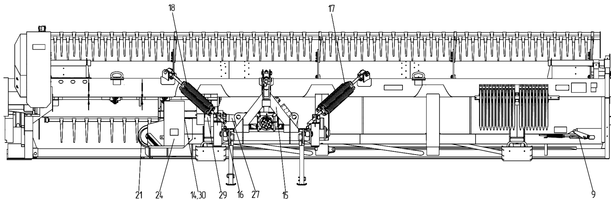
Рисунок 1а – Жатка валковая ЖВЗ-7УМ (ЖВЗ-7-1000000Э)
