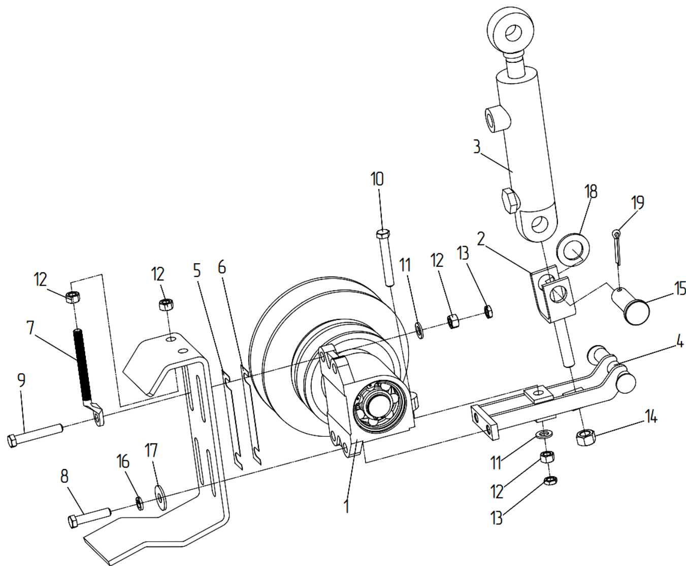
Рисунок 15 – Установка вариатора
