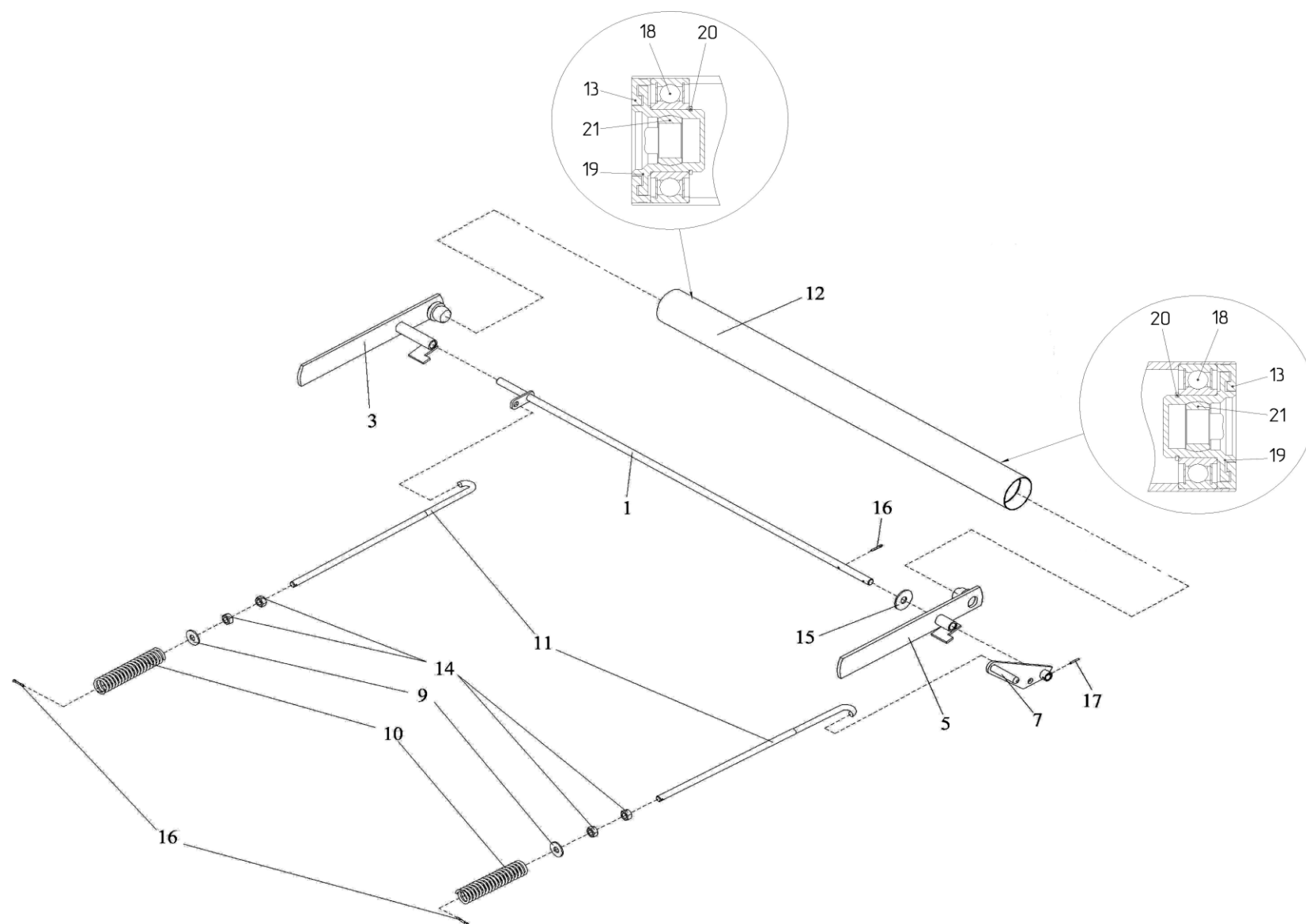
Рисунок 25 – Натяжное устройство ЖВЗ 1220000
