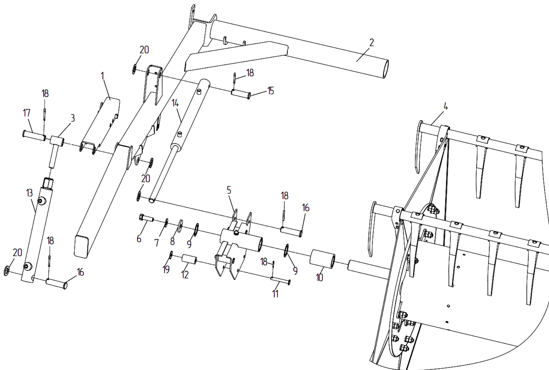
Рисунок 4 – Установка мотовила (вид справа)
