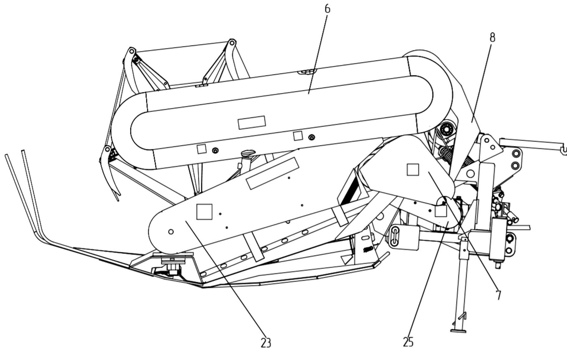
Рисунок 1г – Жатка валковая ЖВЗ-7УМ (ЖВЗ-7-1000000Э)
