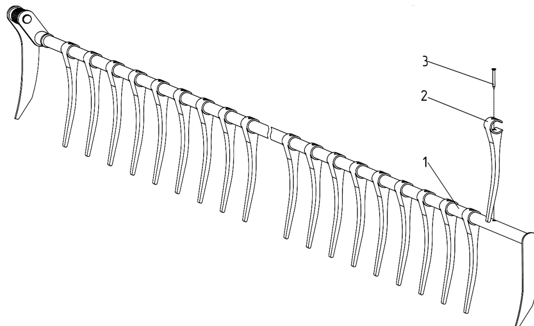
Рисунок 3 – Граблина ЖВЗ-7-1503550Э/-01
