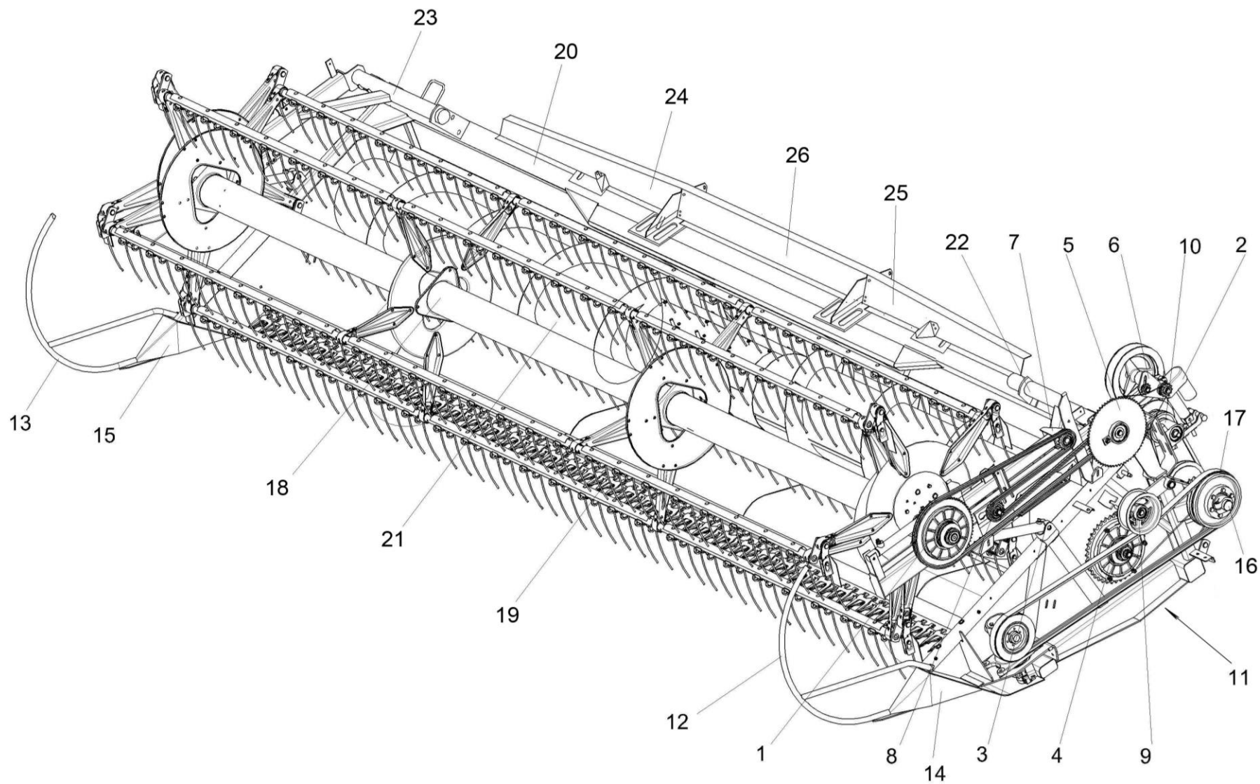
Рисунок 2 – Жатка для зерновых культур КЗР 1500010Б-09
