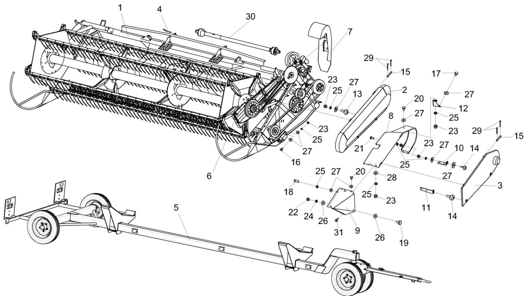
Рисунок 1 – Жатка для зерновых культур ЖЗК-7-6 КЗР 1500000-09
