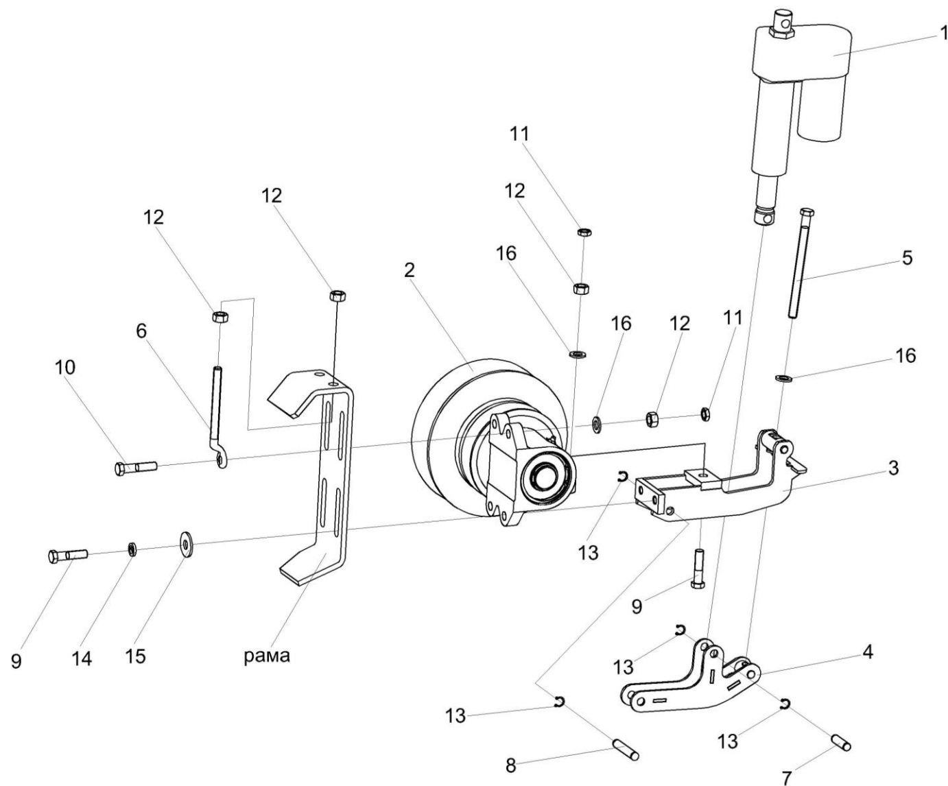
Рисунок 10 – Установка электромеханизма КЗР 0700390-01 или МК-150М-02
