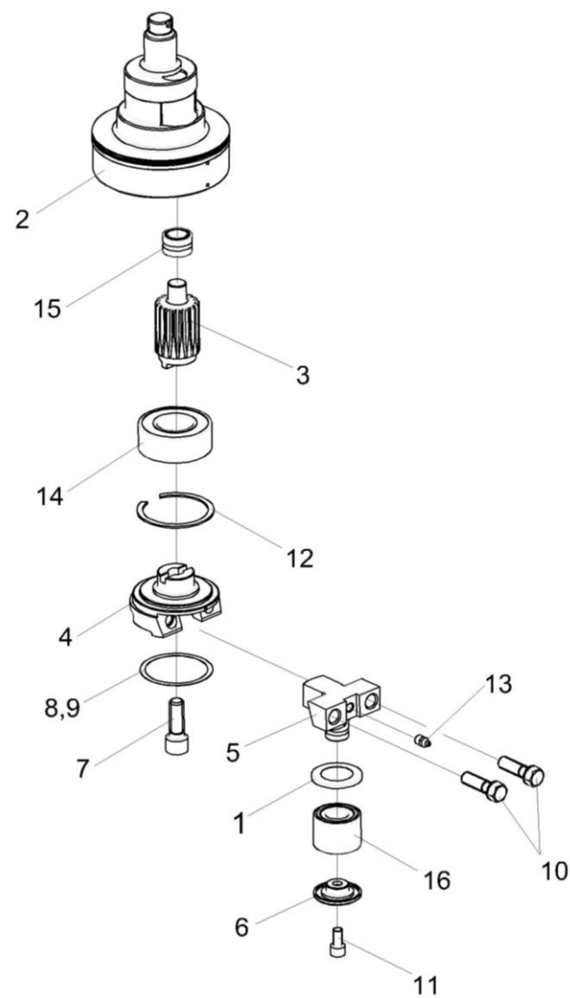
Рисунок 28 – Водило КЗР 1517230
