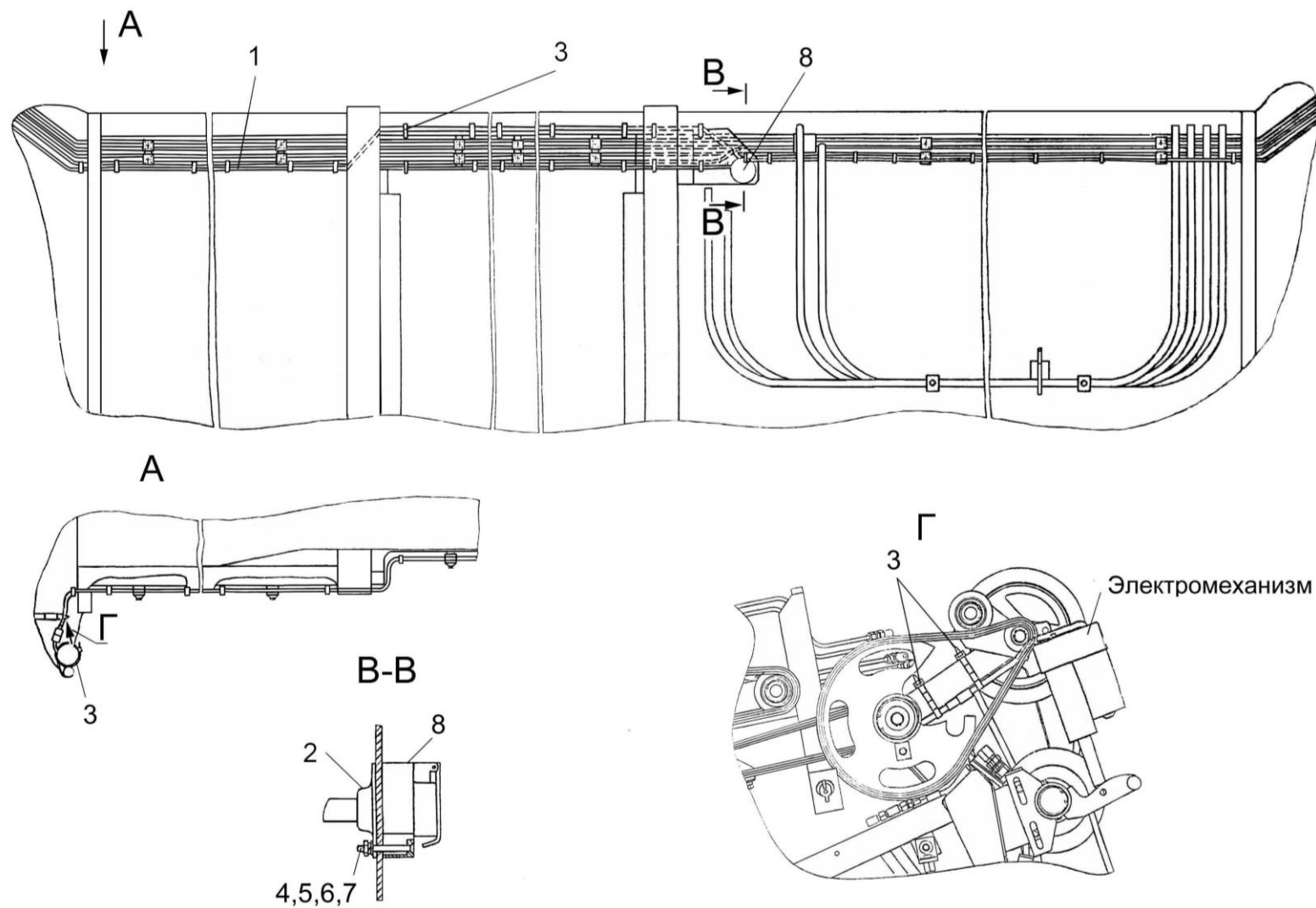
Рисунок 42 – Электрооборудование жатки для зерновых культур КЗР 1500000-09
