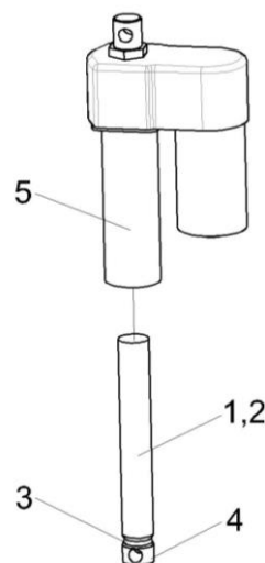
Рисунок 11 – Электромеханизм КЗР 0700390-01
