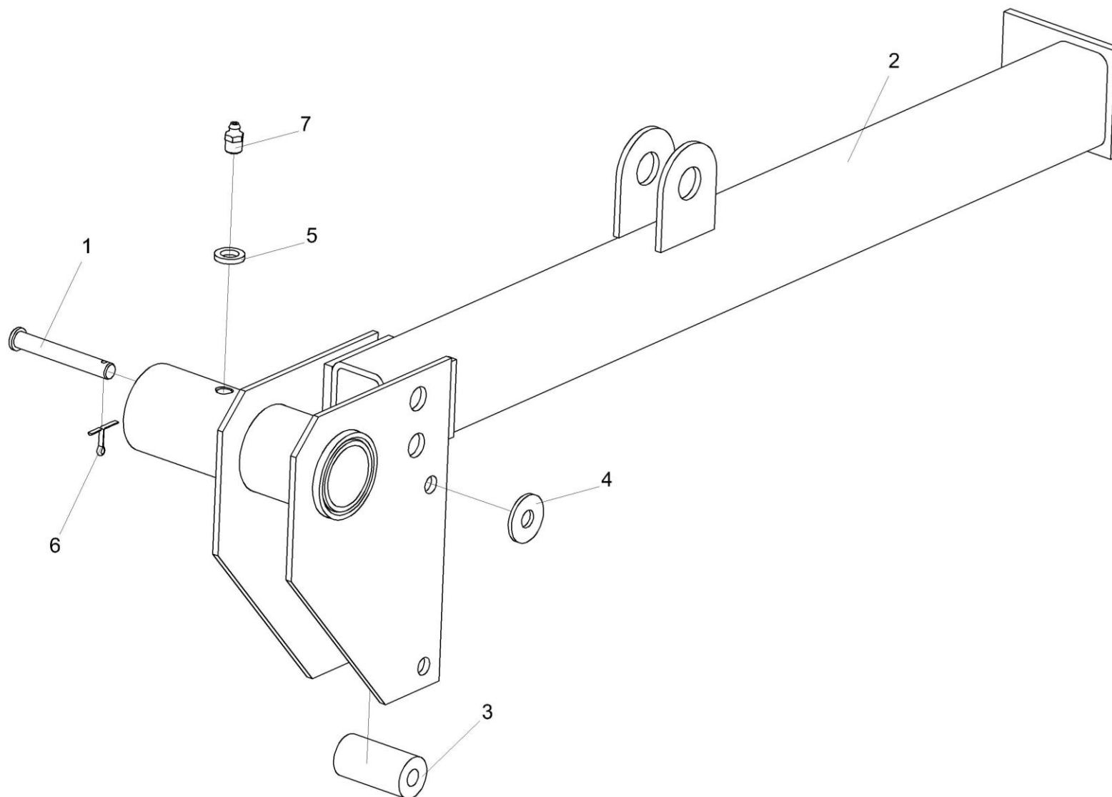
Рисунок 21 – Направляющая КЗР 1573080-01
