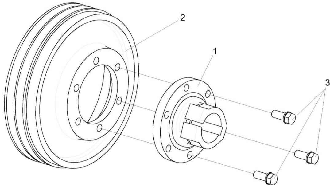
Рисунок 9 – Шкив КЗР 1524020
