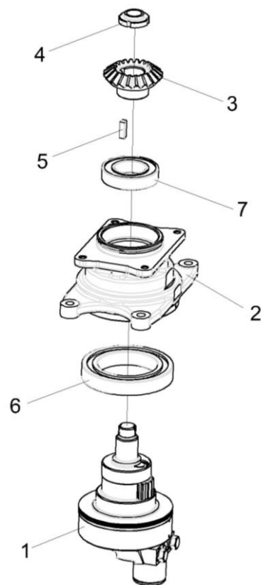
Рисунок 37 – Стакан КЗР 1517220
