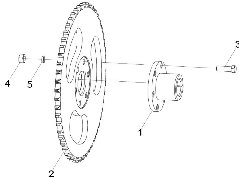
Рисунок 14 – Звездочка КЗК-1420-1527290
