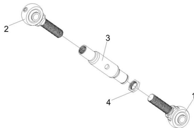
Рисунок 61 – Тяга верхняя КПР 9122000
