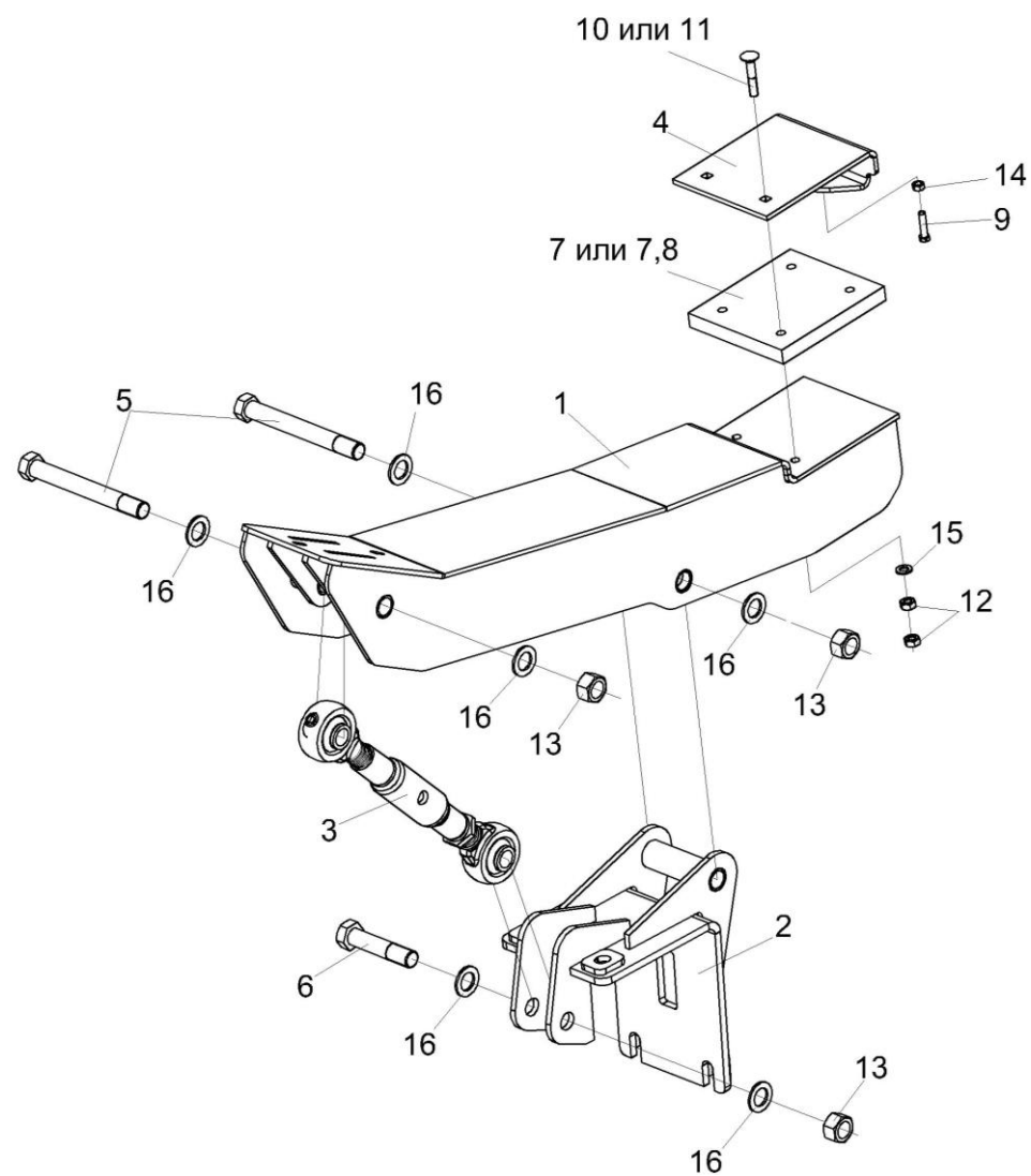
Рисунок 60 – Ложемент КЗК-1475-2595000
