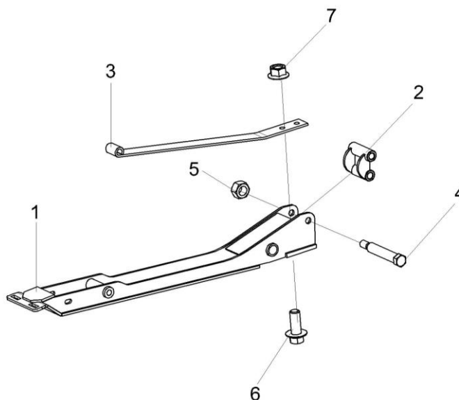
Рисунок 41 – Рычаг КЗК 2503000Б
