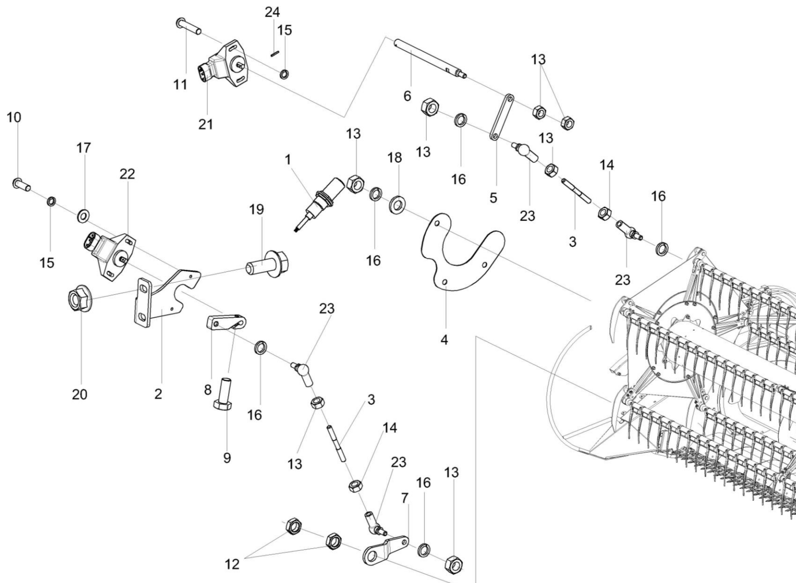
Рисунок 53 – Установка датчиков КЗК-1492-2506000 (лист 2)
