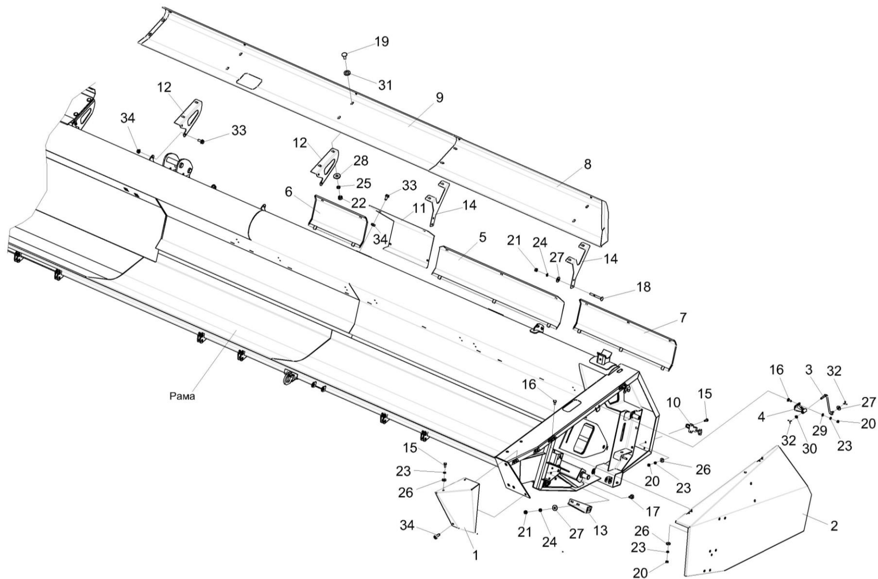
Рисунок 49 – Установка ограждений КЗК-1492-2525000 (лист 1)
