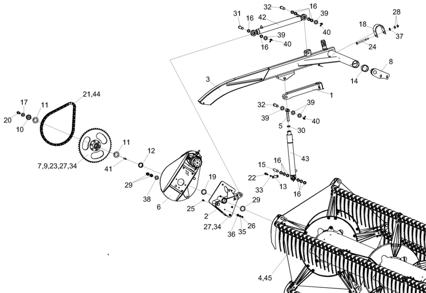
Рисунок 10 – Установка мотовила КЗК-1492-2503000 (лист 2)
