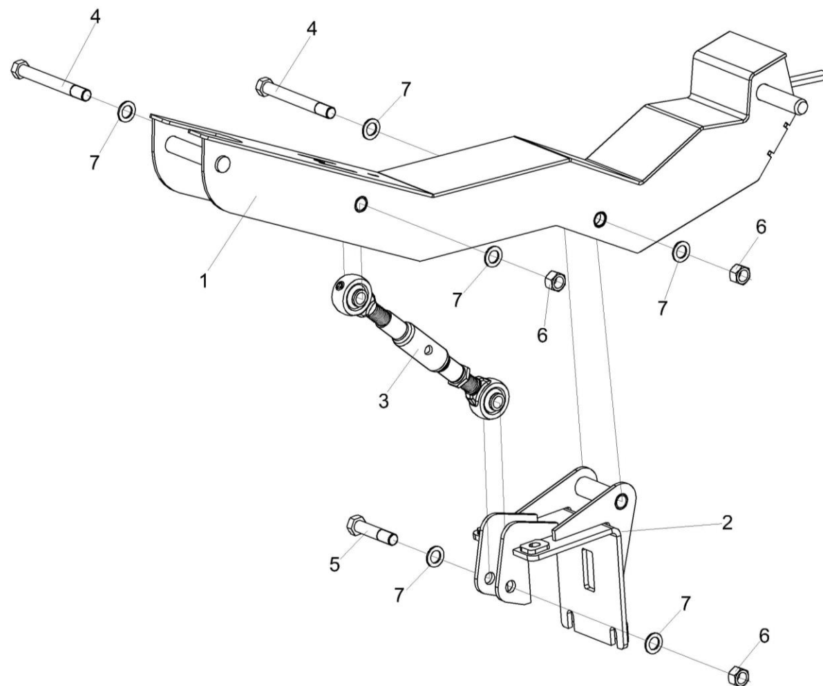
Рисунок 59 – Ложемент КЗК-1475-2594000
