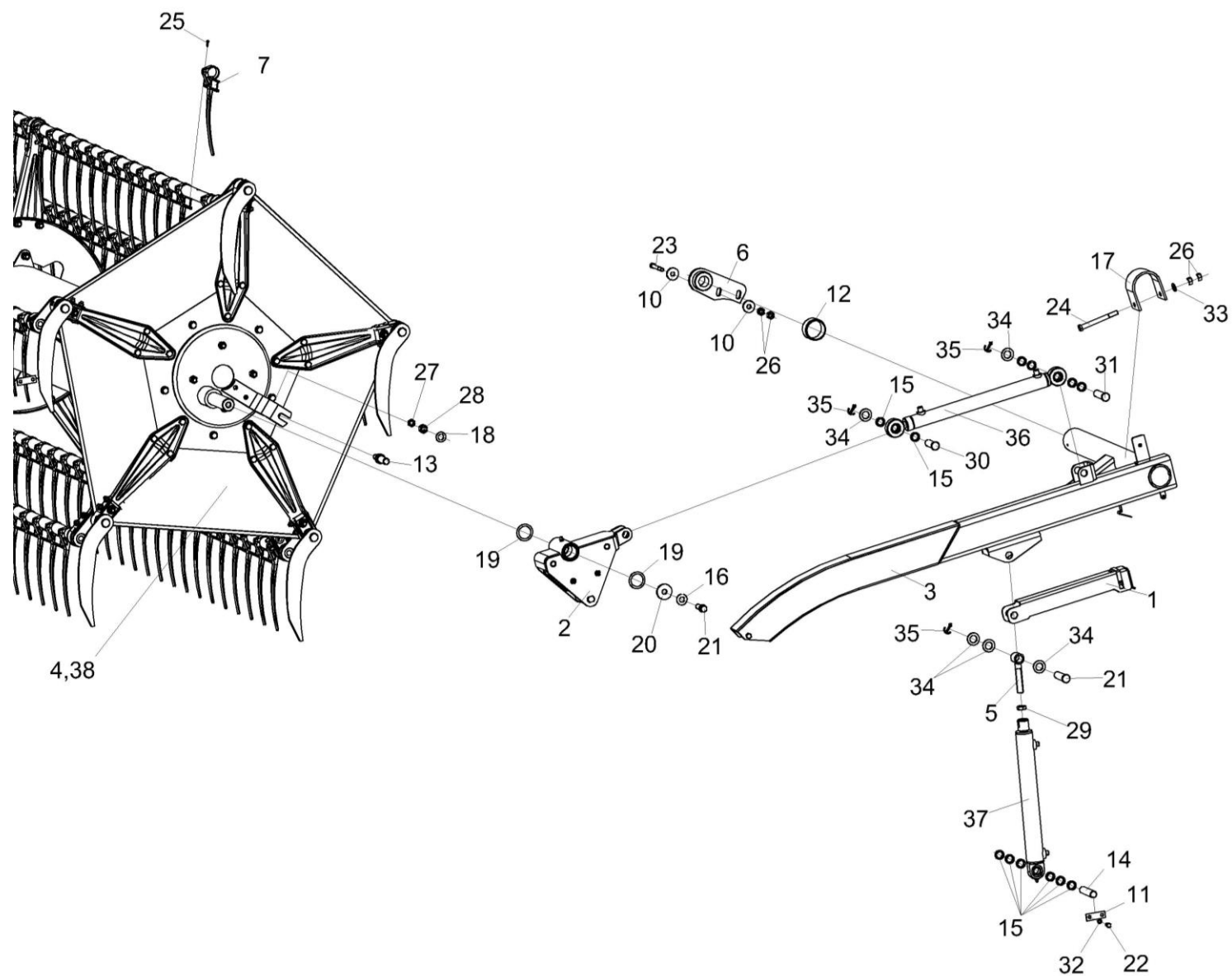
Рисунок 9 – Установка мотопила КЗК-1492-2503000 (лист 1)
