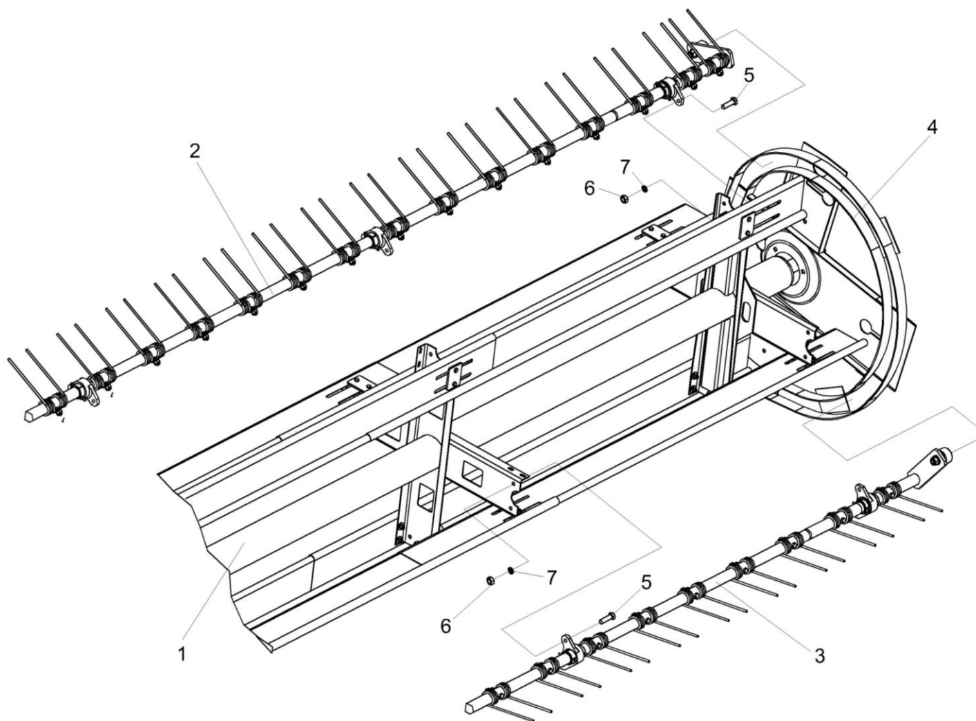
Рисунок 22 – Установка граблин
