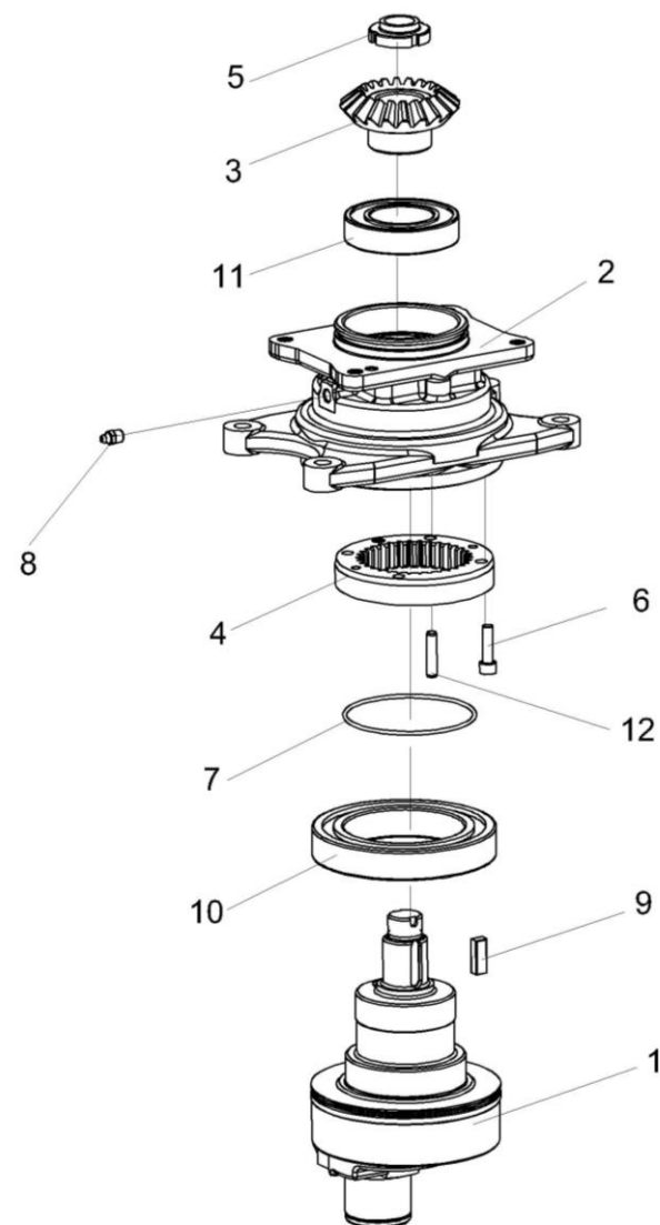
Рисунок 33 – Стакан КЗР 1517220
