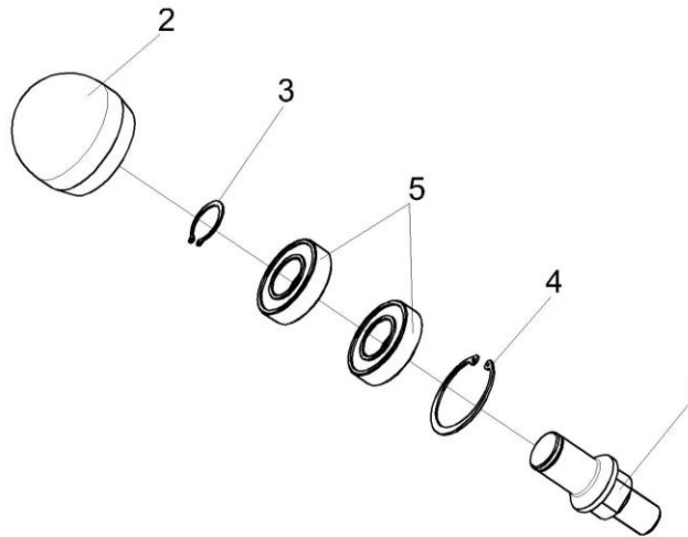
Рисунок 10 – Ролик КЗК 1780010
