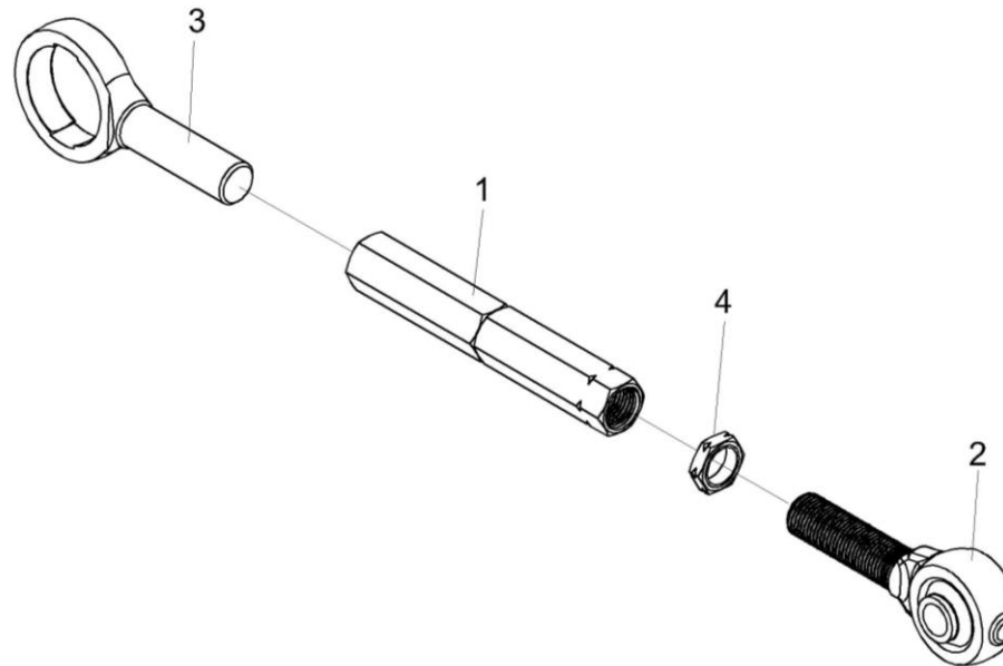
Рисунок 11 – Тяга КЗК-8-1780300-02
