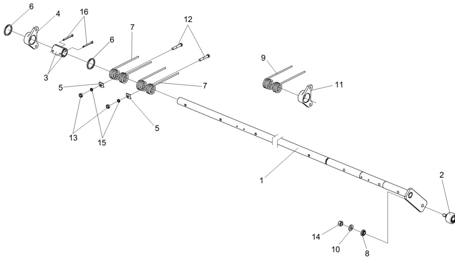
Рисунок 23 – Граблина КГК 1203020
