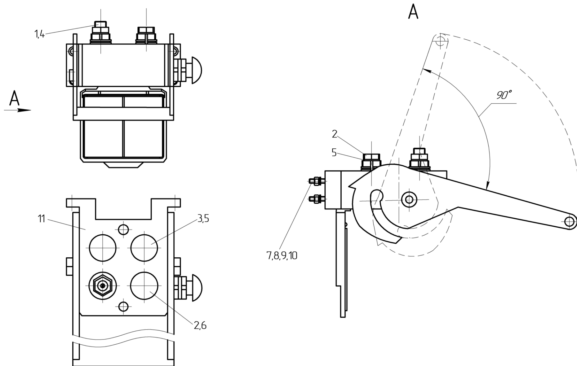
Рисунок 39 – Разъем гидравлический многофункциональный ПЗЗ 2180390
