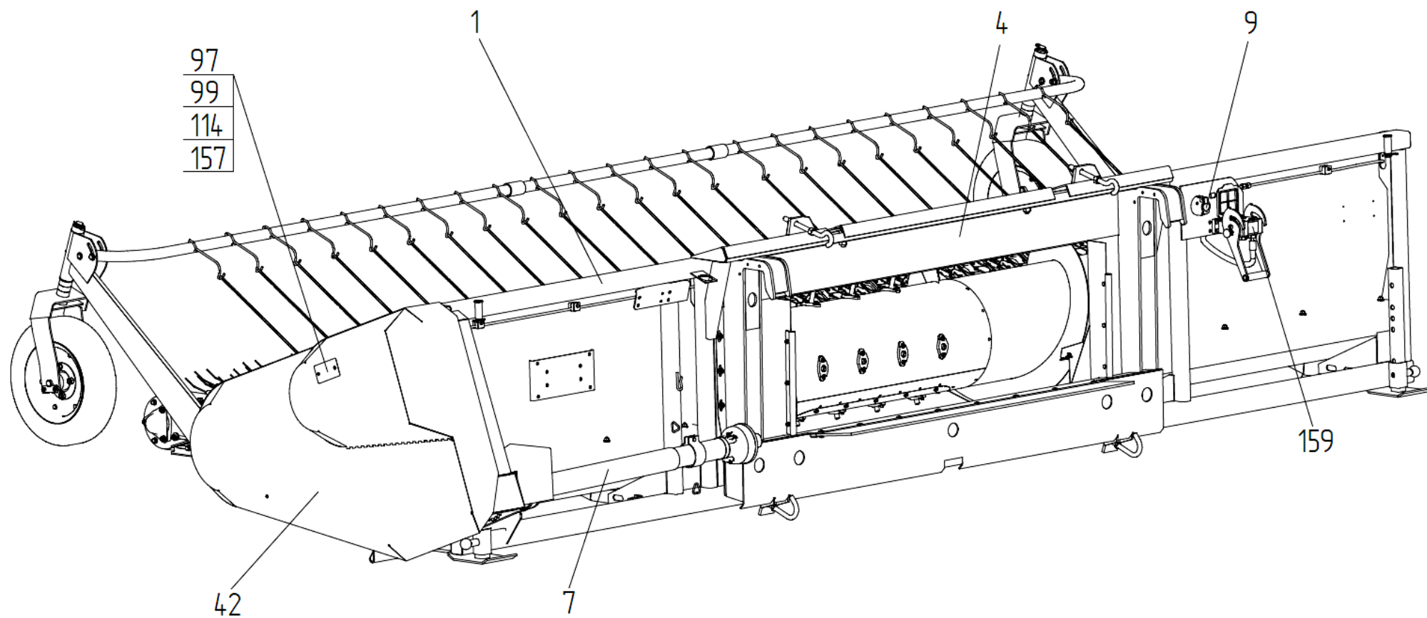
Рисунок 26 – Подборщик зерновой ПЗ-4,4-8 (ПЗЗ 2200000/-01/-02/-03/-04/-05/-06/-07/-08/-09/-10/-11)
