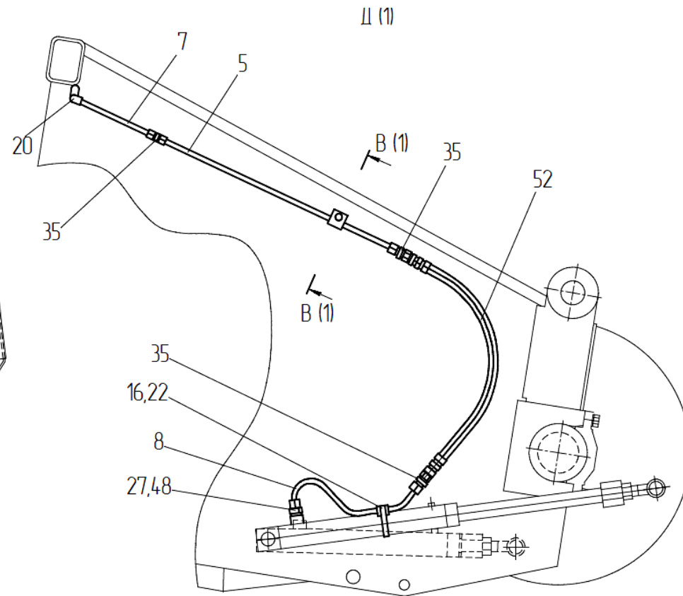
Рисунок 37 – Гидросистема подборщика ПЗЗ 2283000 (Лист 2)
