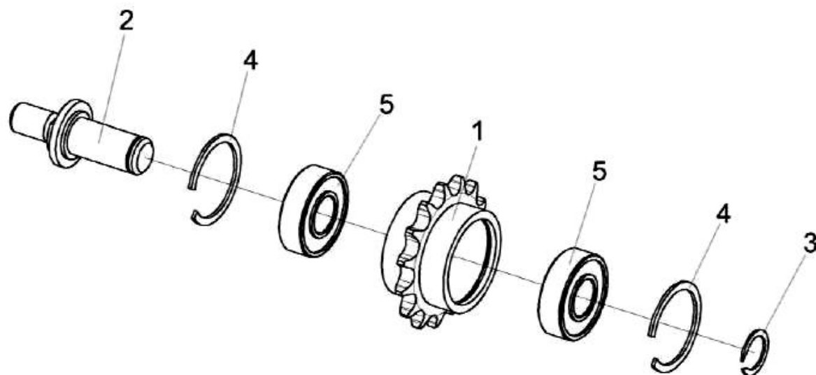
Рисунок 18 – Устройство натяжное КЗК 1914040
