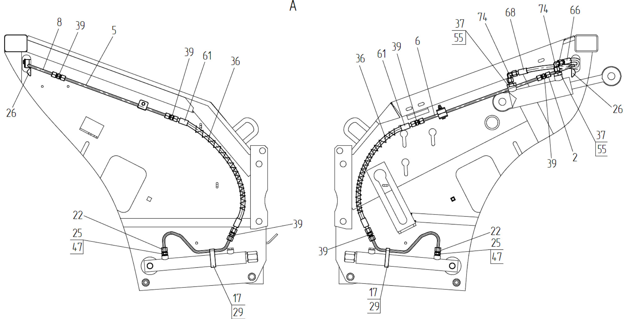
Рисунок 38 – Гидросистема подборщика ПЗЗ 2284000 (Лист 2)
