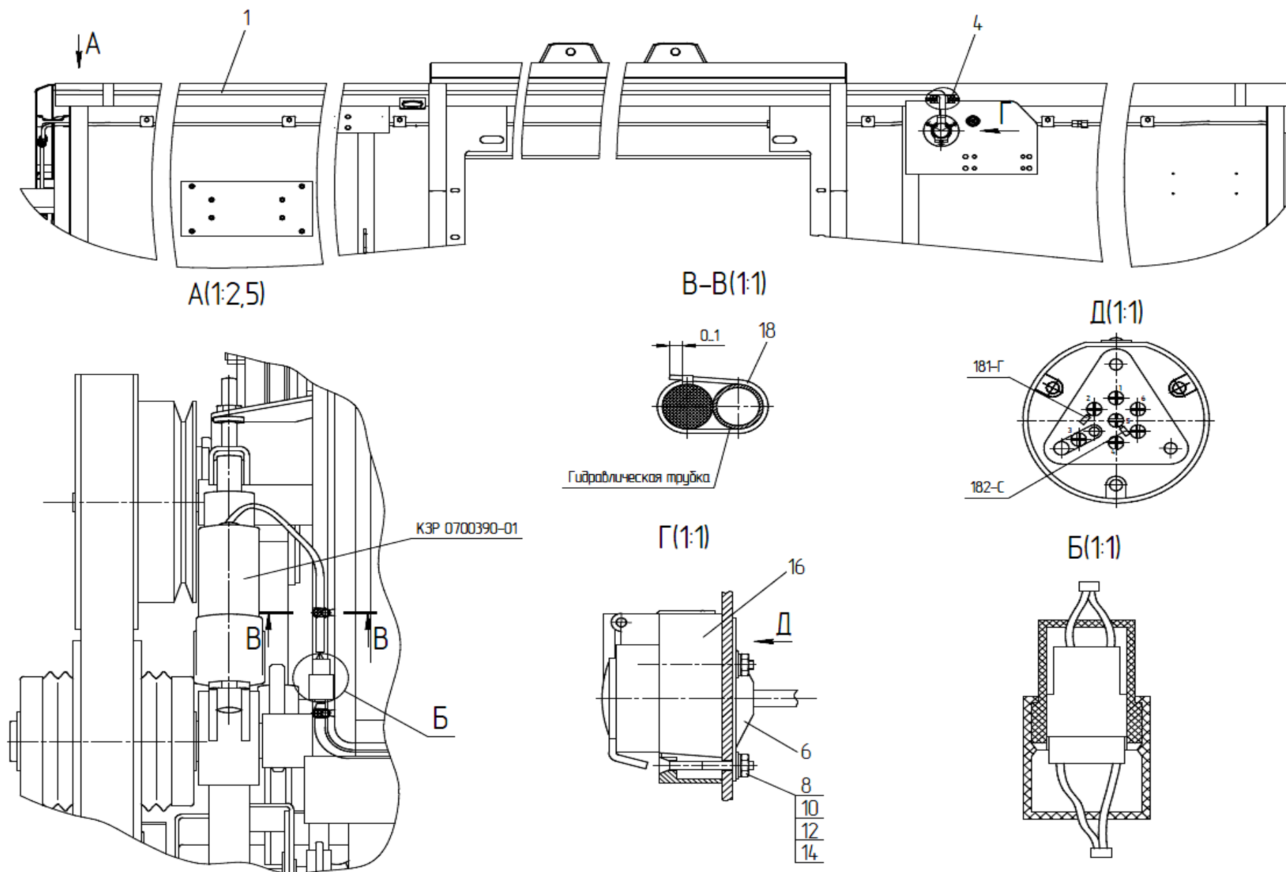
Рисунок 32 – Электрооборудование подборщика зернового ПЗЗ 2271000
