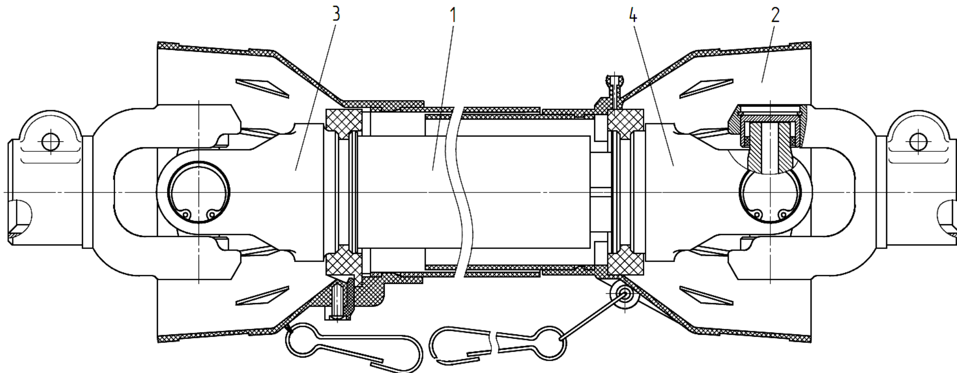
Рисунок 22 – Вал карданный телескопический ПЗЗ 2209000
