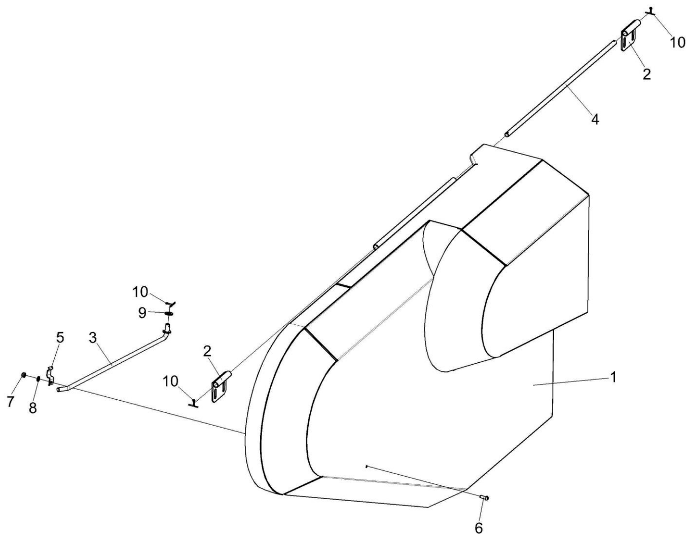
Рисунок 23 – Ограждение КЗР 1918000
