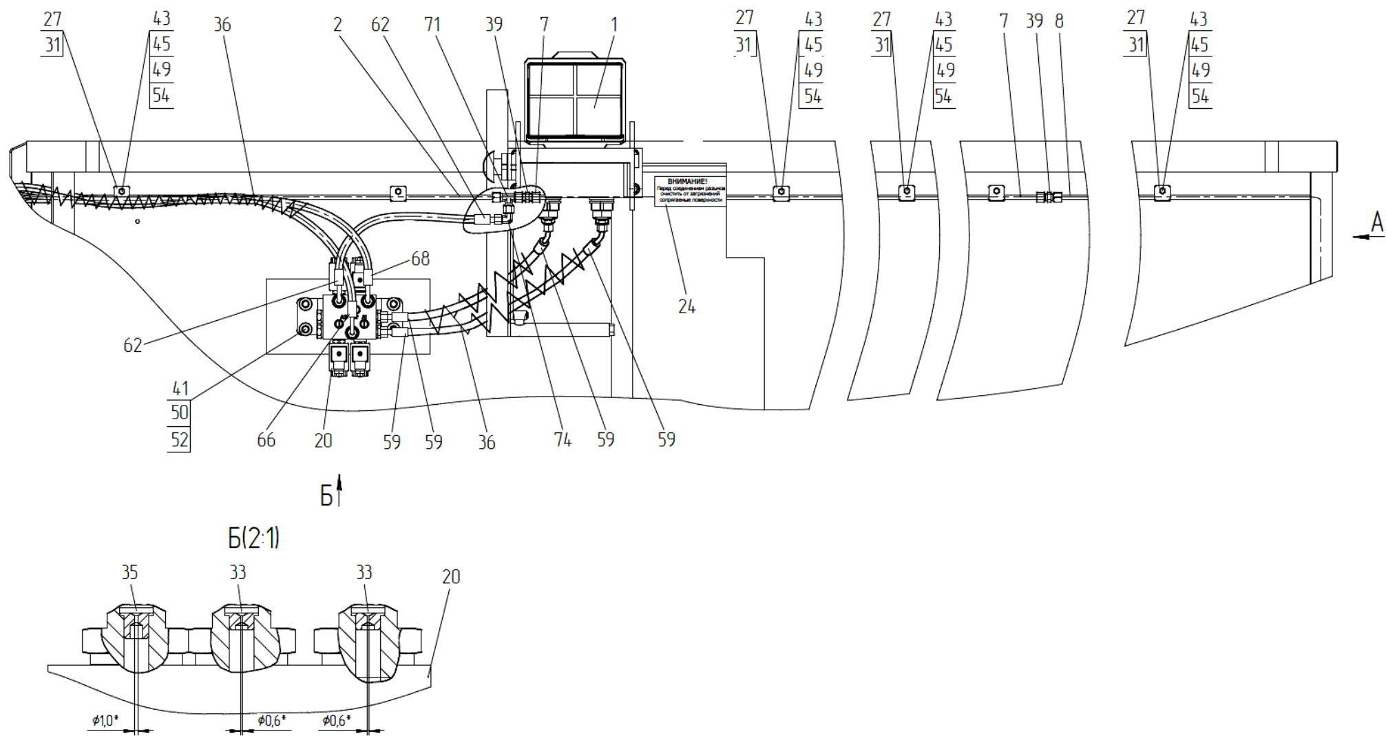
Рисунок 38 – Гидросистема подборщика ПЗЗ 2284000 (Лист 1)
