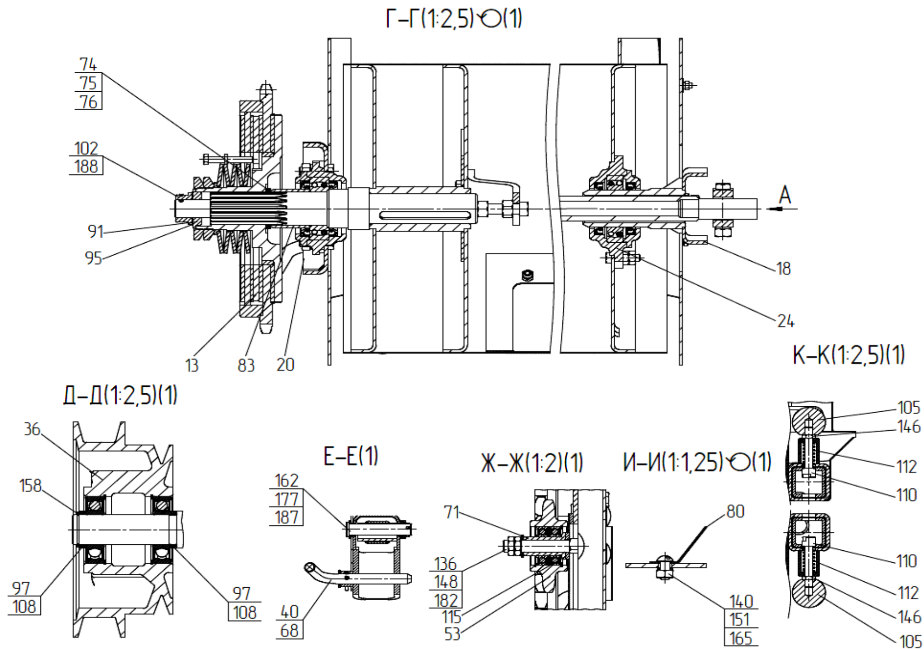
Рисунок 4 – Платформа ПЗЗ 2200010 (Лист 2)
