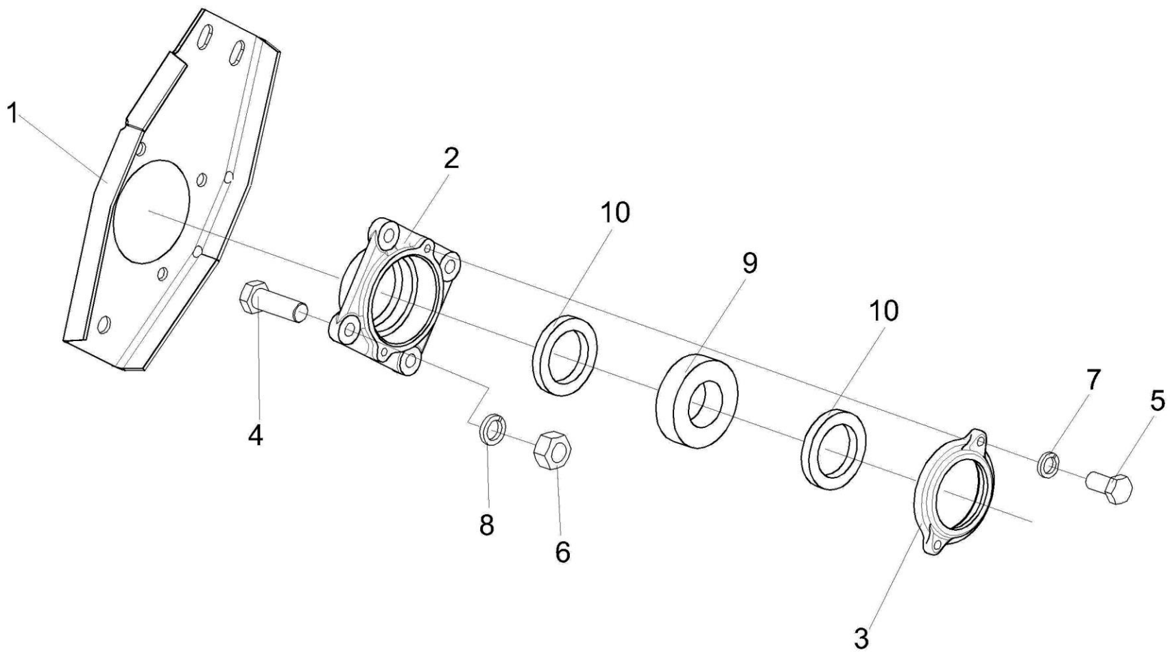
Рисунок 11 – Опора K3P 1502110-01
