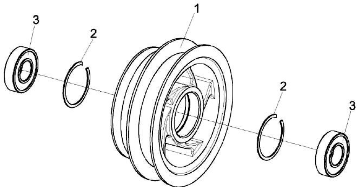
Рисунок 14 – Шкив КЗР 1906000
