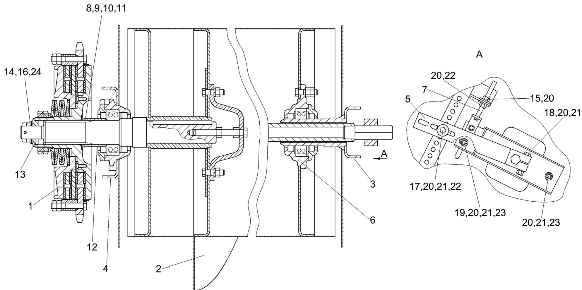
Рисунок 7 – Установка шнека ПЗЗ 1502000
