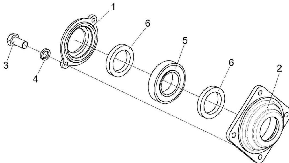
Рисунок 12 – Корпус КЗР 1502160
