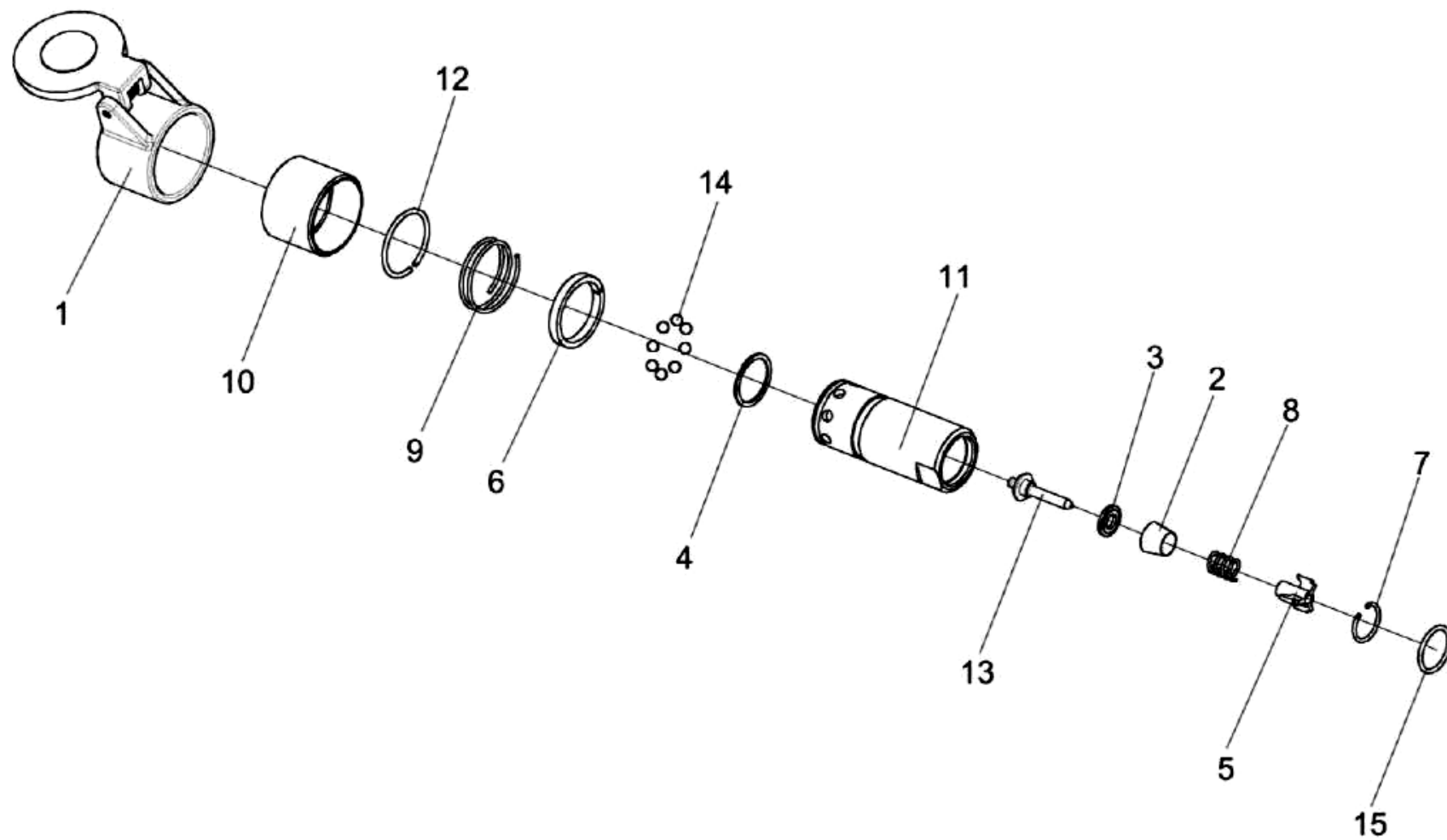
Рисунок 36 – Полумуфта наружная МС 12-3-010
