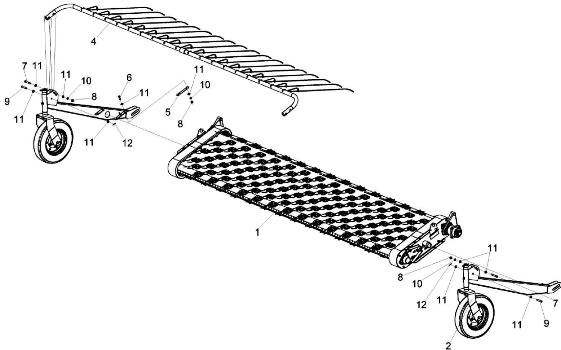
Рисунок 24 – Транспортер ПЗЗ 1920000
