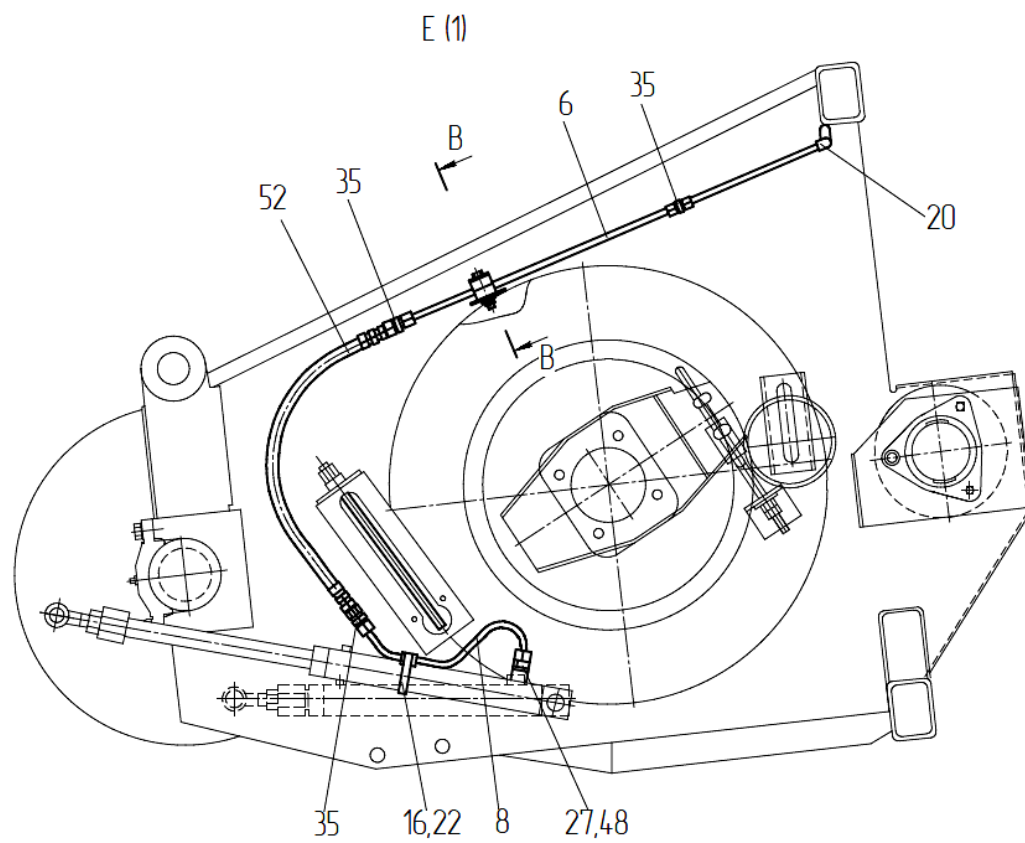
Рисунок 37 – Гидросистема подборщика ПЗЗ 2283000 (Лист 2)
