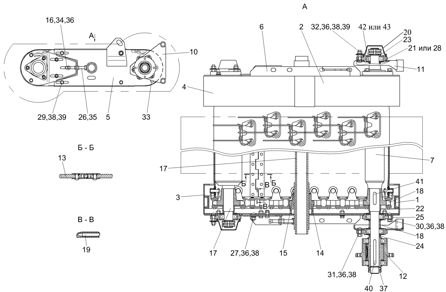
Рисунок 25 – Транспортер ПЗЗ 1920040
