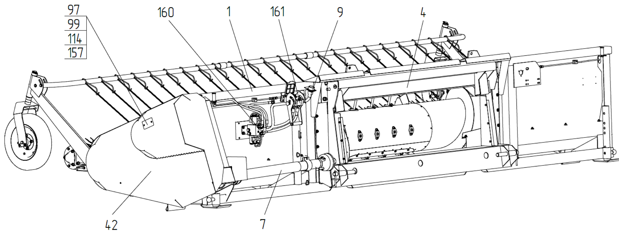
Рисунок 2в – Подборщик зерновой ПЗ-4,4-8 (ПЗЗ 2200000/-01/-02/-03/-04/-05/-06/-07/-08/-09/-10/-11)
