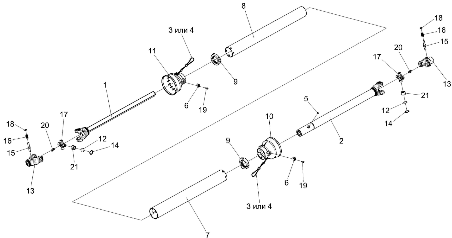
Рисунок 21 – Вал карданный телескопический ПЗЗ 1909000
