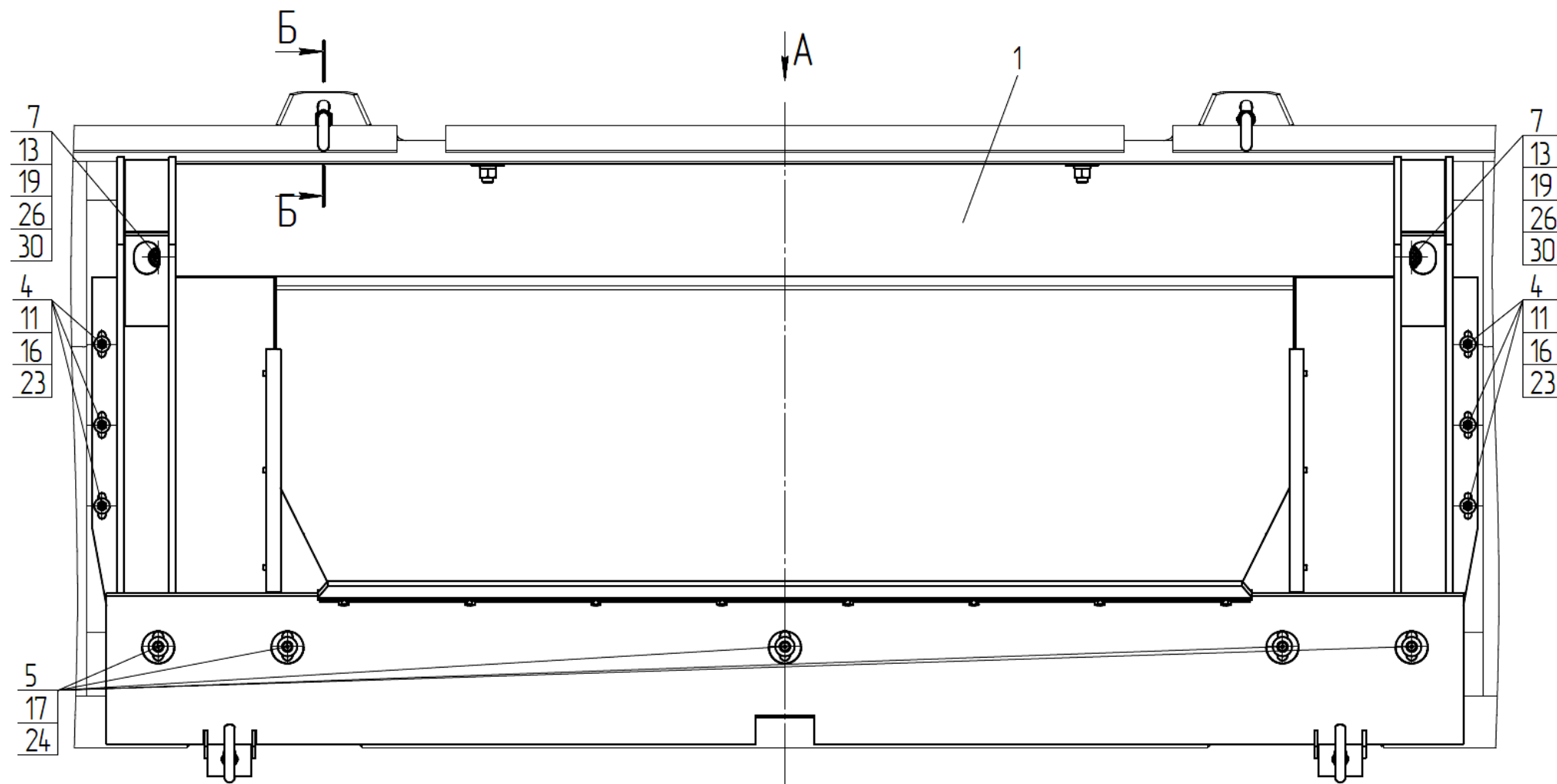
Рисунок 5а – Установка переходной рамки ПЗЗ 2201100А (Лист 1)
