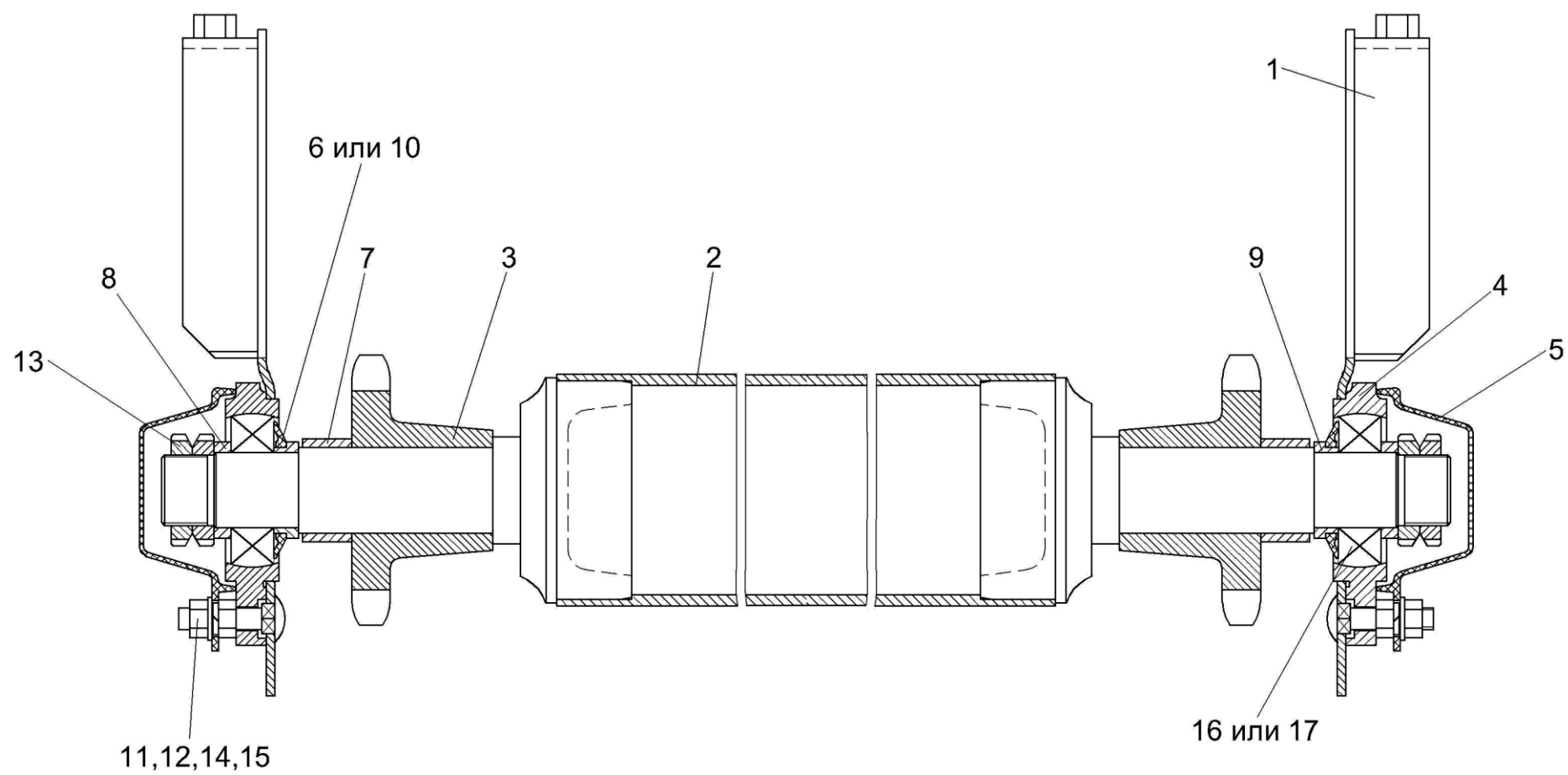
Рисунок 26 – Вал ведомый ПЗЗ 1924000
