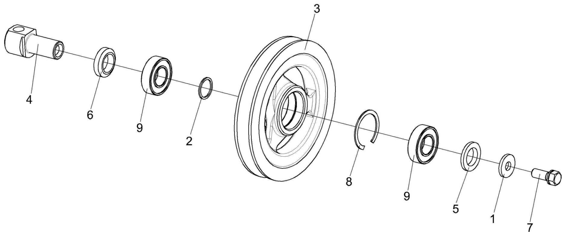
Рисунок 15 – Шкив натяжной КЗР 1907000
