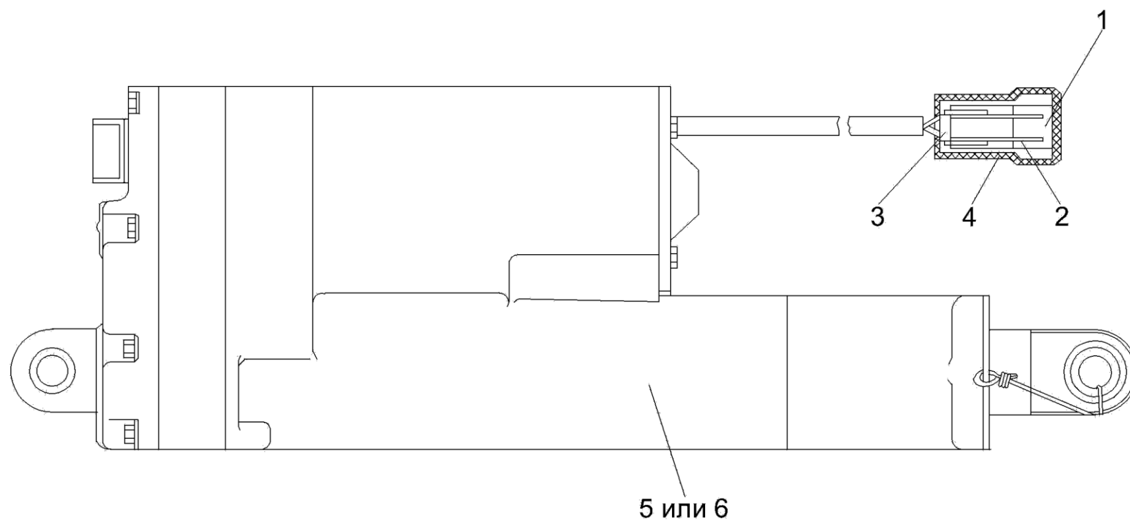
Рисунок 20 – Электромеханизм КЗР 0700390-01
