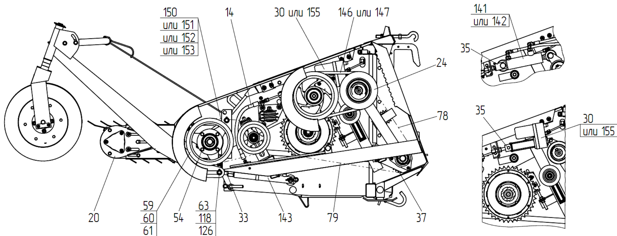
Рисунок 2 – Подборщик зерновой ПЗ-4,4-8 (ПЗЗ 2200000/-01/-02/-03/-04/-05/-06/-07/-08/-09/-10/-11)
