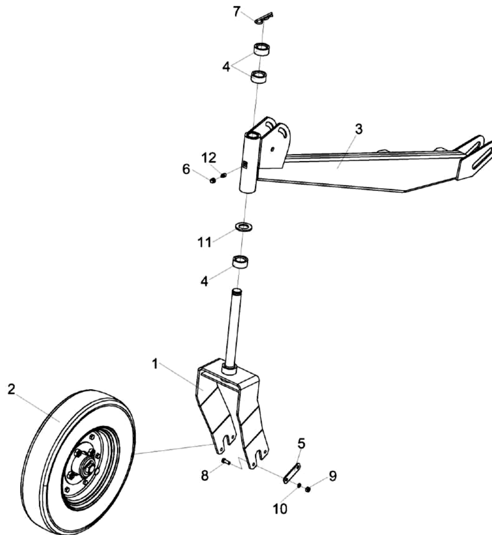
Рисунок 28 – Колесо КЗР 1925000
