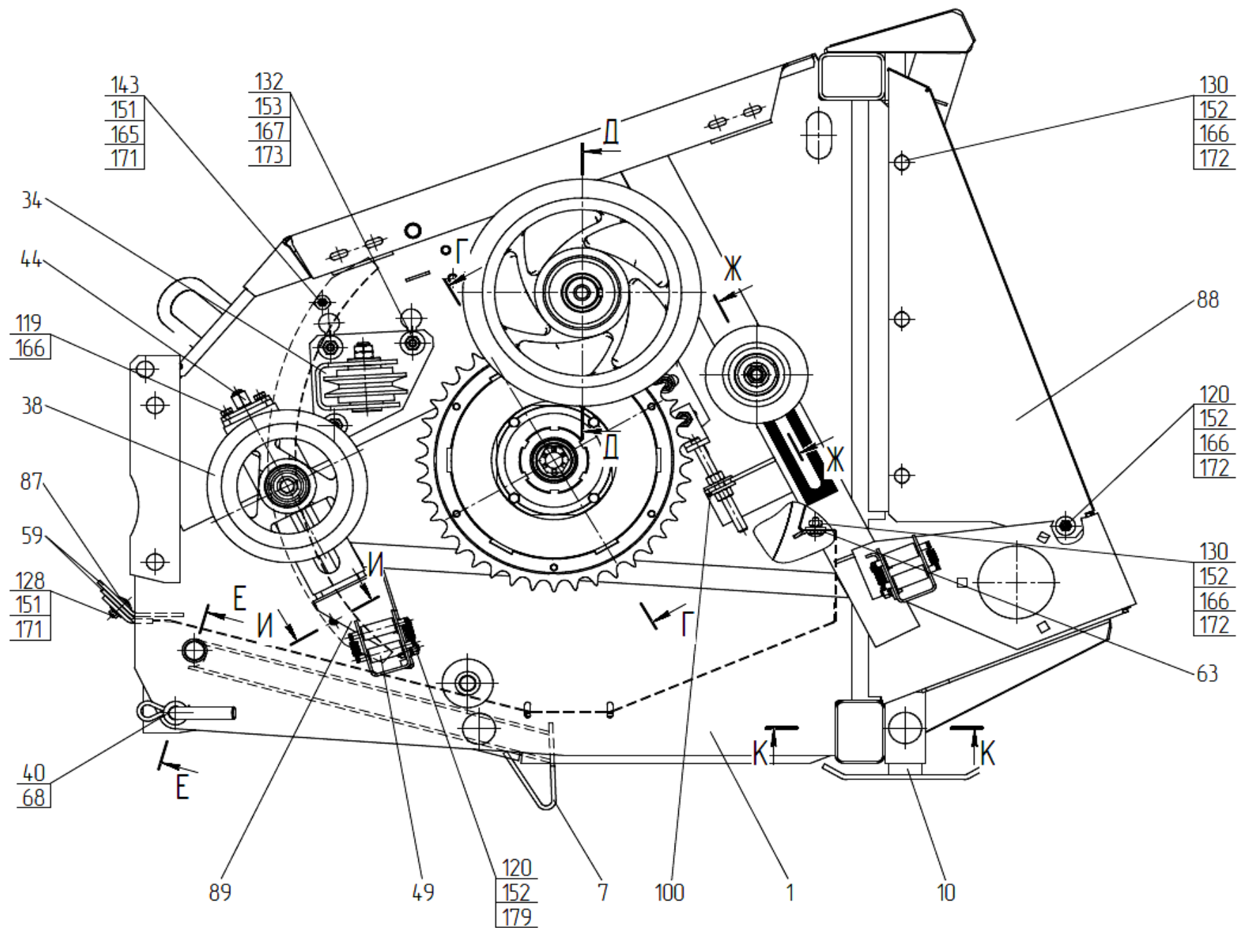
Рисунок 3 – Платформа ПЗЗ 2200010 (Лист 1)
