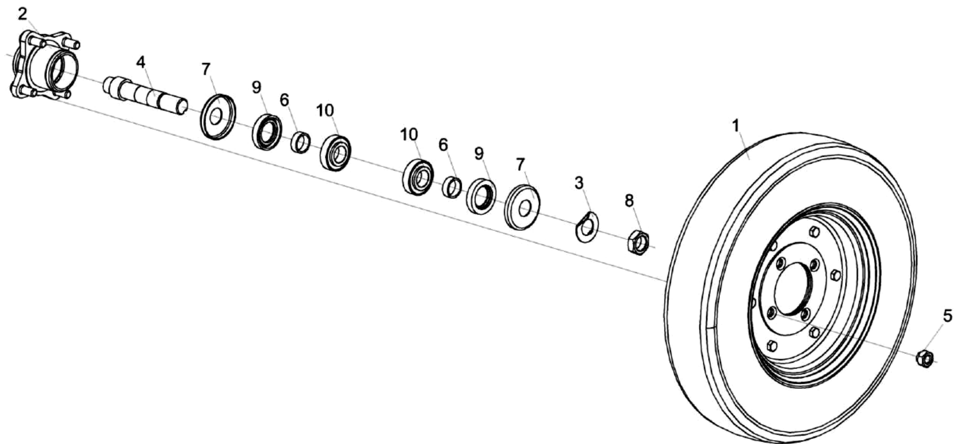
Рисунок 30 – Колесо 1925070
