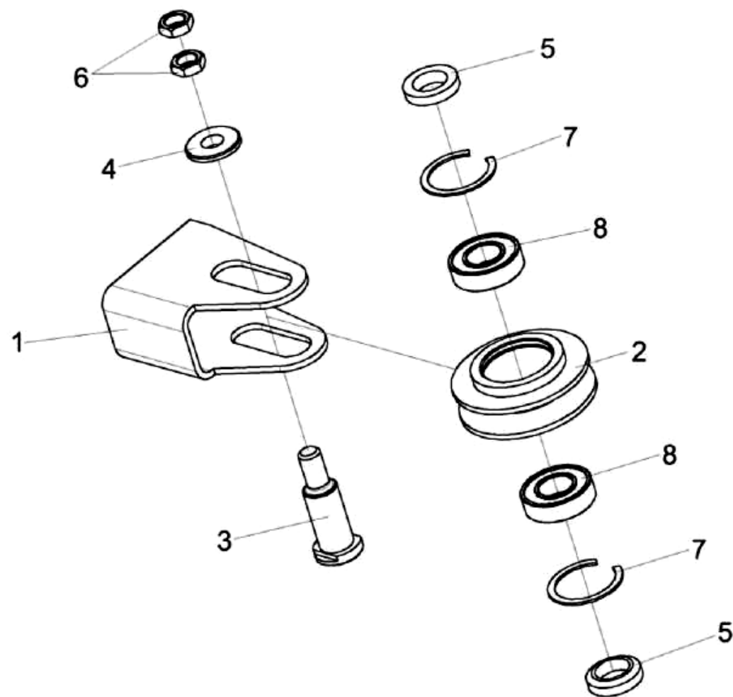
Рисунок 13 – Ролик КЗР 1905000
