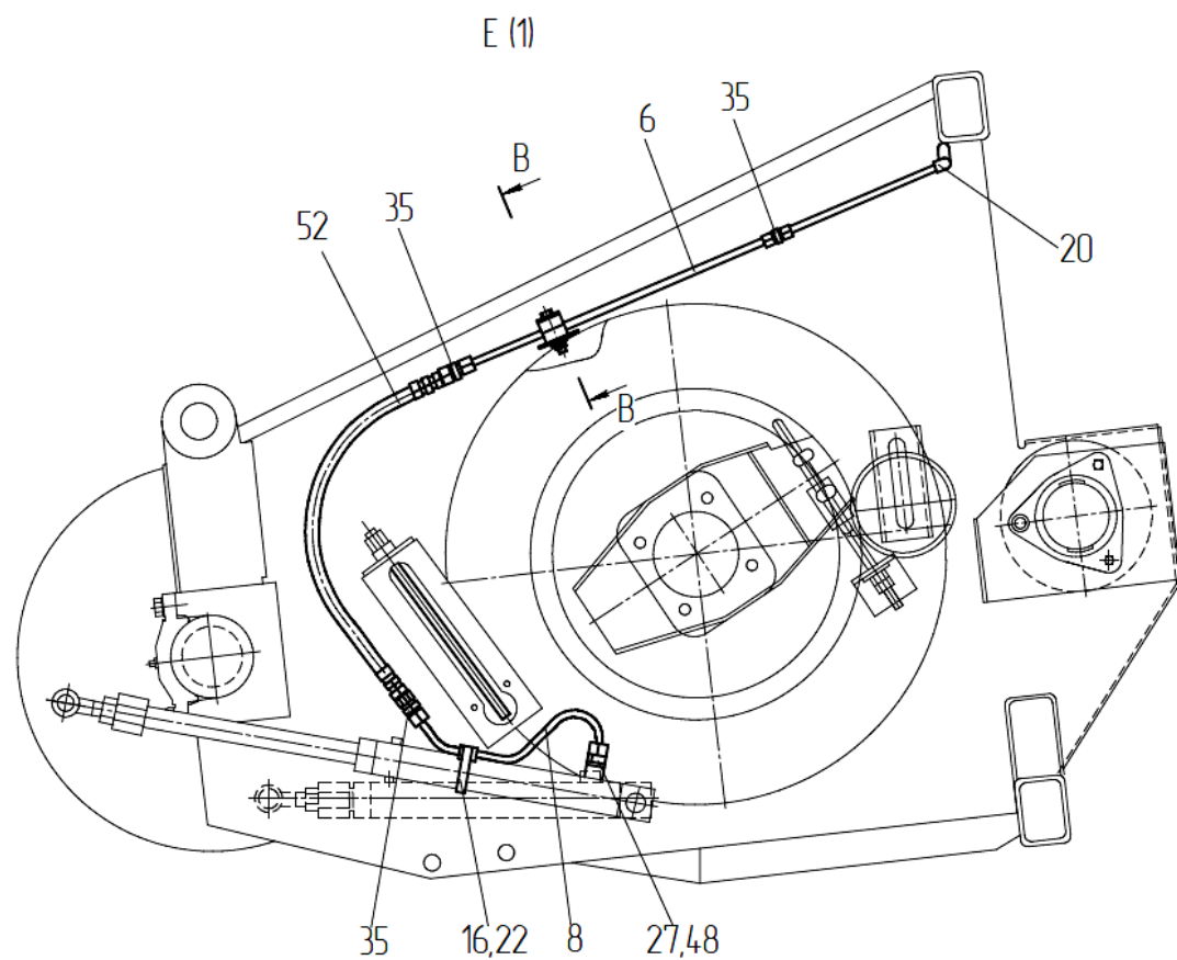
Рисунок 34 – Гидросистема подборщика ПЗЗ 2281000 (Лист 2)
