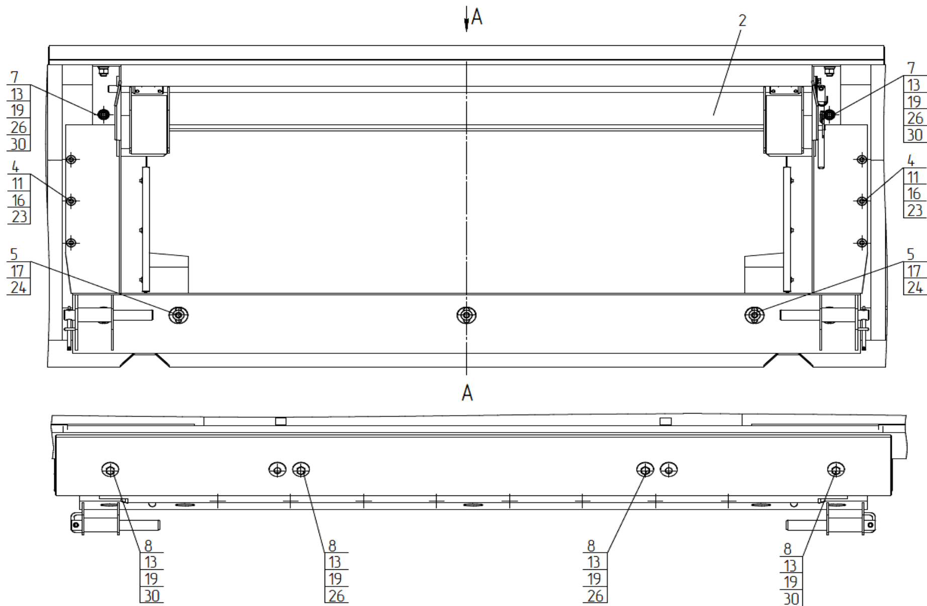
Рисунок 6 – Установка переходной рамки ПЗЗ 2201200
