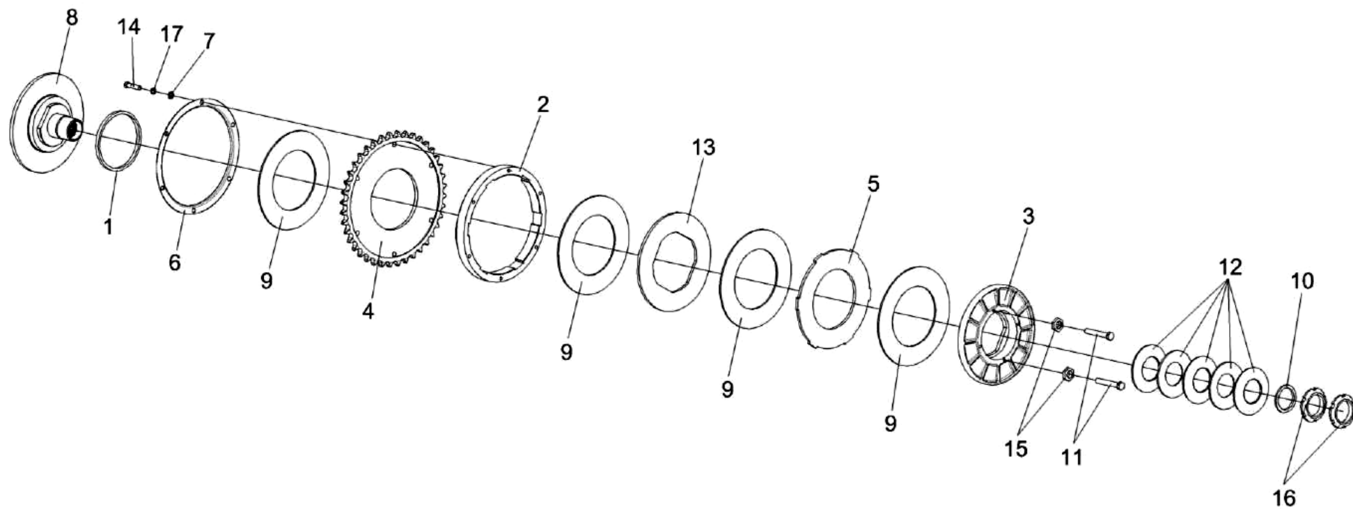
Рисунок 9 – Муфта предохранительная КГС 0202100-02
