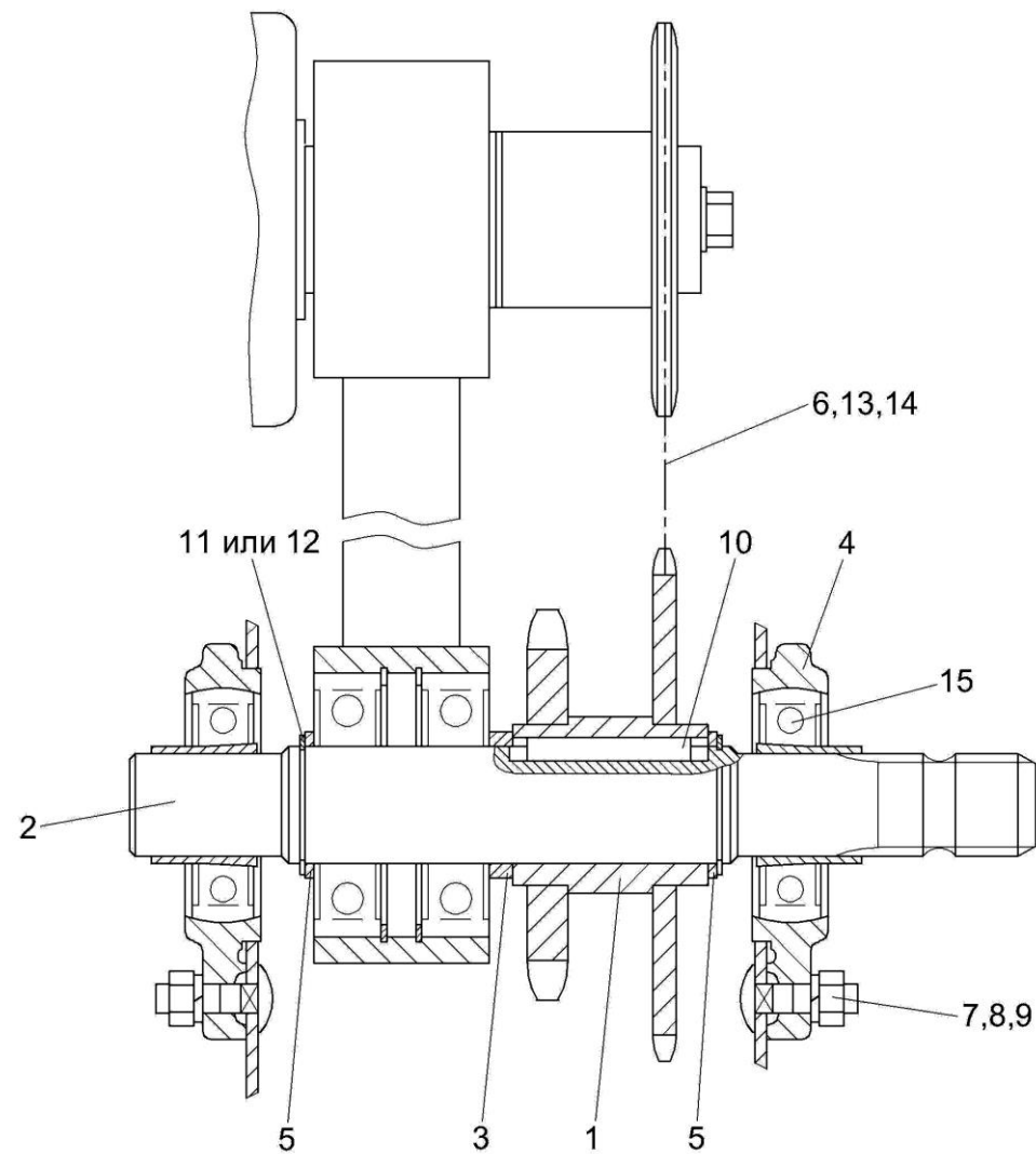
Рисунок 8 – Установка вала КЗК 1900601
