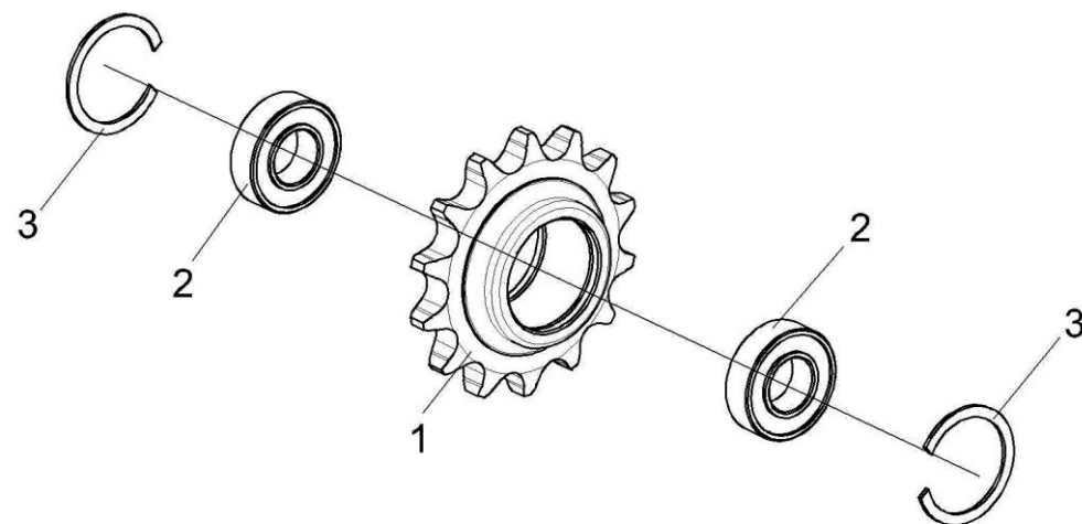
Рисунок 19 – Звездочка МКС 0514010
