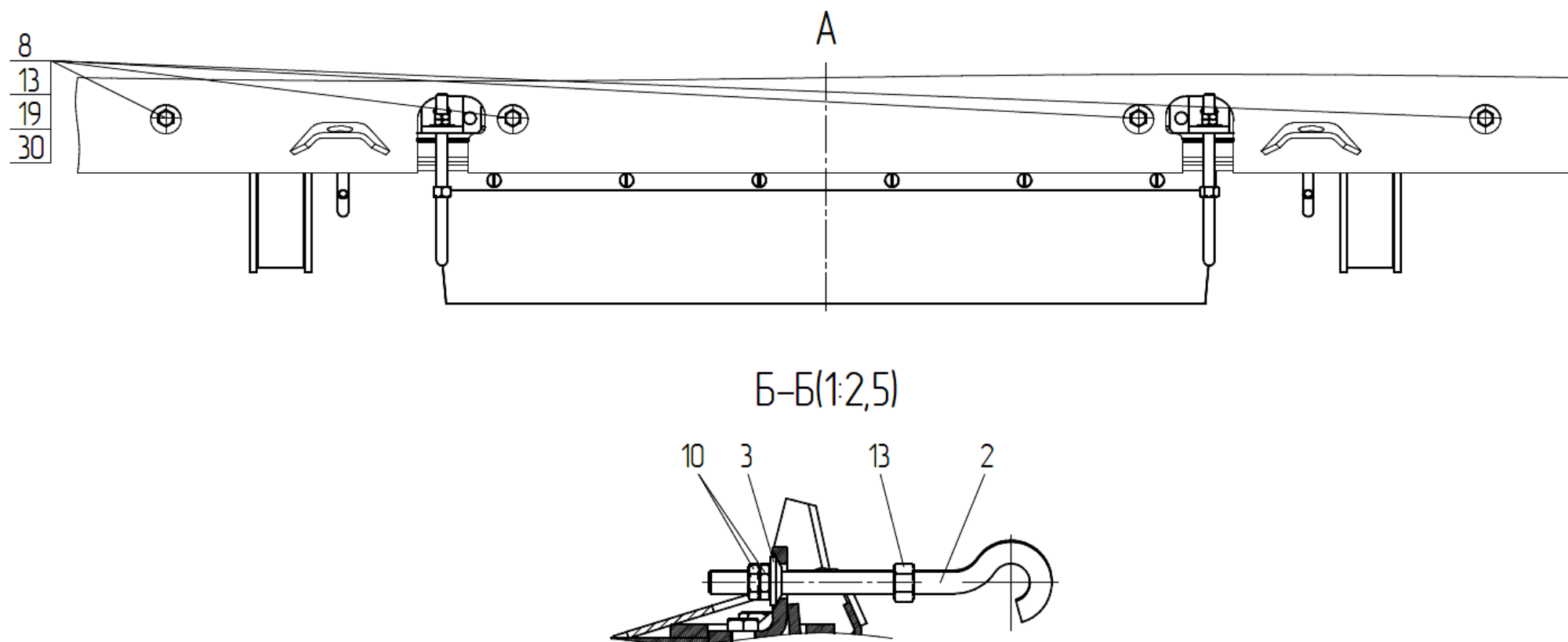
Рисунок 5б – Установка переходной рамки ПЗЗ 2201100А-01 (Лист 2)
