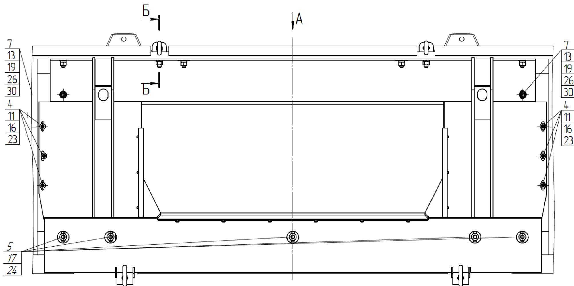
Рисунок 5б – Установка переходной рамки ПЗЗ 2201100А-01 (Лист 1)
