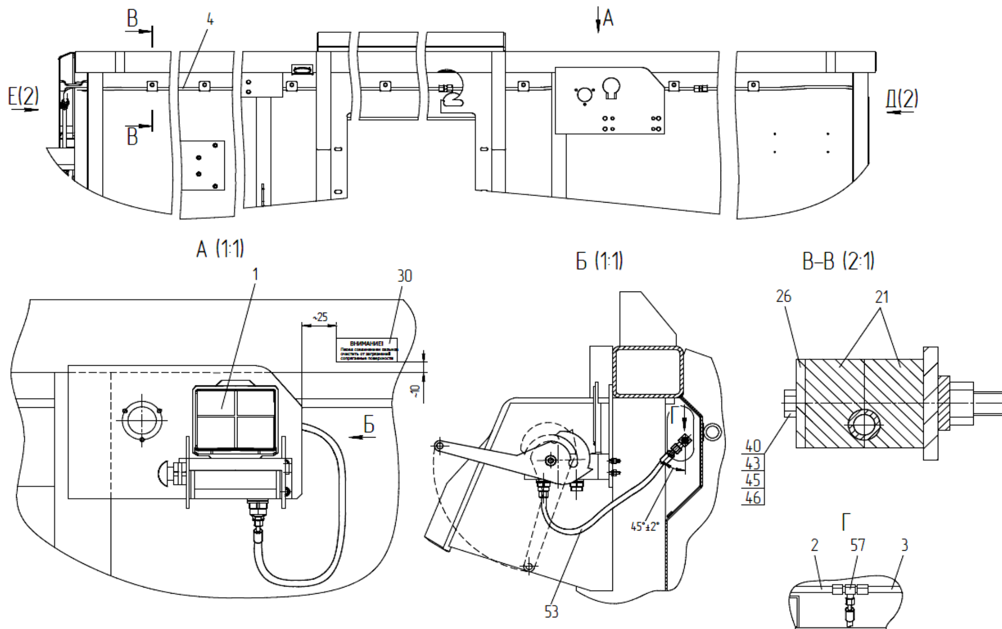
Рисунок 37 – Гидросистема подборщика ПЗЗ 2283000 (Лист 1)
