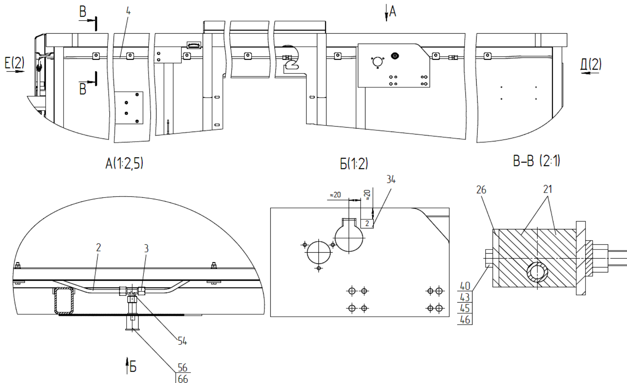
Рисунок 34 – Гидросистема подборщика ПЗЗ 2281000 (Лист 1)
