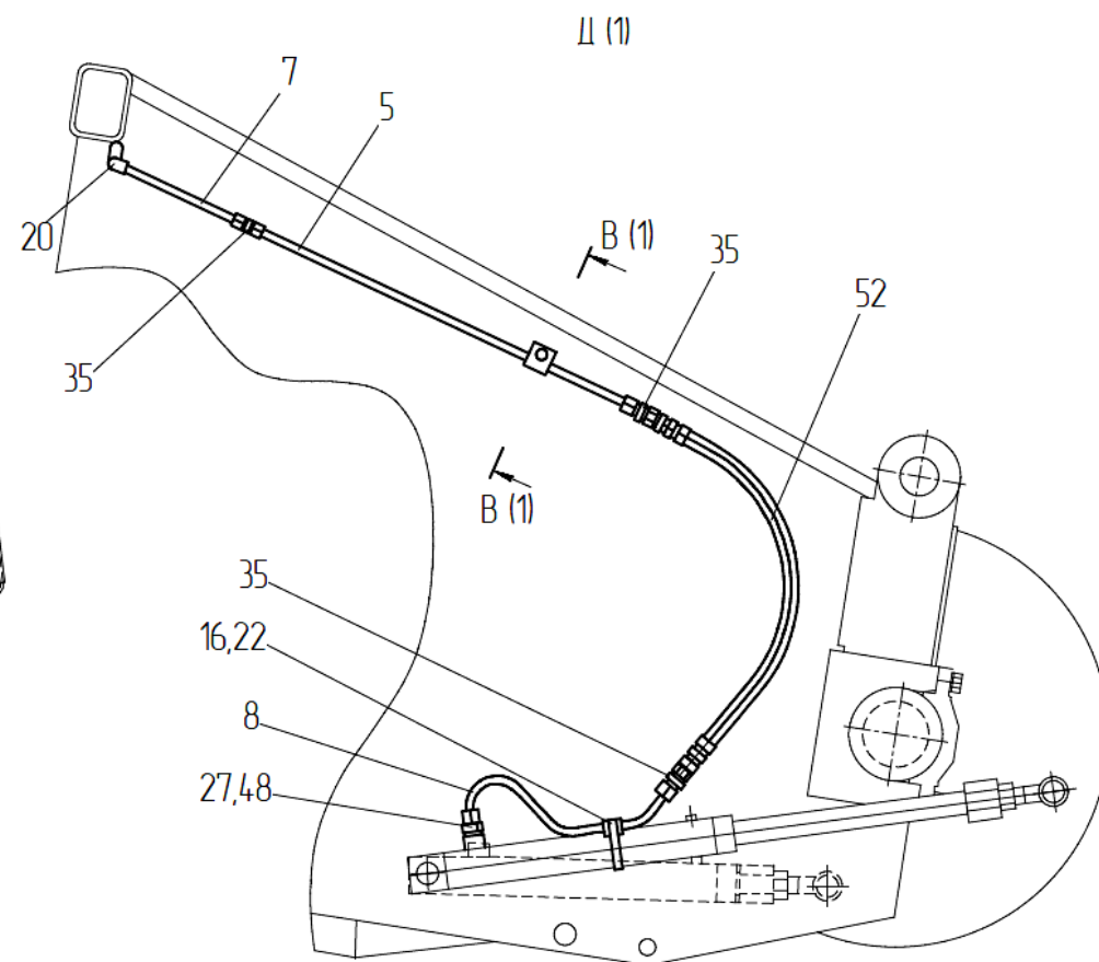
Рисунок 34 – Гидросистема подборщика ПЗЗ 2281000 (Лист 2)
