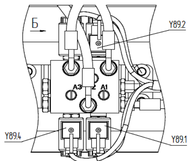
Рисунок 33 – Электрооборудование подборщика зернового ПЗЗ 2272000
