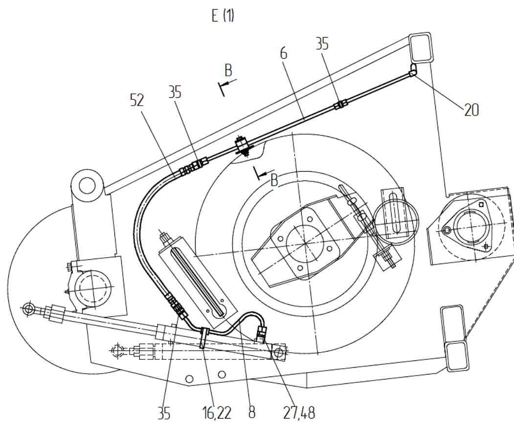
Рисунок 35 – Гидросистема подборщика ПЗЗ 2282000 (Лист 2)
