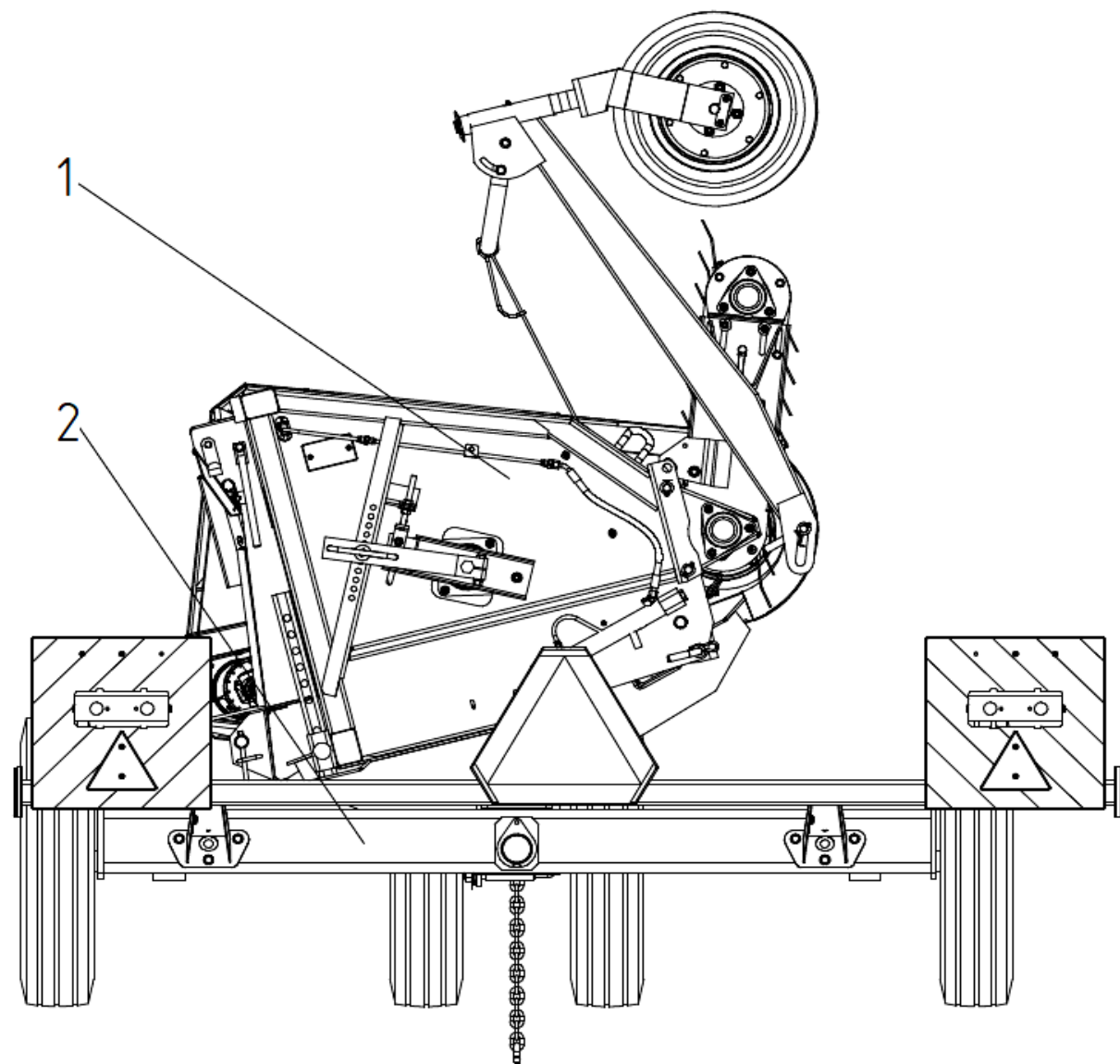
Рисунок 1 – Подборщик зерновой ПЗ-4,4-8 (ПЗЗ 2200000/-01/-02/-03/-04/-05/-06/-07/-08/-09/-10/-11)
