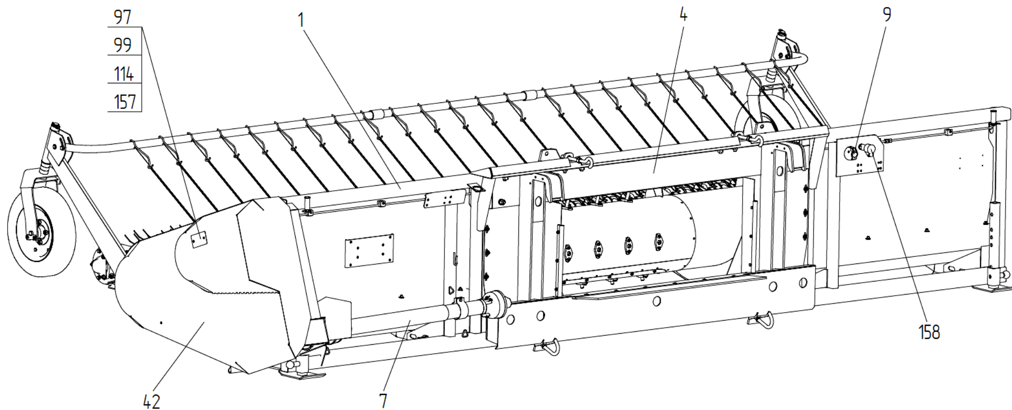
Рисунок 2а – Подборщик зерновой ПЗ-4,4-8 (ПЗЗ 2200000/-01/-02/-03/-04/-05/-06/-07/-08/-09/-10/-11)
