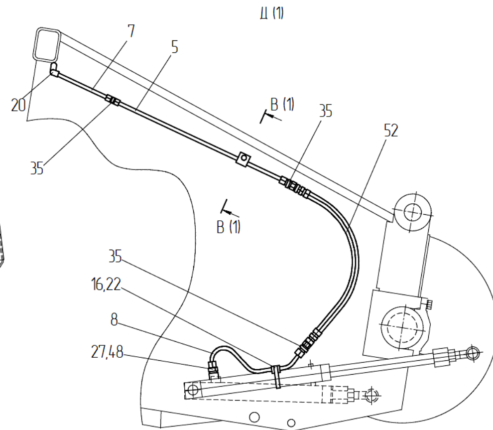
Рисунок 35 – Гидросистема подборщика ПЗЗ 2282000 (Лист 2)
