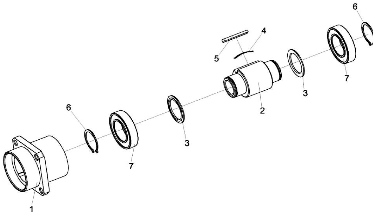
Рисунок 27 – Муфта обгонная КЗР 1928010
