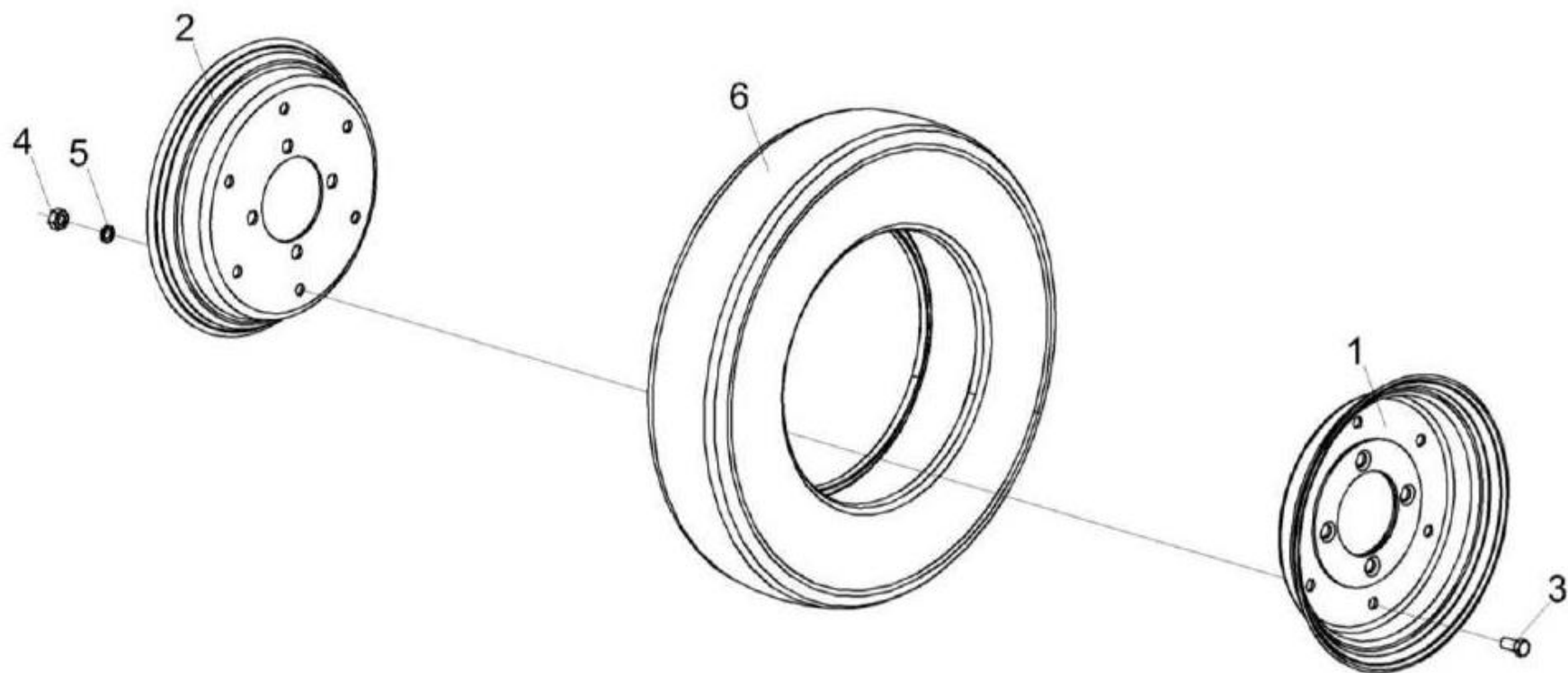
Рисунок 31 – Колесо 1925050
