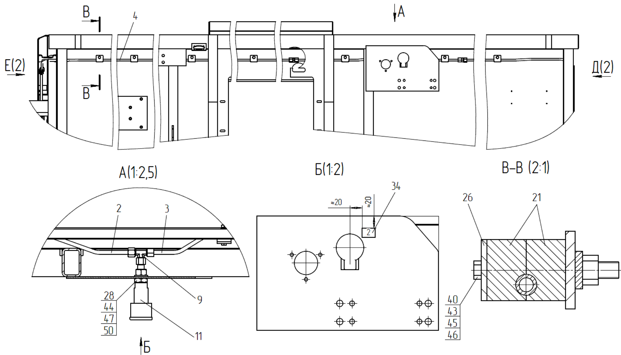
Рисунок 35 – Гидросистема подборщика ПЗЗ 2282000 (Лист 1)
