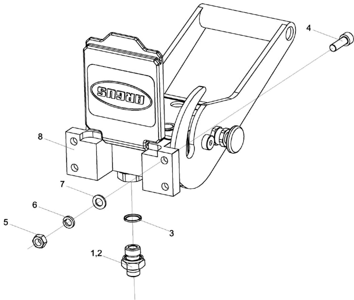
Рисунок 40 – Разъем гидравлический многофункциональный КЗК-12А-1-0689390
