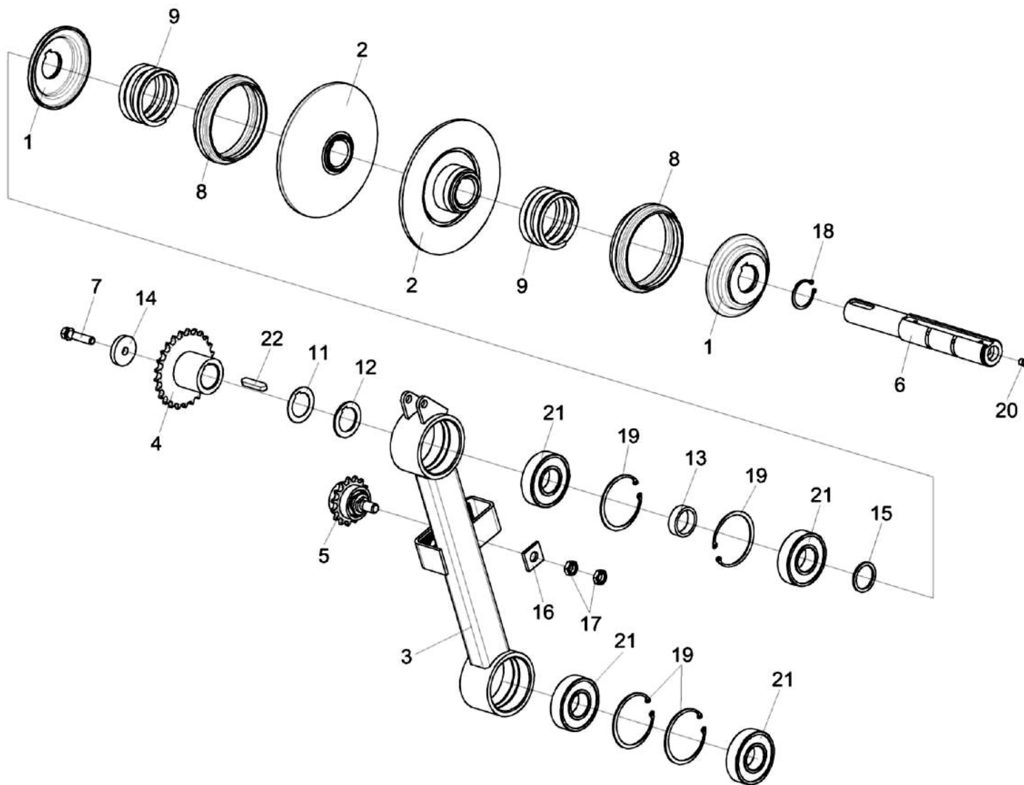
Рисунок 17 – Вариатор КЗР 1914000-01
