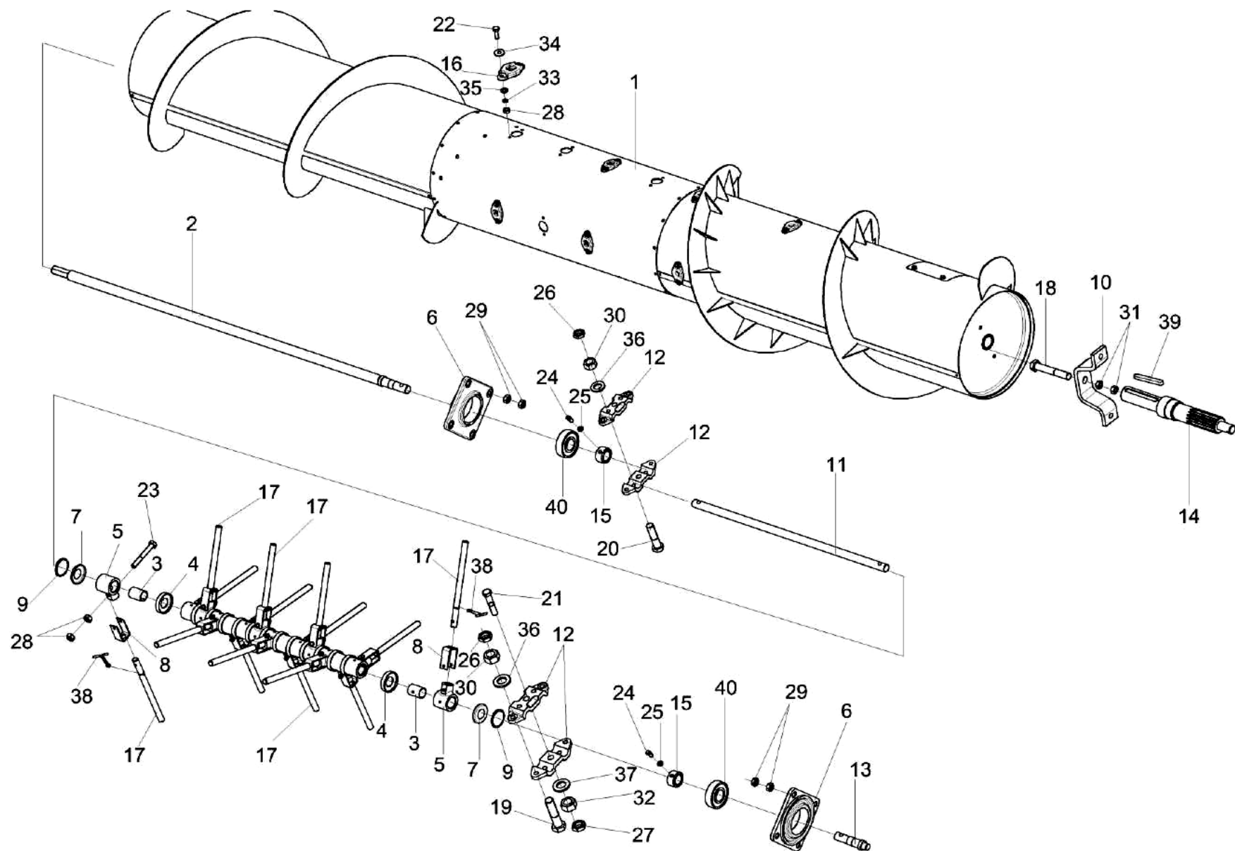
Рисунок 10 – Шнек ПЗЗ 1502000
