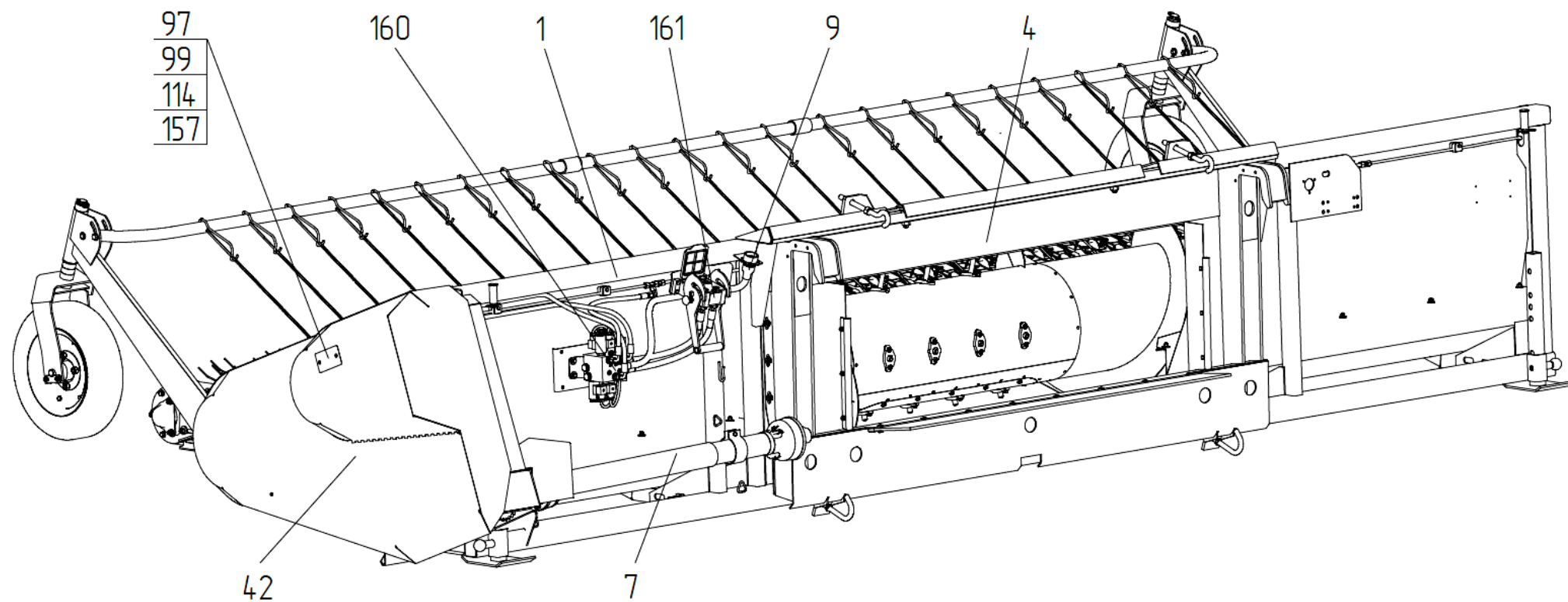
Рисунок 2г – Подборщик зерновой ПЗ-4,4-8 (ПЗЗ 2200000/-01/-02/-03/-04/-05/-06/-07/-08/-09/-10/-11)
