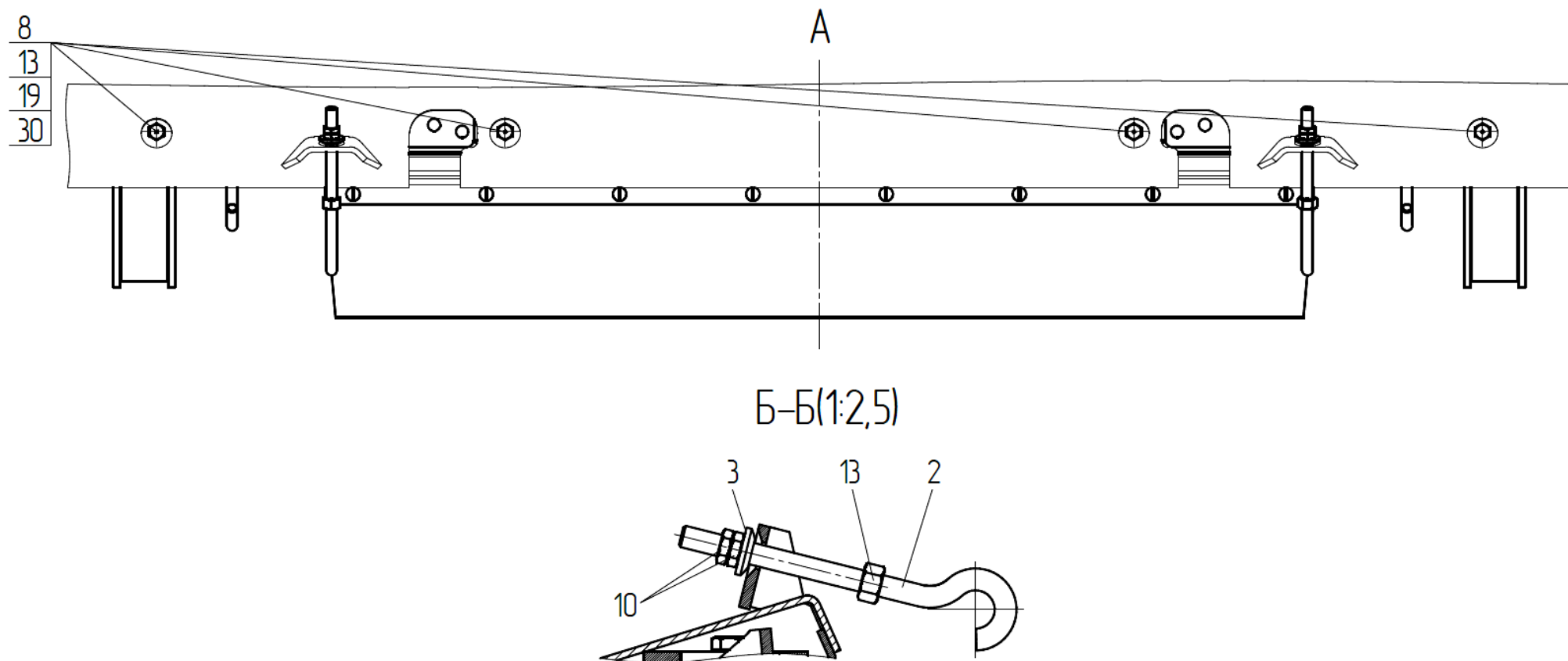
Рисунок 5а – Установка переходной рамки ПЗЗ 2201100А (Лист 2)
