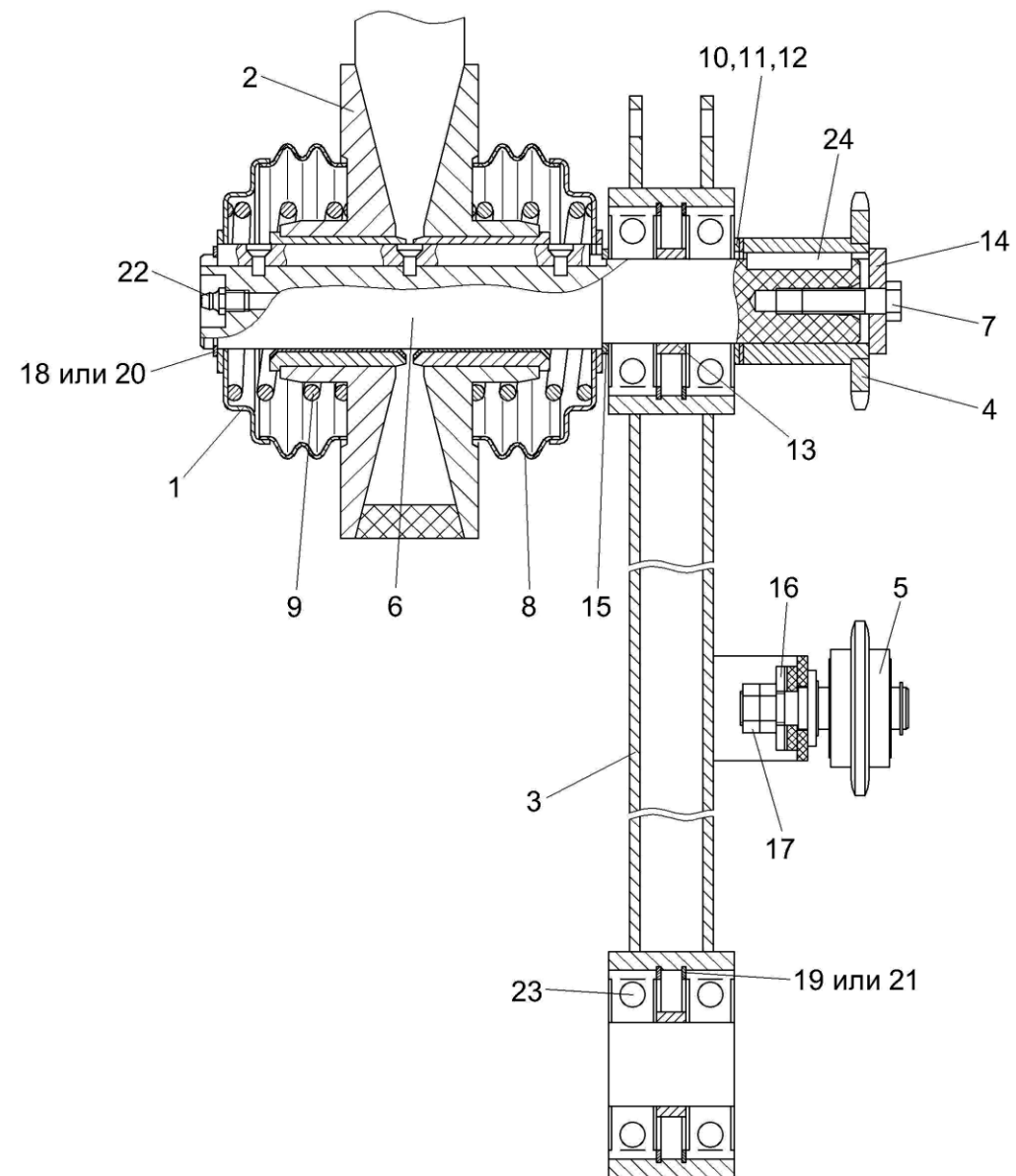
Рисунок 16 – Вариатор ПЗЗ 2014000-01
