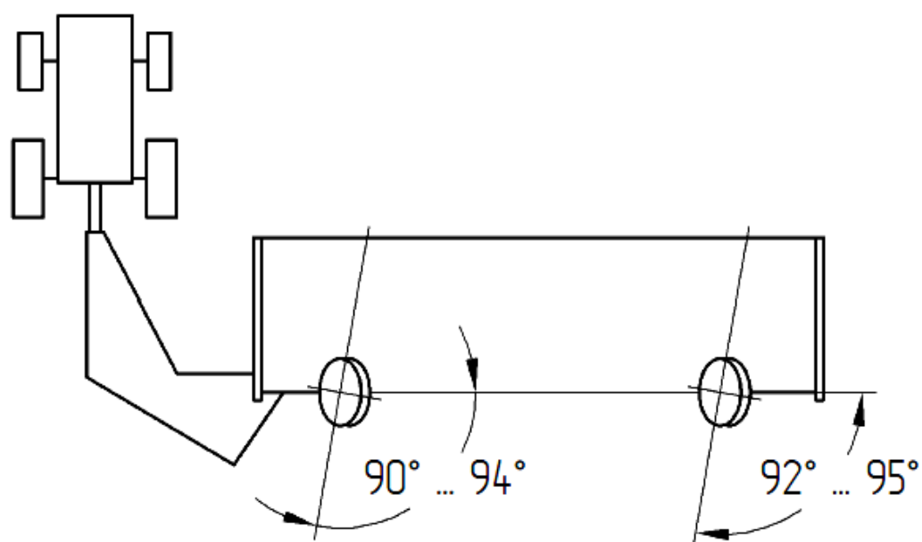
Рисунок 2.12 – Расположение колес (схождение)
