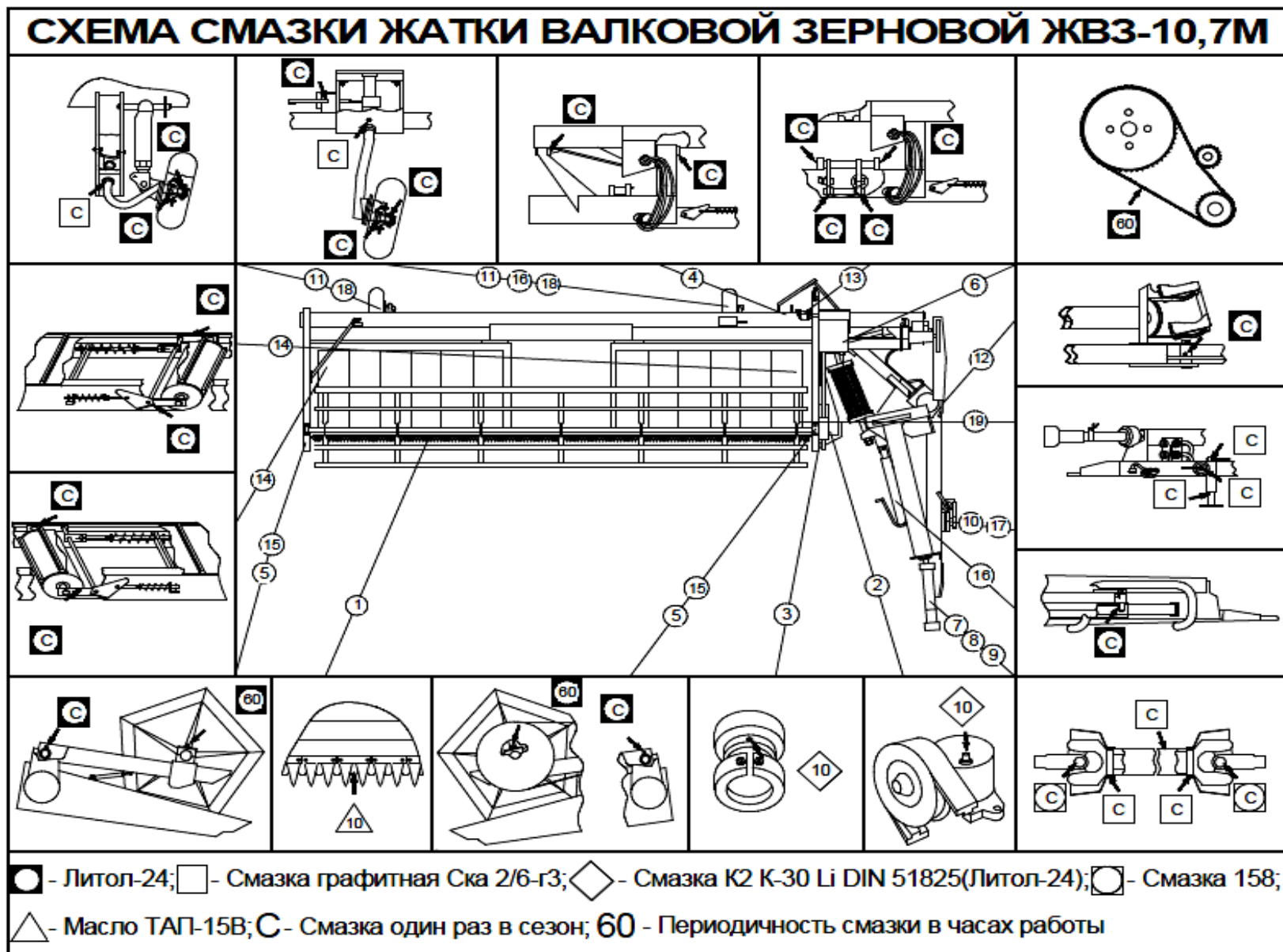
Рисунок 4.1 – Схема смазки жатки валковой зерновой ЖВЗ-10,7М
