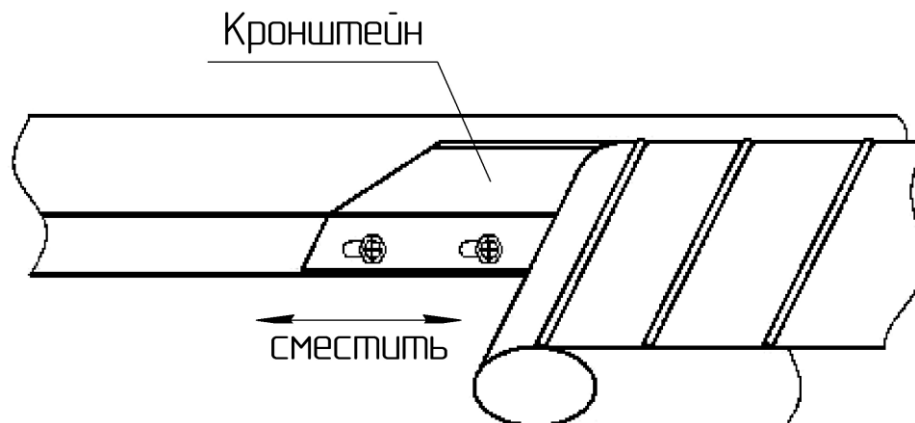
Рисунок 2.6 – Устранение перекося и сползания лент
