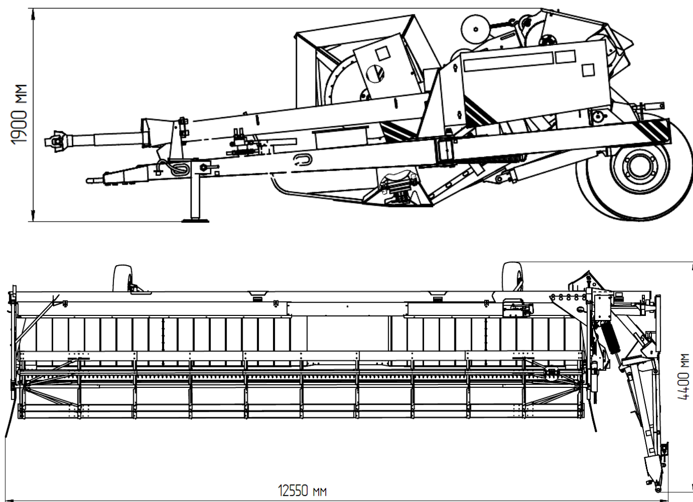
Рисунок 1.1а – Габаритные размеры жатки ЖВЗ-10,7М
