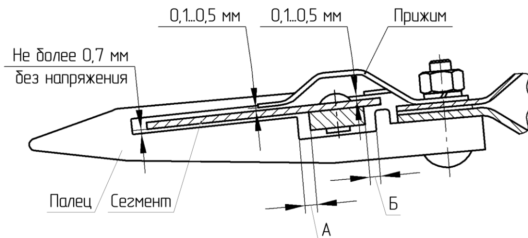
Зазоры А и Б не менее 1 мм на первом пальце в любом положении тяги привода Рисунок 2.9 – Регулировка режущего аппарата
