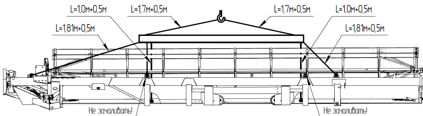
Рисунок 10.1 – Строповка жатки
