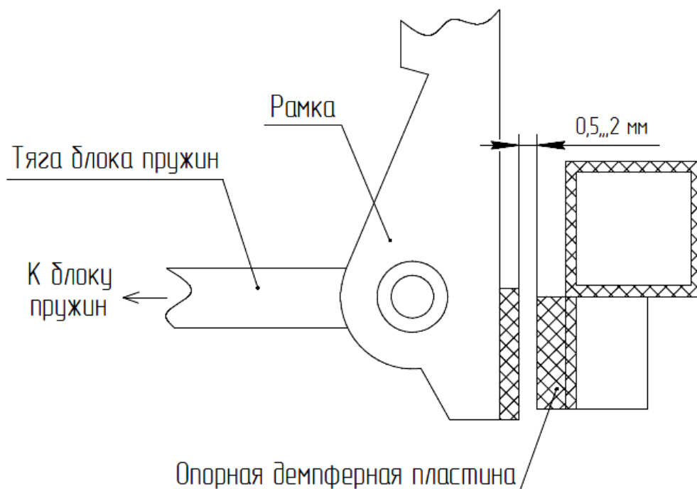
Рисунок 2.13 – Регулировка механизма копирования
