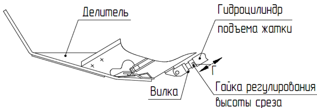
Рисунок 2.3 – Установка левого делителя и регулировка высоты среза
