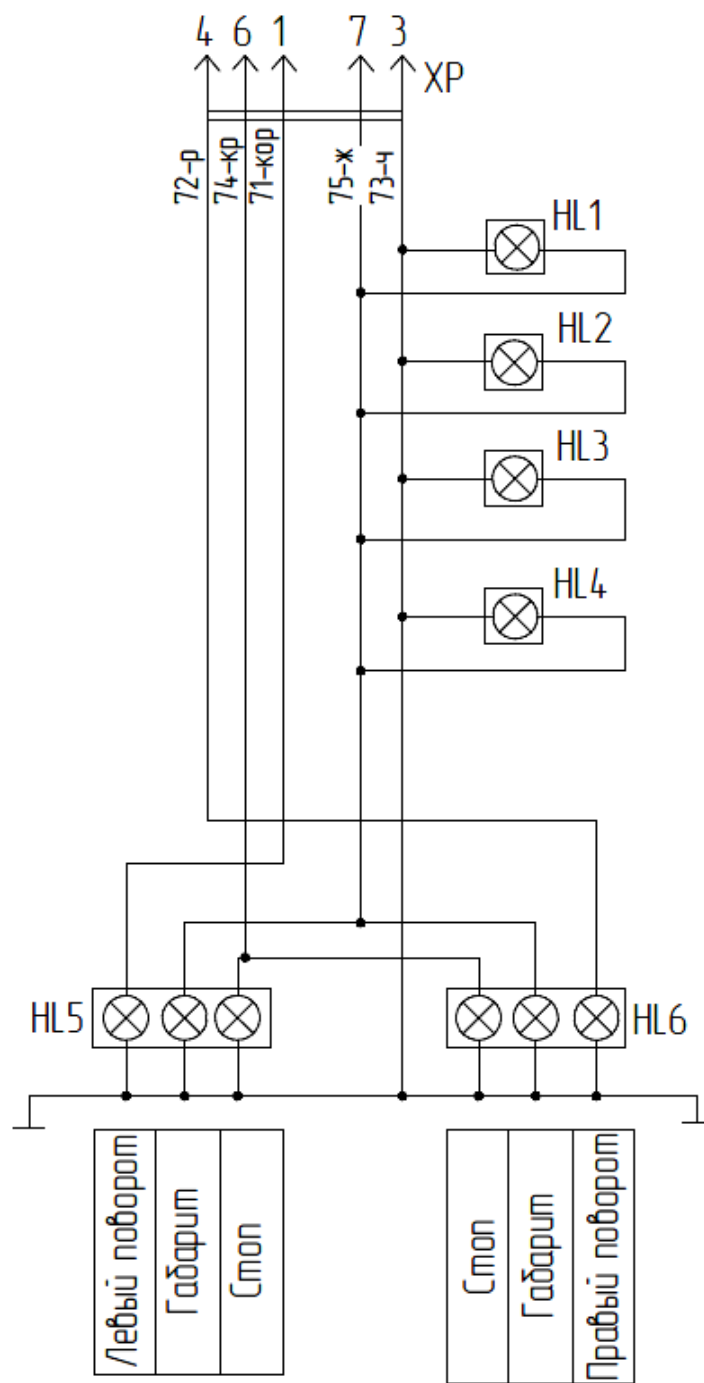
Рисунок 1.4 – Схема электрическая принципиальная
