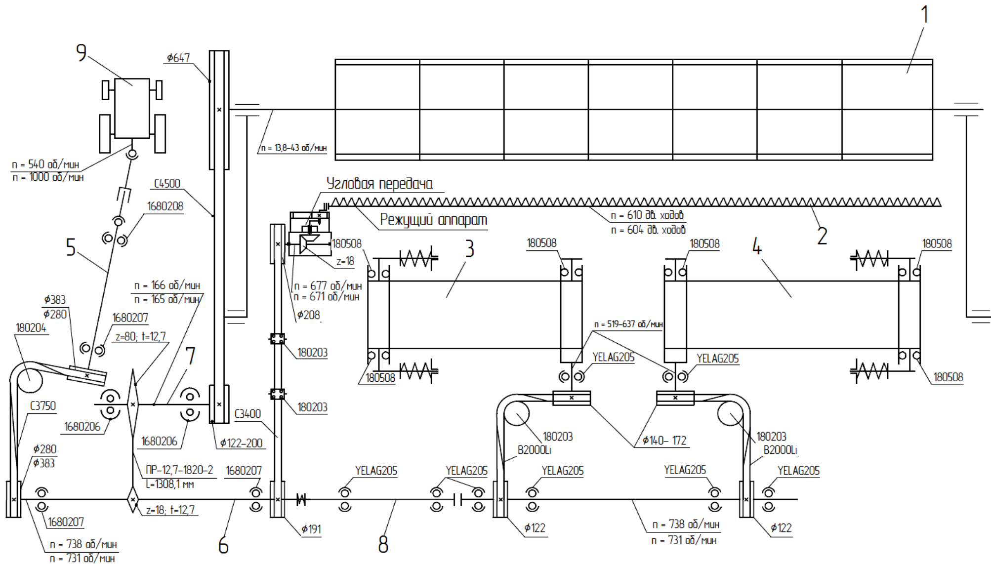
1 – мотовило; 2 – режущий аппарат; 3 – транспортер левый; 4 – транспортер правый; 5 – вал снщи; 6 – промежуточный вал рамы навески; 7 – промежуточный вал привода мотовила; 8 – промежуточный вал привода транспортеров; 9 – трактор.
