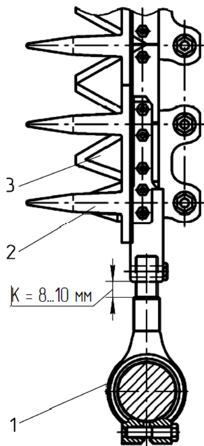
1 – головка ножа; 2 – палец направляющий; 3 – сегмент Рисунок 2.8 – Режущий аппарат
