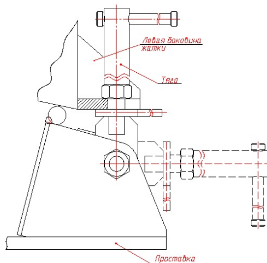
Рисунок 5. Фиксация жатки тягой.
