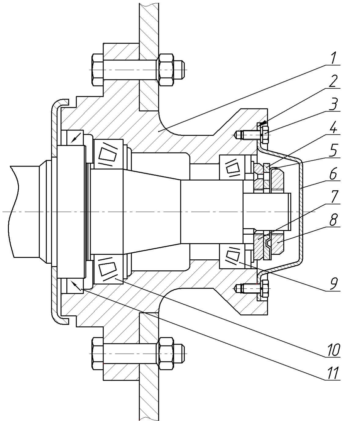
1-ступица; 2-прокладка; 3-болт; 4-шайба замковая; 5-шайба замочная; 6-крышка; 7-гайка-шайба; 8-гайка; 9-подшипник 7509 ТУ 37.006.162-89; 10-подшипник 7512 ТУ 37.006.162-89; 11-манжета 2.2-110x135-1ГОСТ 8752-79.
