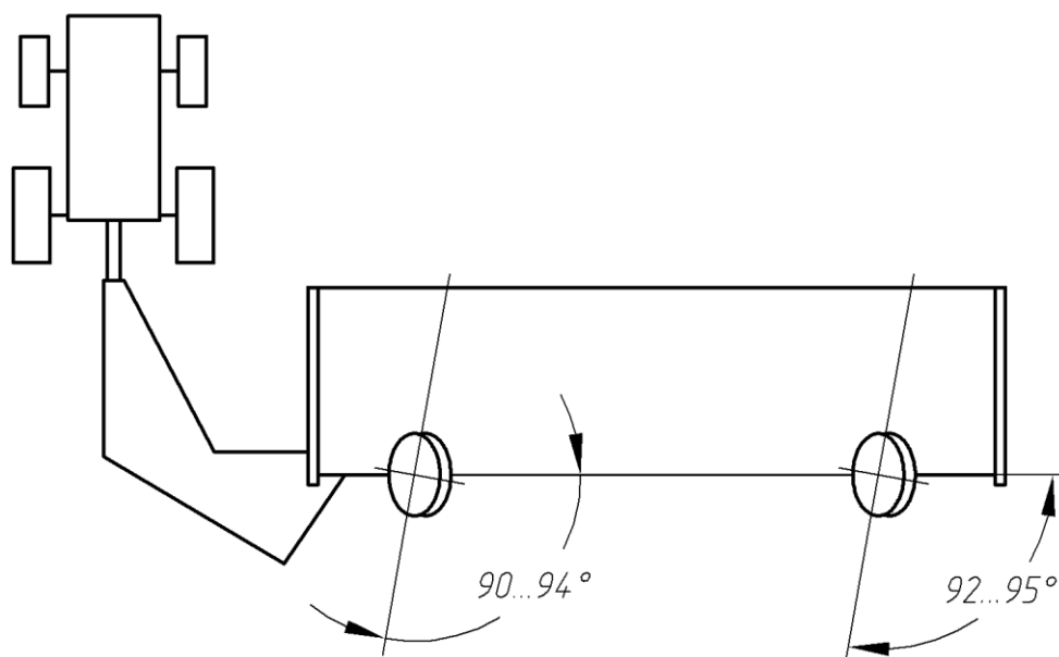
Рисунок 18. Расположение колёс (схождение).
