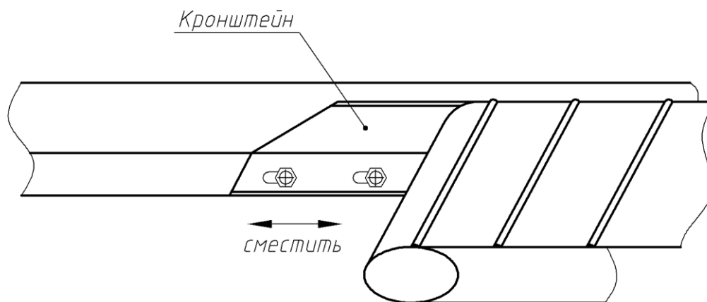
Рисунок 12. Устранение перекоса и сползания лент.
