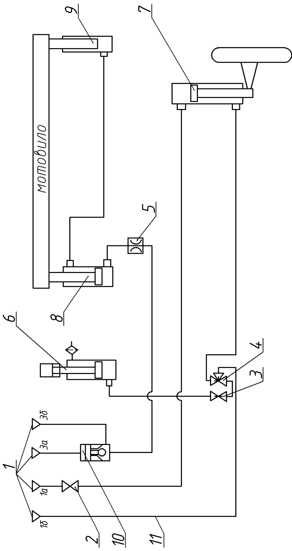
1-полушфты наружные ПН (МС 12-3-120); 2,3-клапан запорный FT221/1-14 (клапан 2 запирает гидроцилиндр 7 при переводе жатки в транспортное положение, клапан 3 запирает гидроцилиндр 6 подъема жатки); 4-клапан распределительный FT221/3-14 (клапан 4 распределяет давление жидкости на гидроцилиндры 7 или 6); 5-дроссель (дроссель 5 обеспечивает срабатывание гидроцилиндров 8 и 9); 6-гидроцилиндр подъема жатки КГЦ 228.80.40-4.00; 7-гидроцилиндр поворота колеса КГЦ 227.50.32-250; 8,9-гидроцилиндры подъема мотобила КГЦ 214.00.000 и КГЦ 215.00.000; 10-гидрозамок КОНУ 1/4-S (гидрозамок 10 запирает гидроцилиндры 8 и 9); 11-рукава высокого давления или трубопроводы.
