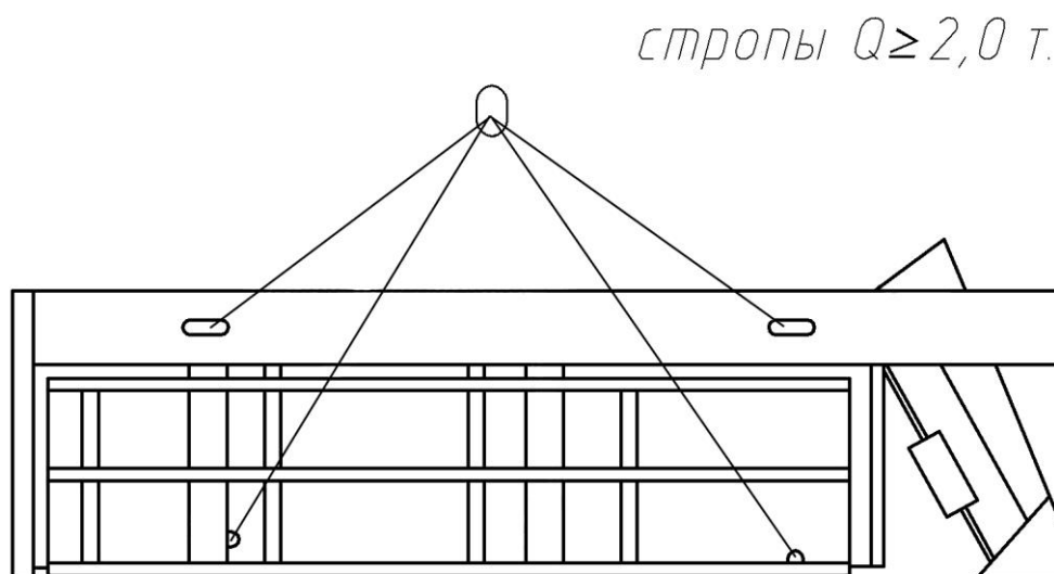
Рисунок 6. Схема строповки жатки ЖВЗ-5 (ЖВЗ-6)
