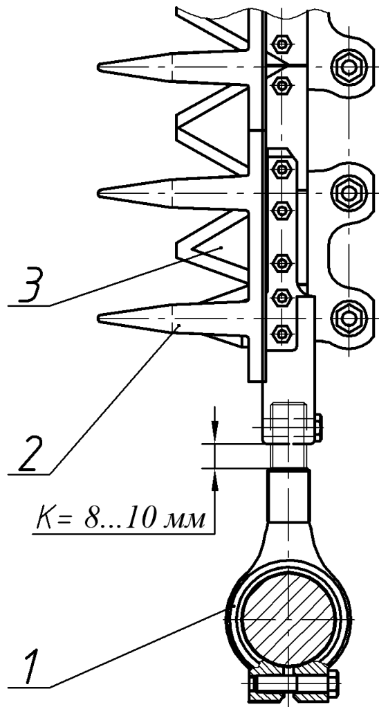
1-головка ножа; 2-палец направляющий; 3-сегмент.
