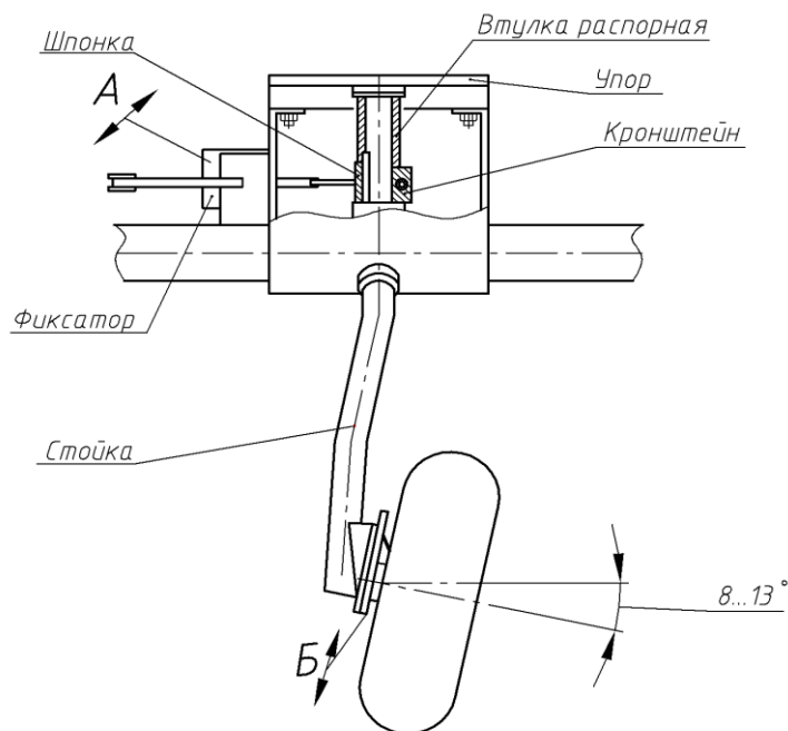
Рисунок 7. Установка левого колеса.
