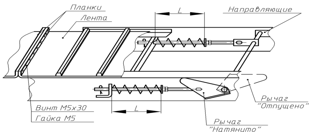
Рисунок 11. Установка и натяжка транспортной ленты
