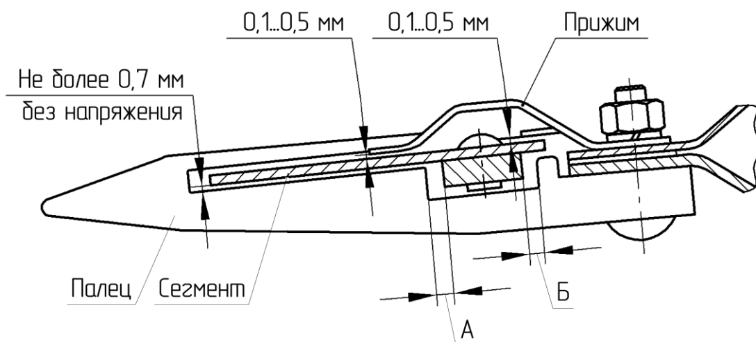
Зазоры А и Б не менее 1 мм на первом пальце в любом положении тяги привода Рисунок 2.10 – Регулировка режущего аппарата
