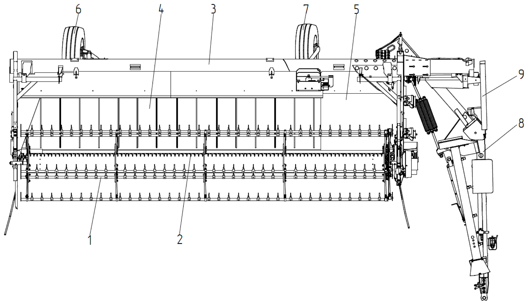
1 – мотовило; 2 – режущий аппарат; 3 – рама жатки; 4 – транспортер; 5 – выгрузное окно; 6, 7 – левое и правое колесо; 8 – сница; 9 – рама навески (проставка).
