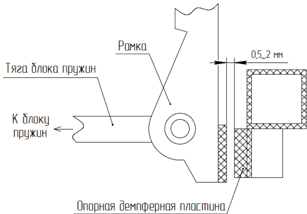
Рисунок 2.15 – Регулировка механизма копирования
