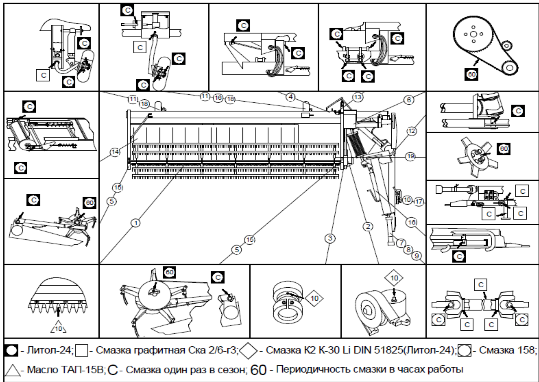
Рисунок 4.1 – Схема смазки жатки валковой зерновой ЖВЗ-6,0П
