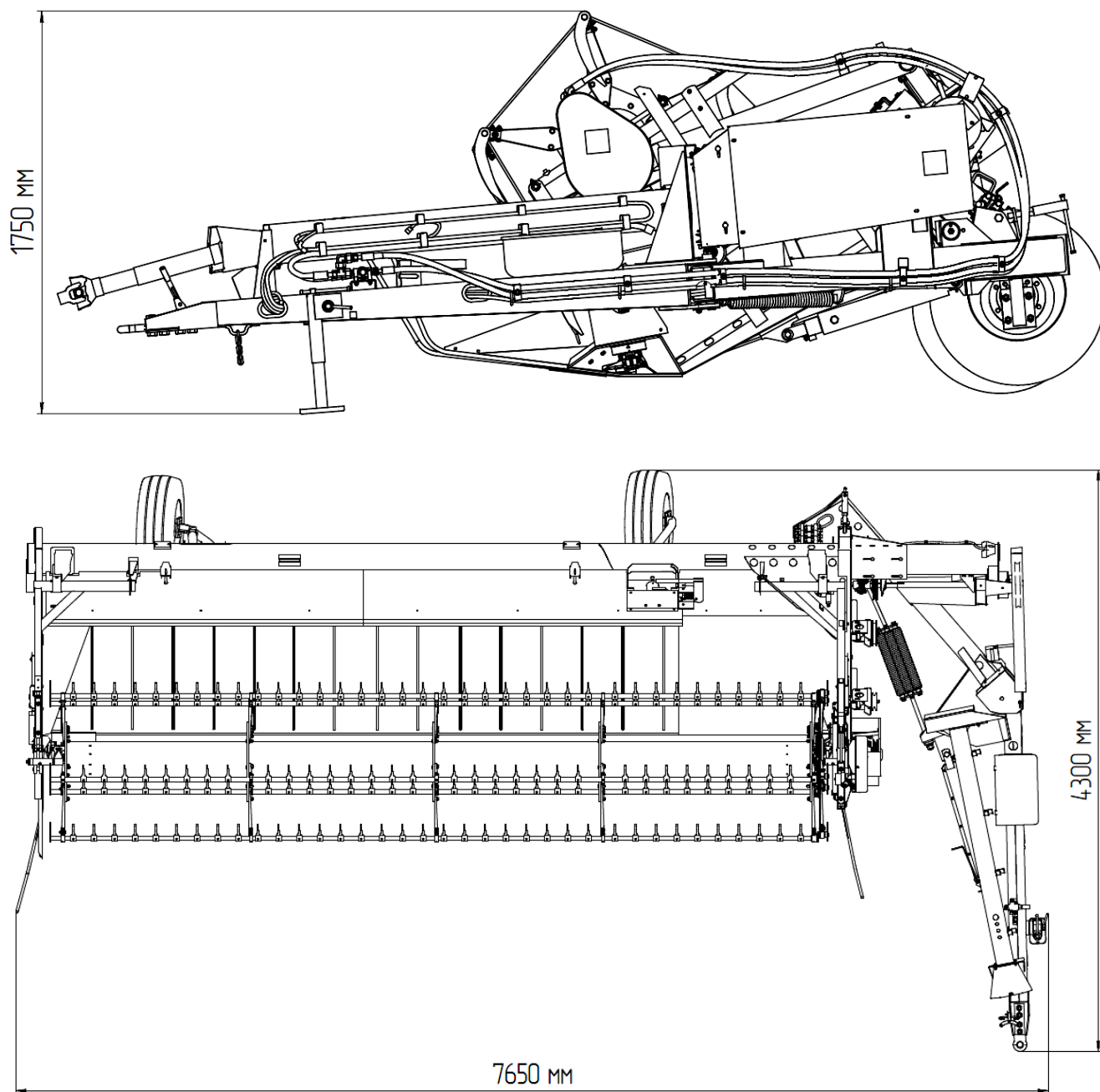
Рисунок 1.1а – Габаритные размеры жатки ЖВЗ-6,0П
