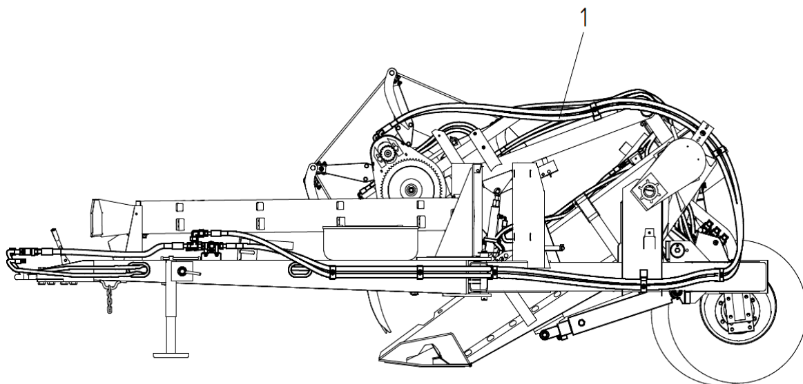
1 – гидросистема жатки
