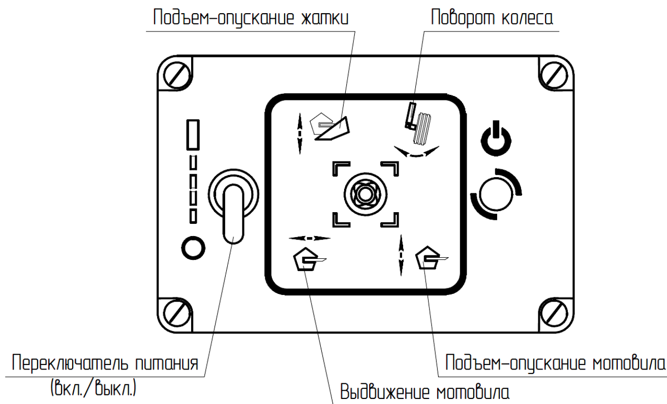
Рисунок 1.8 – Пульт управления жаткой
