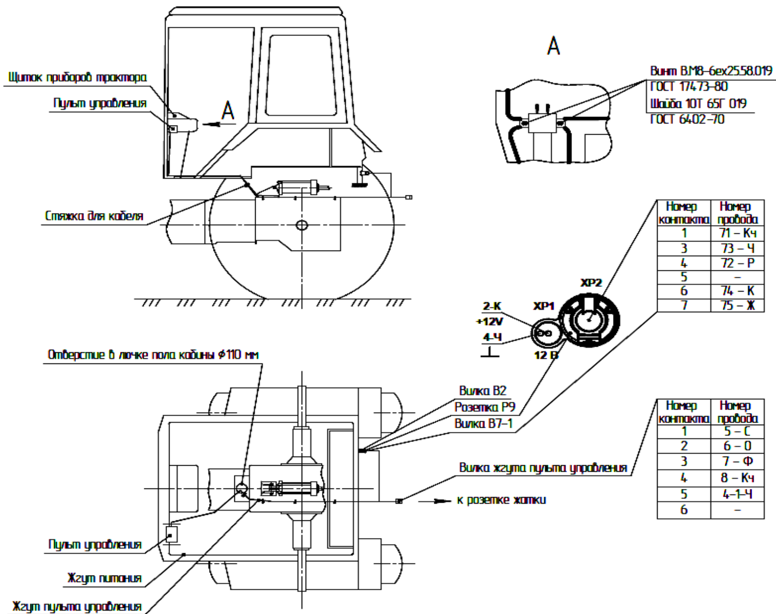
Рисунок 1.6 – Схема подключения электрооборудования жатки в кабине трактора
