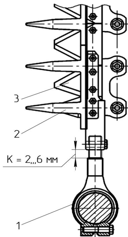
1 – головка ножа; 2 – палец направляющий; 3 – сегмент Рисунок 2.9 – Режущий аппарат
