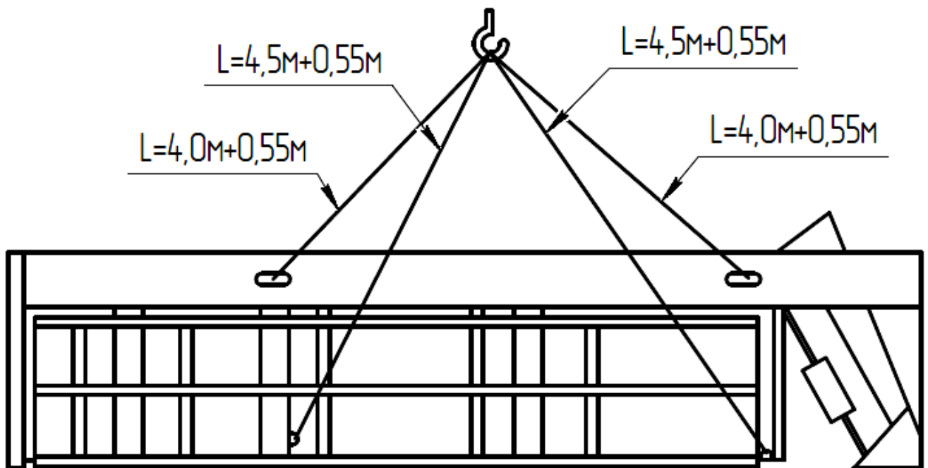
Стропы не должны касаться мотовила Рисунок 2.1 – Схема строповки жатки ЖВЗ-6,0П
