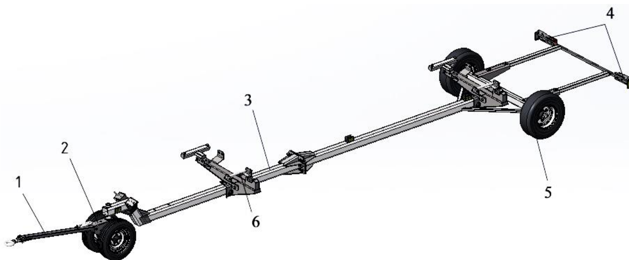
1 – дышло; 2 – ось передняя; 3 – рама тележки; 4 – балка габаритная; 5 – колесо; 6 – фиксатор
