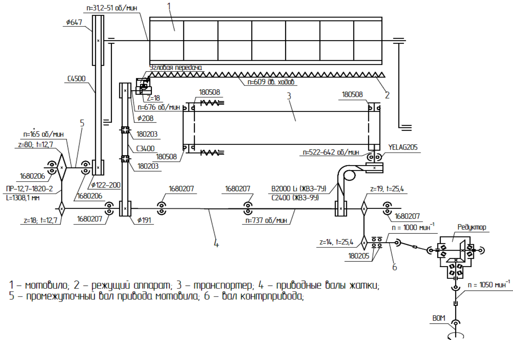
Рисунок 1.2 – Кинематическая схема жатки ЖВЗ-7У(ЖВЗ-9У)
