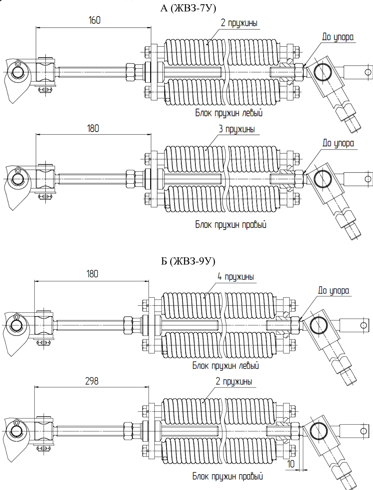
Рисунок 15 – Регулировка блока пружин на ЖВЗ-7У(А), ЖВЗ-9У(Б)
