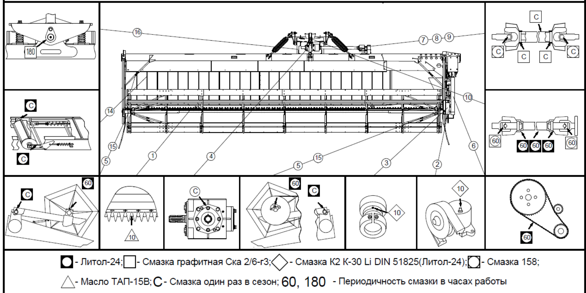
Рисунок 3.1 – Схема смазки жатки валковой ЖВЗ-6УМ
