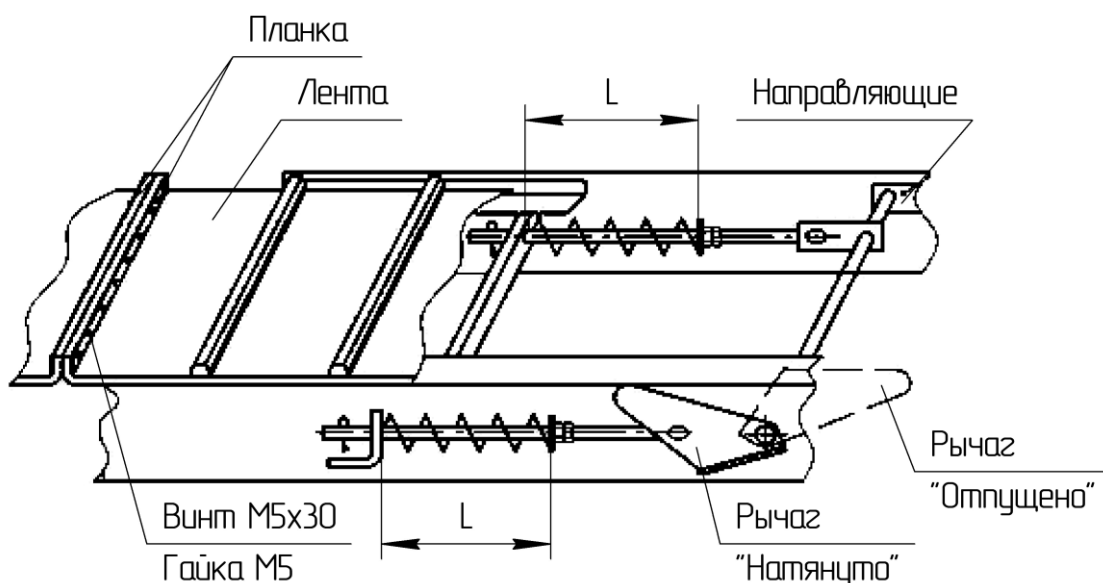
Рисунок 2.6 – Установка и натяжка транспортерной ленты
