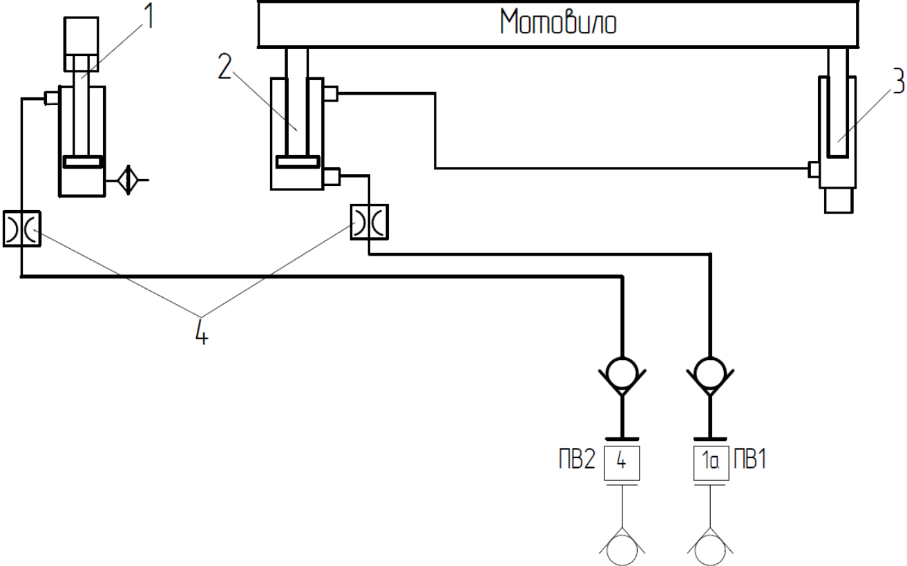
Рисунок 1.4 – Гидравлическая схема жатки
