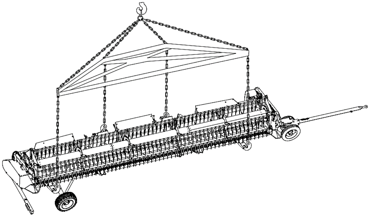
Рисунок 6.1 – Схема строповки жатки с транспортной тележкой
