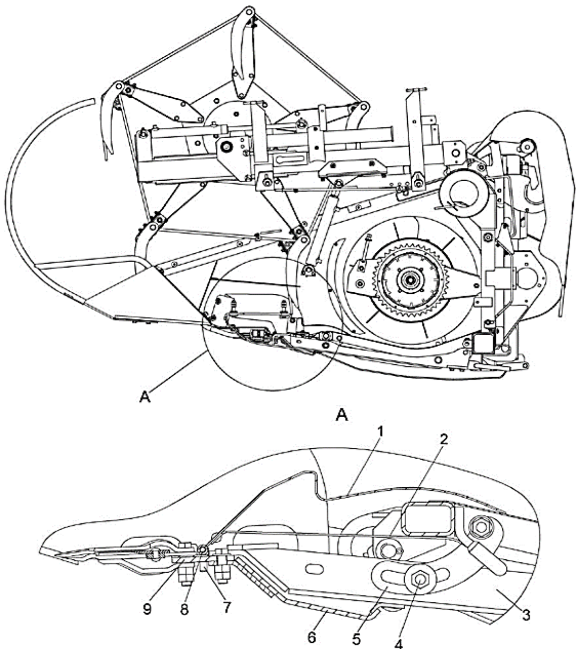
1 – щиток; 2 – рессора; 3 – рычаг; 4 – гайка; 5 – ограничитель хода; 6 – ползья; 7 – винт; 8 – ось; 9 – брус режущего аппарата Рисунок 1.4 – Жатка для сои (вид сбоку)
