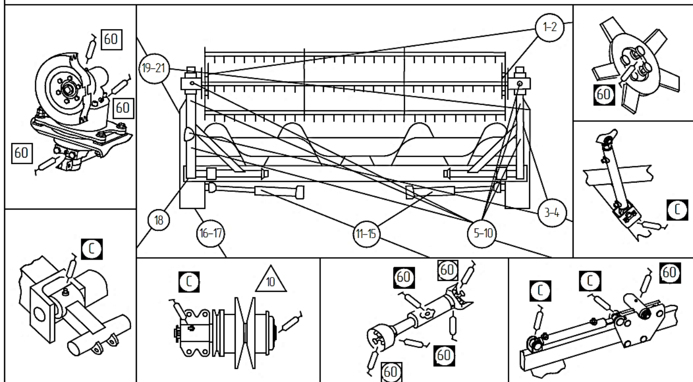
Рисунок 3.1 – Схема смазки жатки
