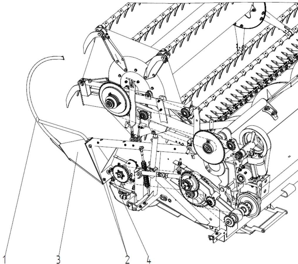
1 – прутковый делитель; 2 – болт DIN M12x20; 3 – носок; 4 – болт M12x25 Рисунок 2.1 – Жатка
