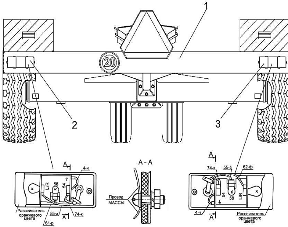
1 – балка габаритна; 2, 3 – фонари Условные обозначения цветов проводов: З – зеленый; К – красный; Р – розовый; Ф – фиолетовый; Ч – черный Рисунок 2.2 – Установка электрооборудования на транспортную тележку
