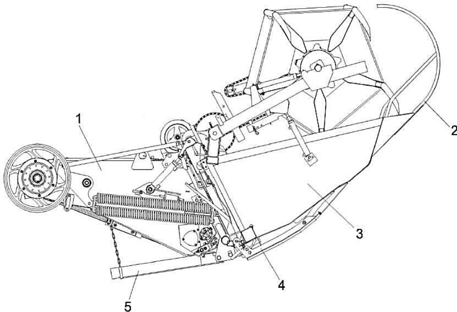
1 – камера наклонная; 2 – делитель прутковый; 3 – жатка; 4 – башмак; 5 – упор Рисунок 2.3 – Жатка, навешенная на наклонную камеру
