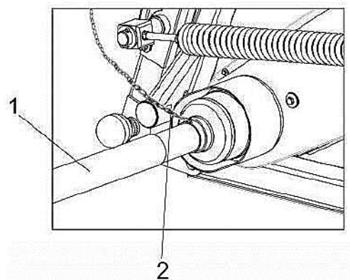
1 – вал карданный; 2 – цепочка Рисунок 2.8 – Подсоединение карданного вала
