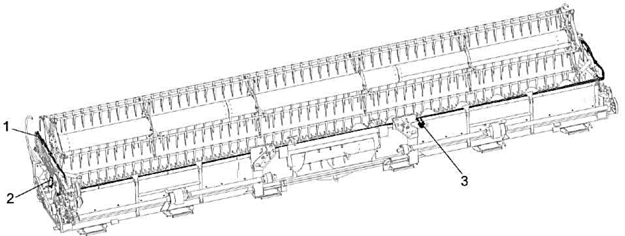
Рисунок 1.6 – Жатка для сои (вид справа)
