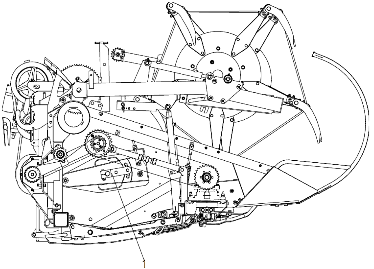
Рисунок 1.6 – Жатка для сои (вид справа)
