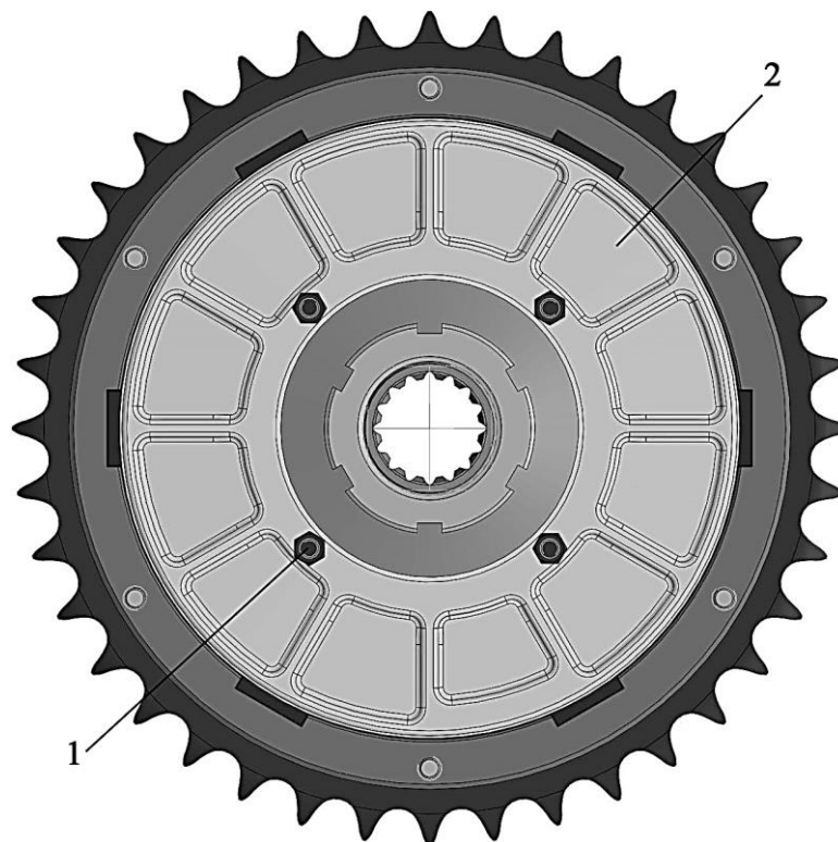
Рисунок 2.22 – Муфта предохранительная КГС 0202100-02
